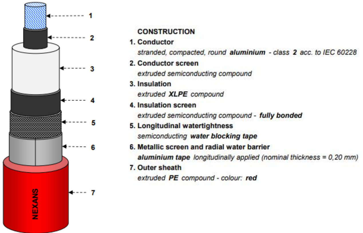
Figura 5 Configurazione tipica dei cavi unipolari previsti
