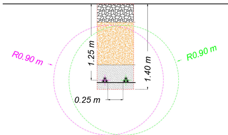
Figura 10 Fascia rispetto - 2 terne AT (interno parco)
