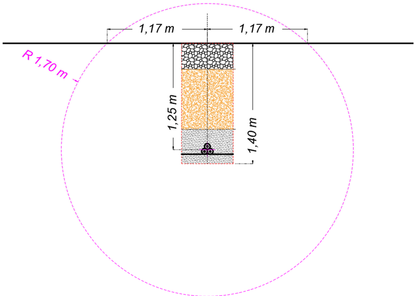
Figura 13 Fascia rispetto - terna AT (esterno parco)
