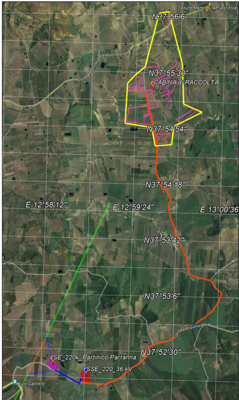
Figura 1 Ortofoto con impianto PV in progetto e collegamento alla RTN
