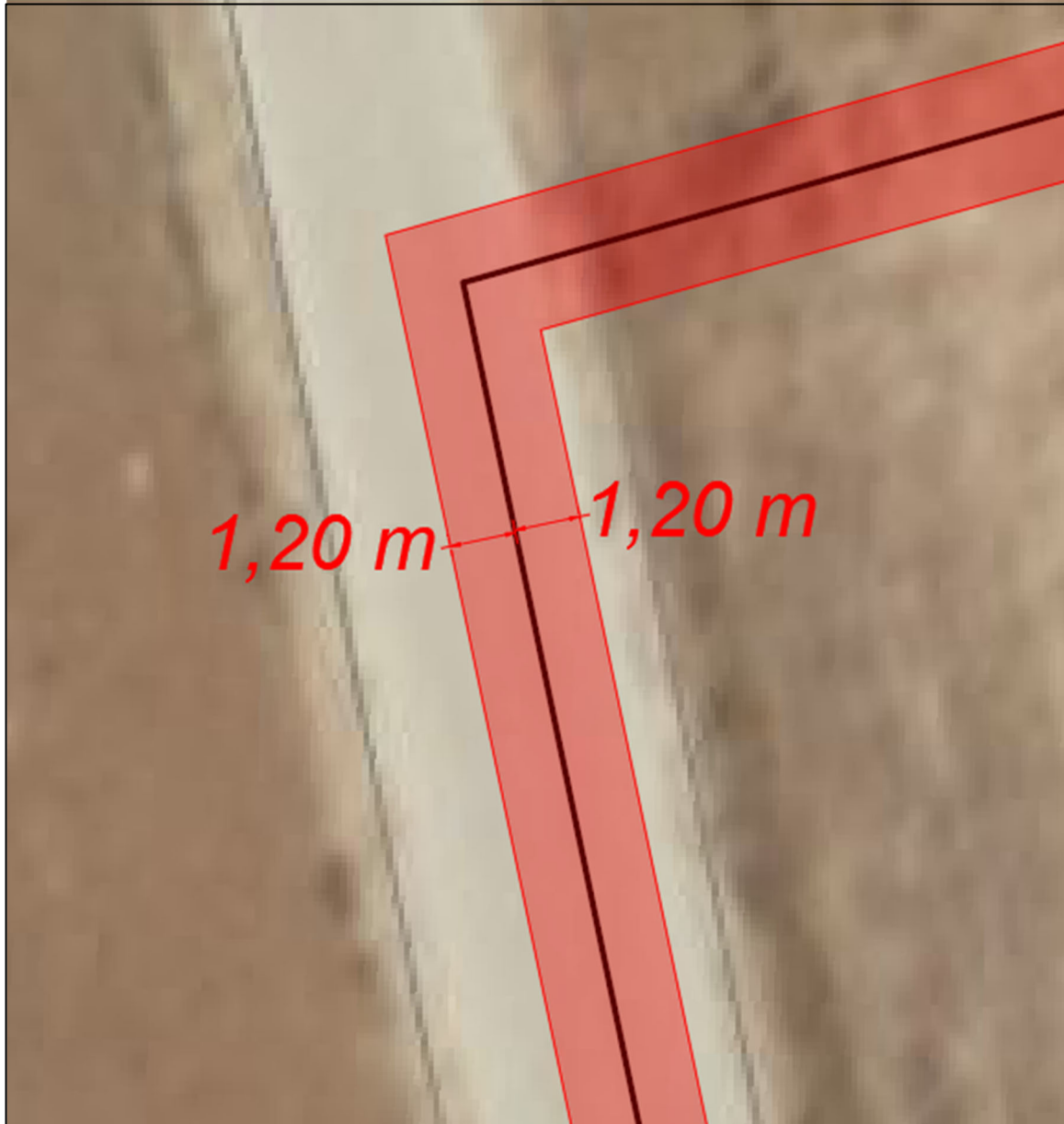
Figura 15 Esempio di buffer EM - lungo sede stradale
