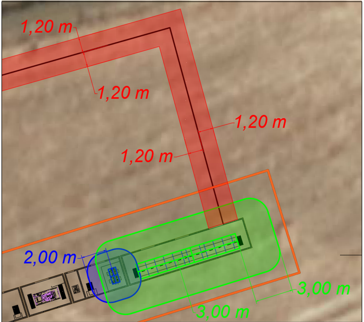
Figura 14 Esempio di buffer EM – CR
