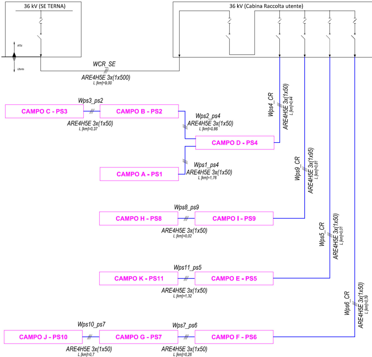
Figura 2 Schema a blocchi impianto PV con cavi in progetto
