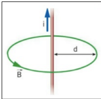
Figura 5 Campo magnetico generato da filo percorso da corrente
