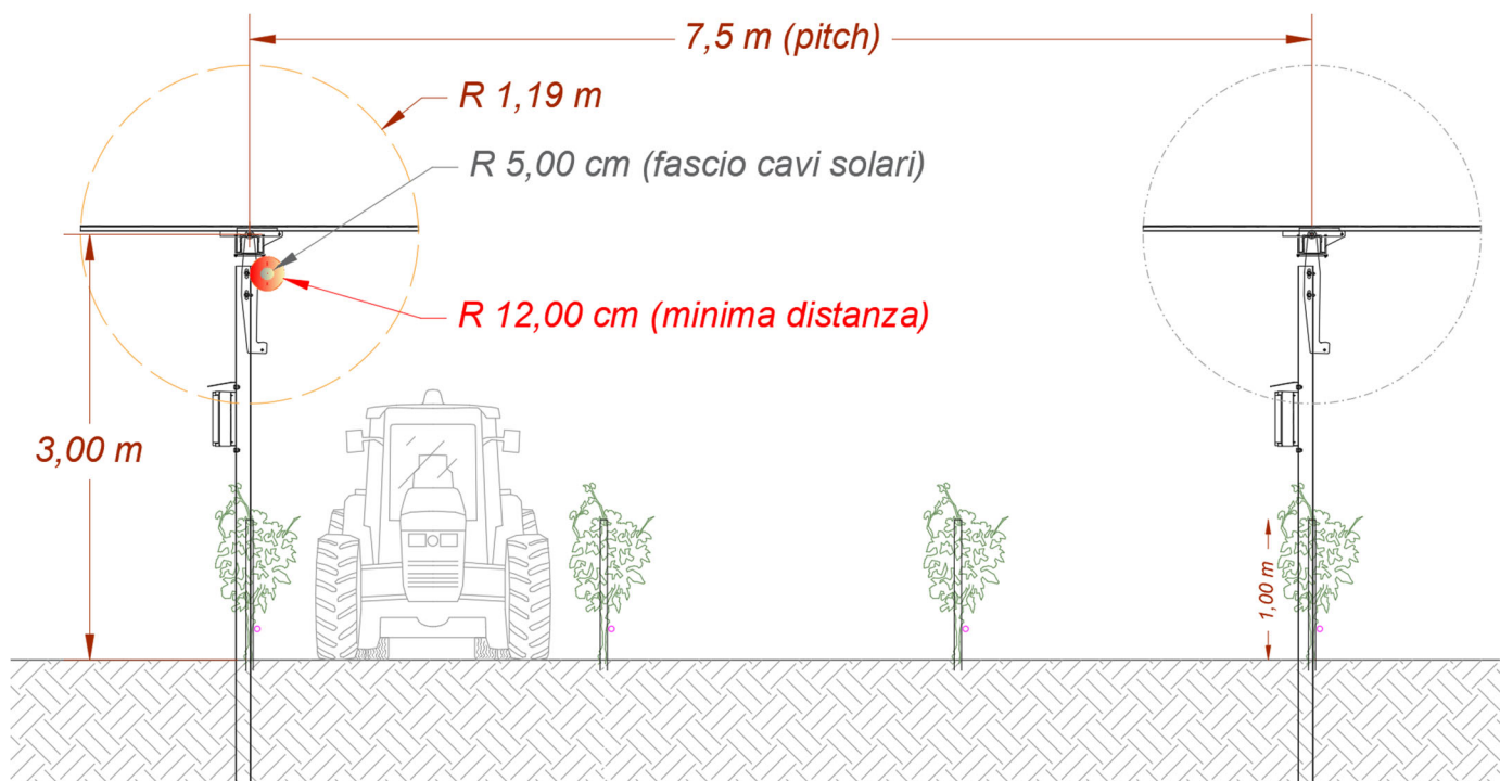
Figura 6 Emissione EM (minima distanza [cm] sotto il tracker)
