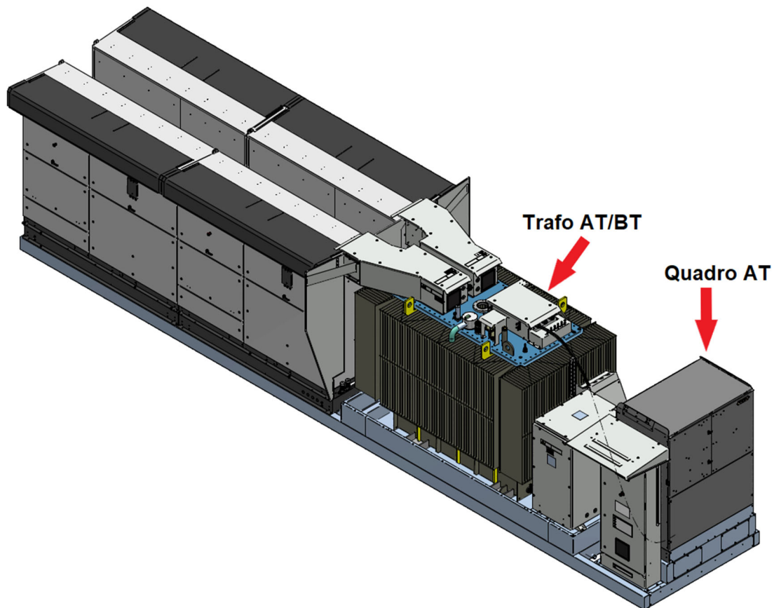
Figura 7 Power Station Ingecon SUN FSK (tipologico)
