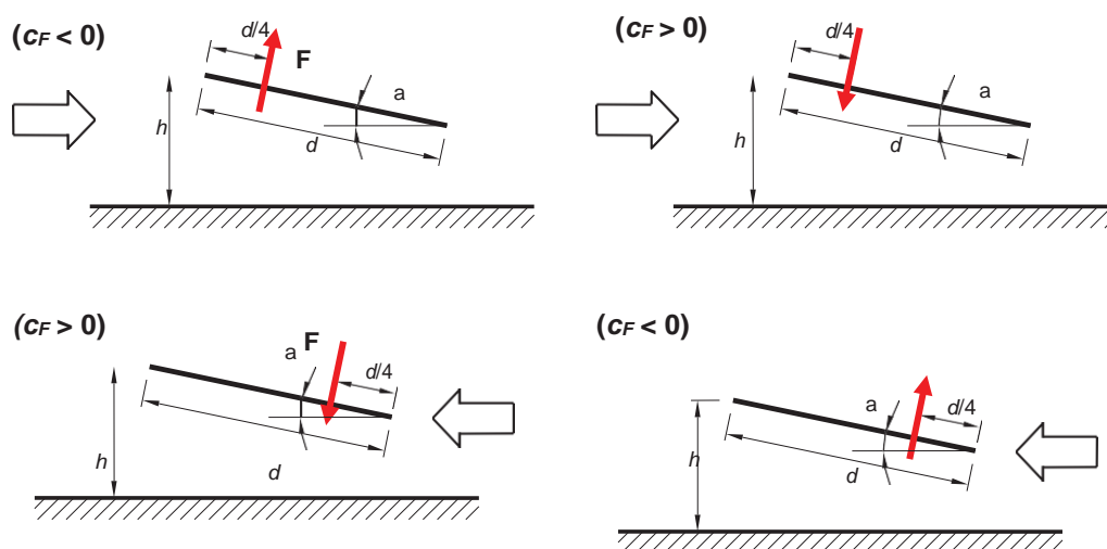
Figura 3: (Rif. Figura G.27 CNR-DT 207 R1/2018) – Tettoie a semplice falda: posizione del punto di applicazione della forza risultante in funzione della direzione di provenienza del vento e della direzione della forza.
