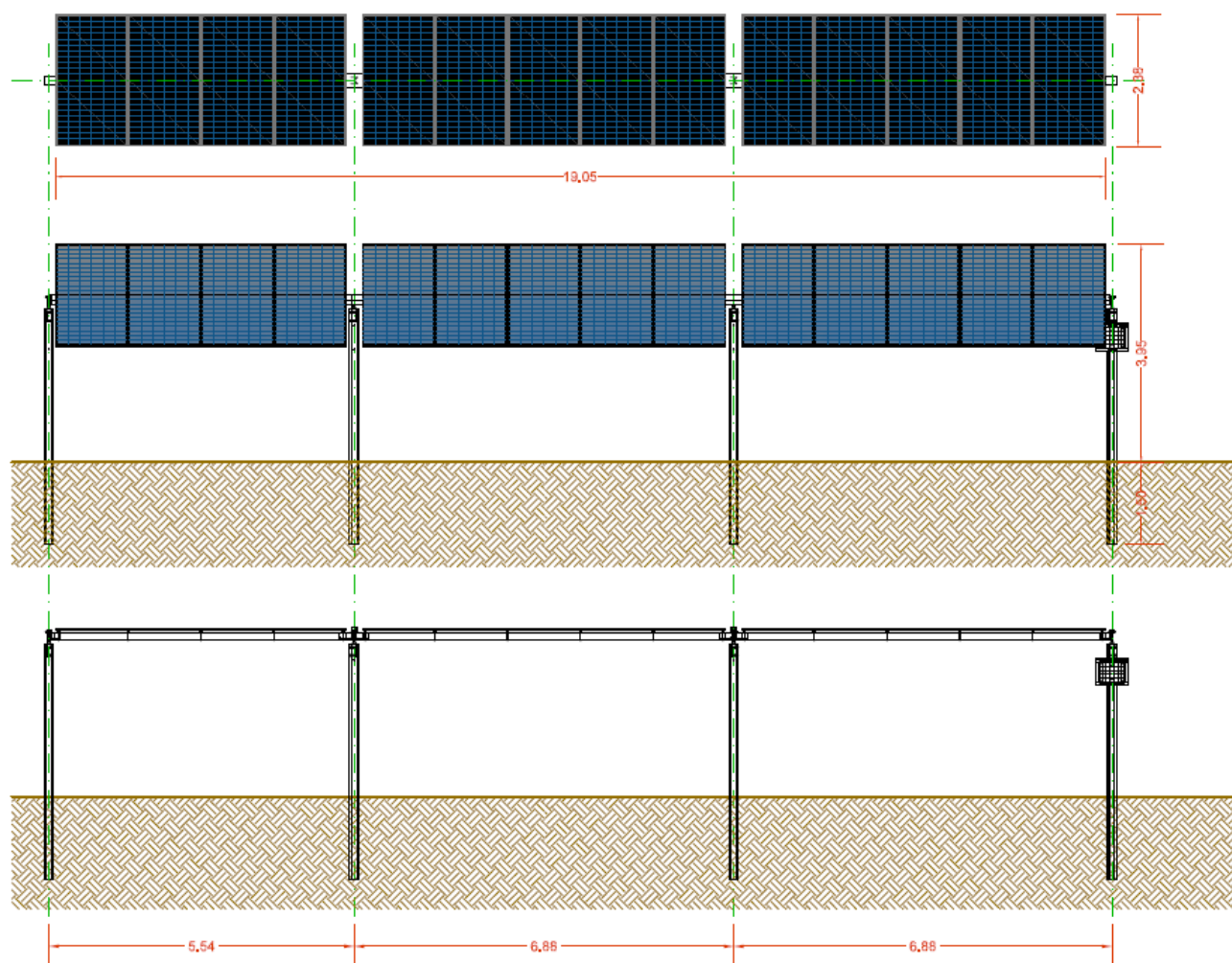
Figura 1: Pianta e prospetti quotati del sistema tracker (inseguitore solare) tipo monoassiale single portrait.
