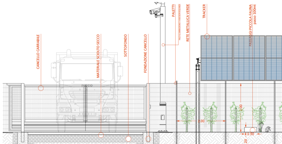
Figura 16 - Particolare delle recinzioni
