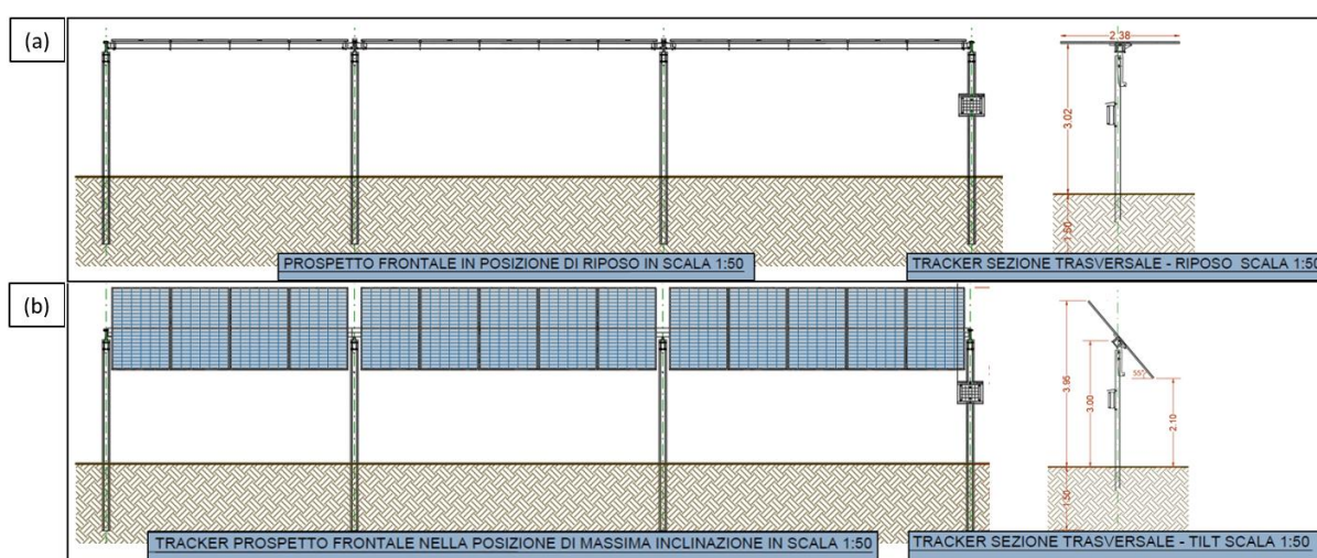
Figura 14 - Tracker: vista in condizione di riposo (a) e di massima inclinazione (b)
