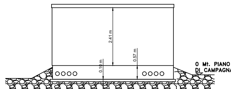
VISTA POSTERIORE
