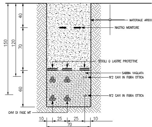
SEZIONE TIPO "D"
