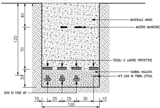
SEZIONE TIPO "C"
