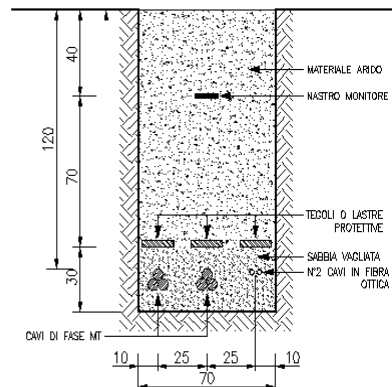
SEZIONE TIPO "B"
