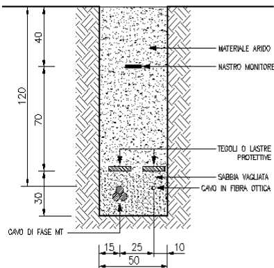
SEZIONE TIPO "A"
