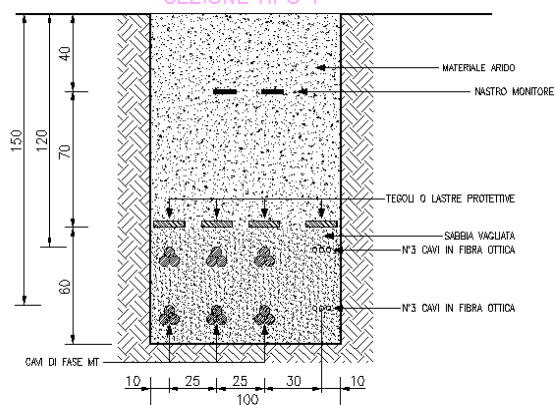
SEZIONE TIPO "F"
