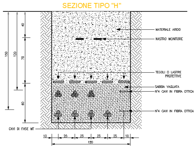
Figura 1: Sezione tipica di posa della linea in cavo su strade sterrate
