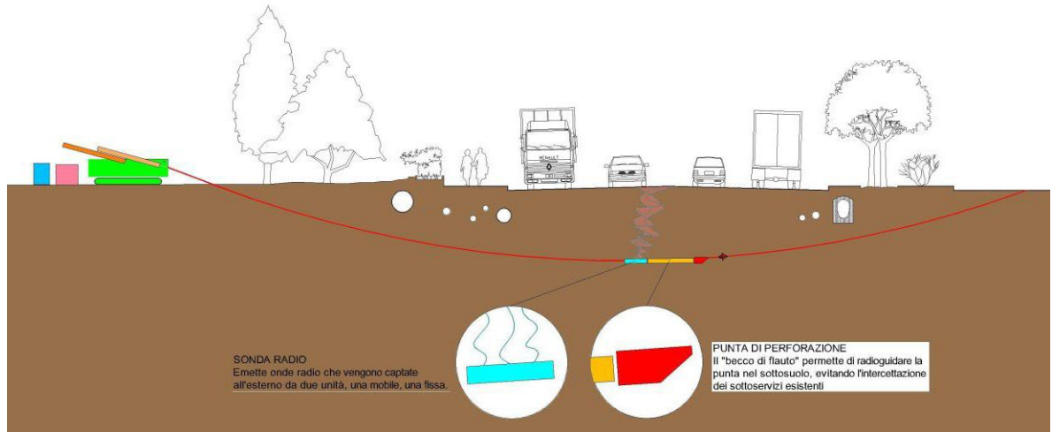
Fase 1: realizzazione foro pilota con controllo altimetrico
