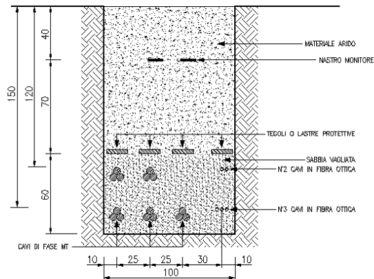
SEZIONE TIPO "E"
