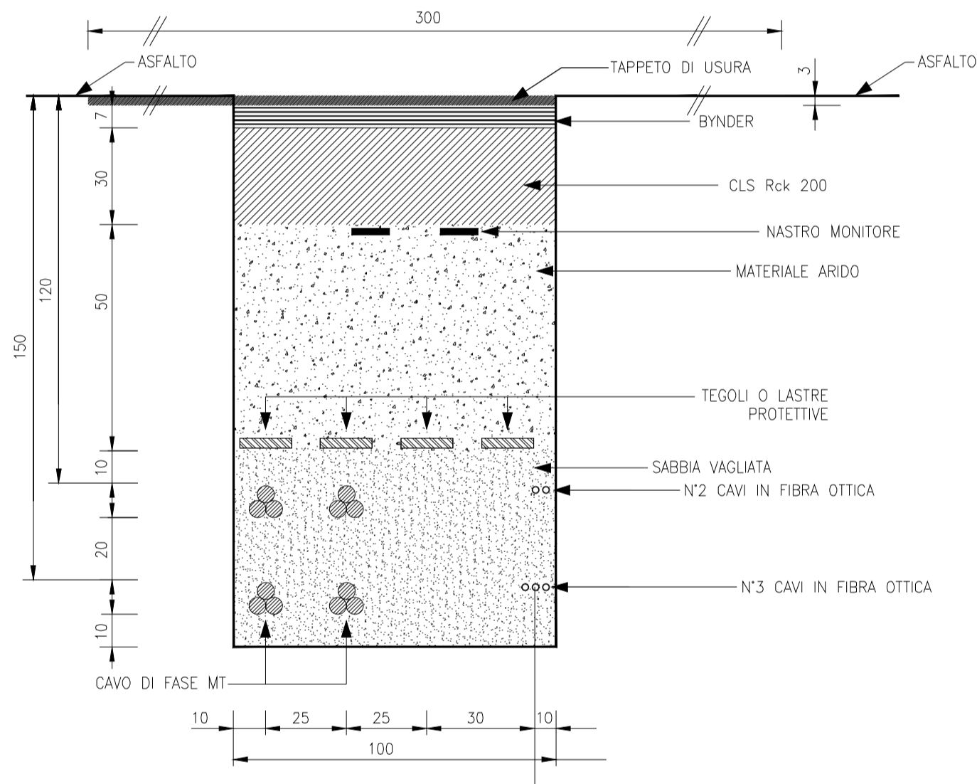
SEZIONE TIPO "DA1"
