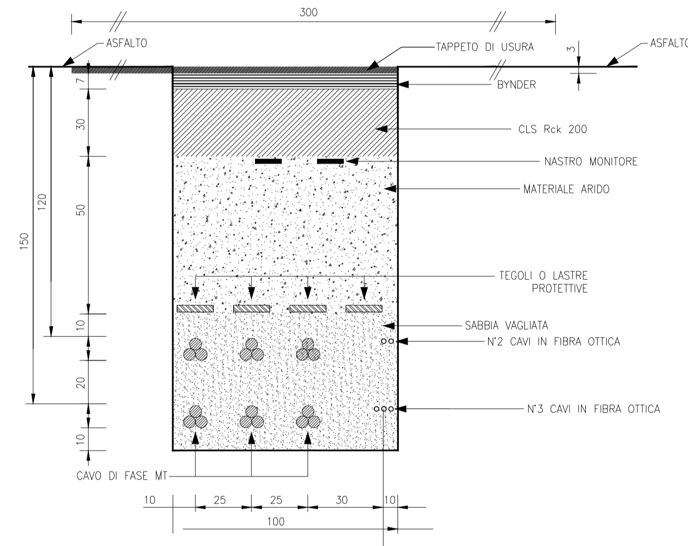
SEZIONE TIPO "FA1"
