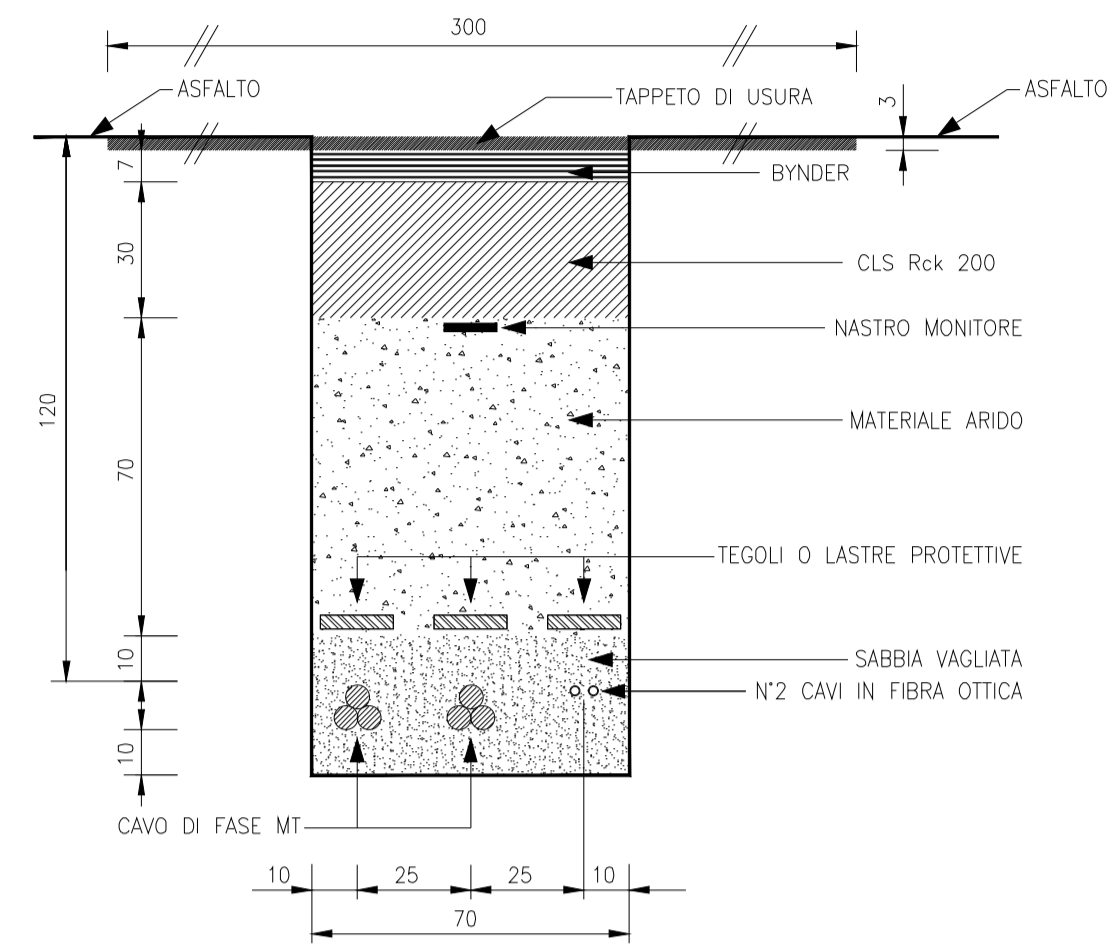
SEZIONE TIPO "BA1"
