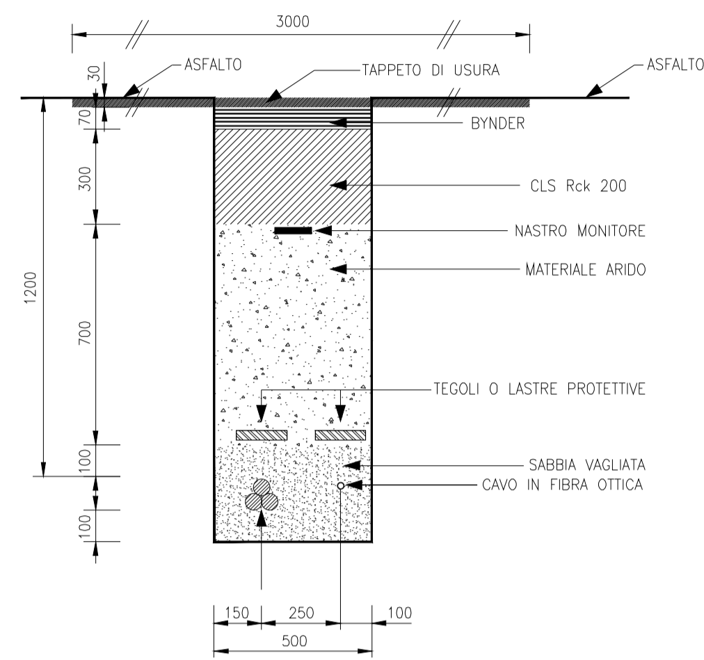
SEZIONE TIPO "AA1"
