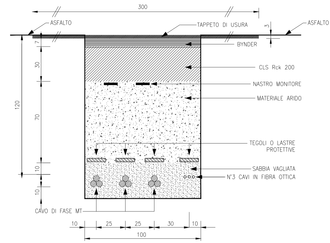
SEZIONE TIPO "CA1"
