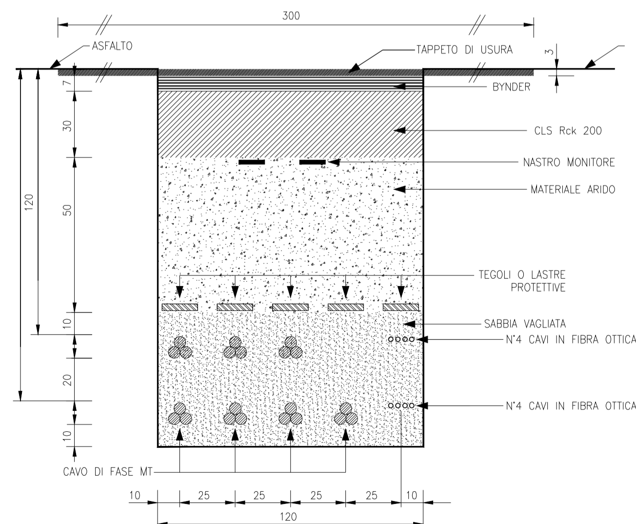
SEZIONE TIPO "HA1"
