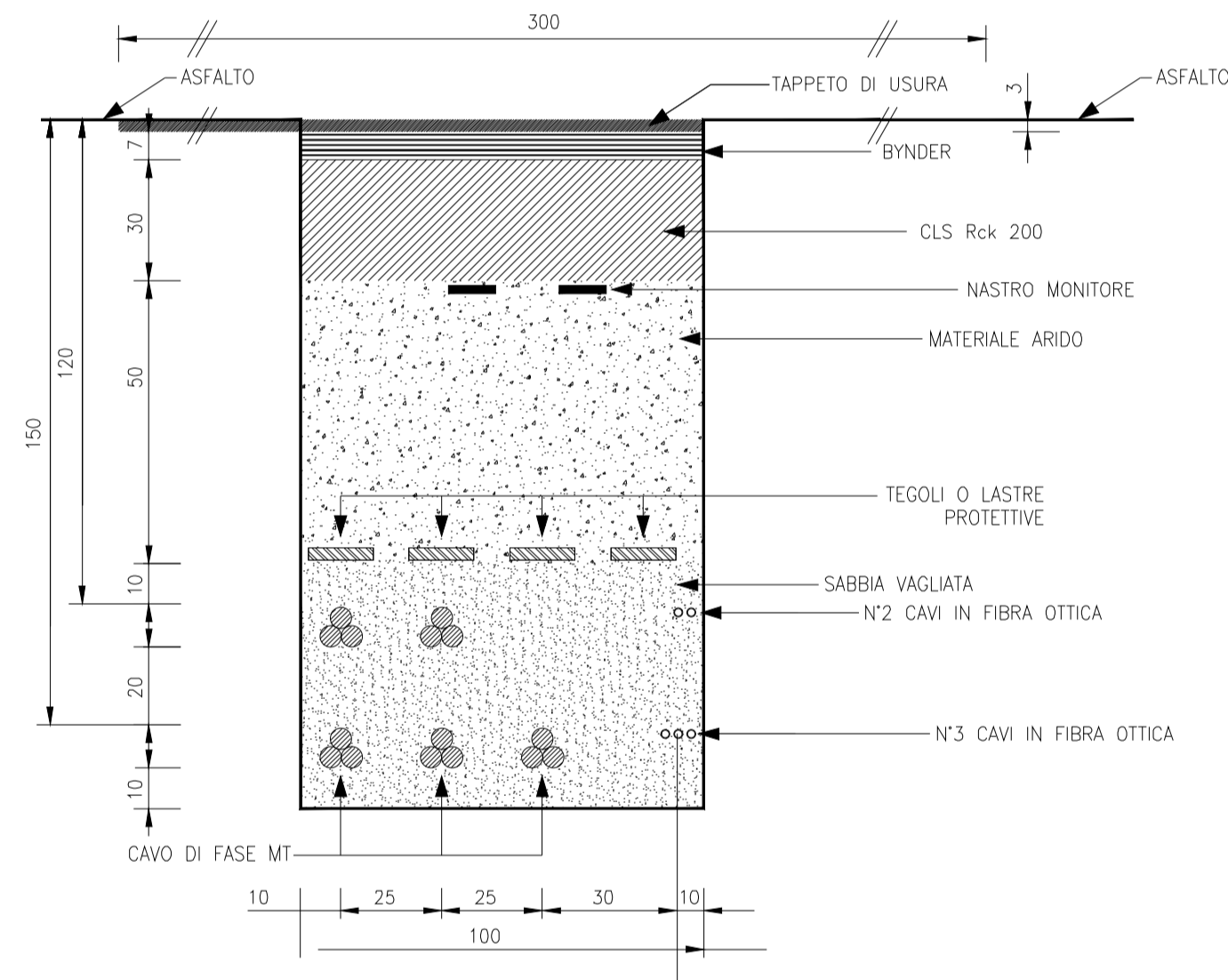
SEZIONE TIPO "HA1"
