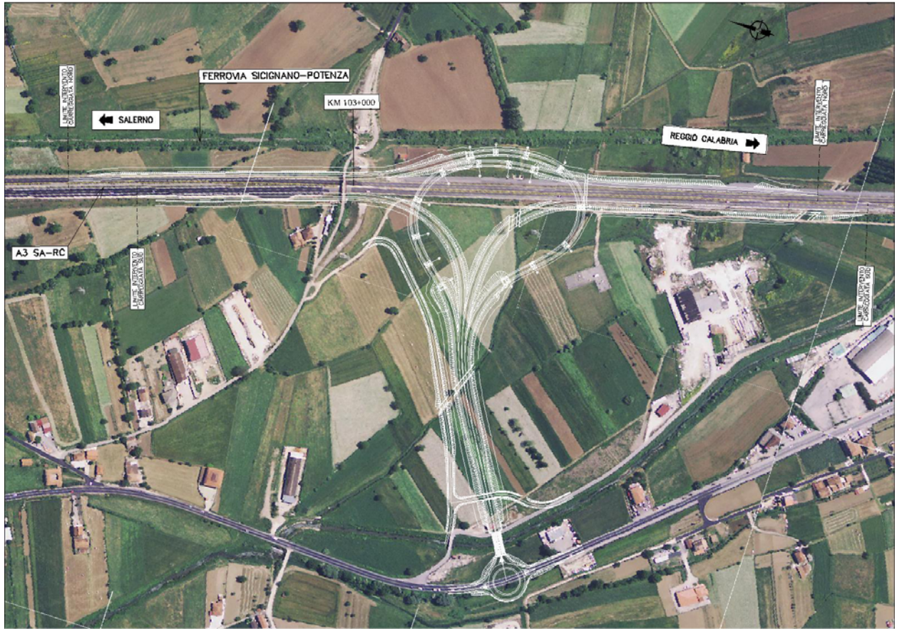
Configurazione nuovo svincolo di Padula - Buonabitacolo
