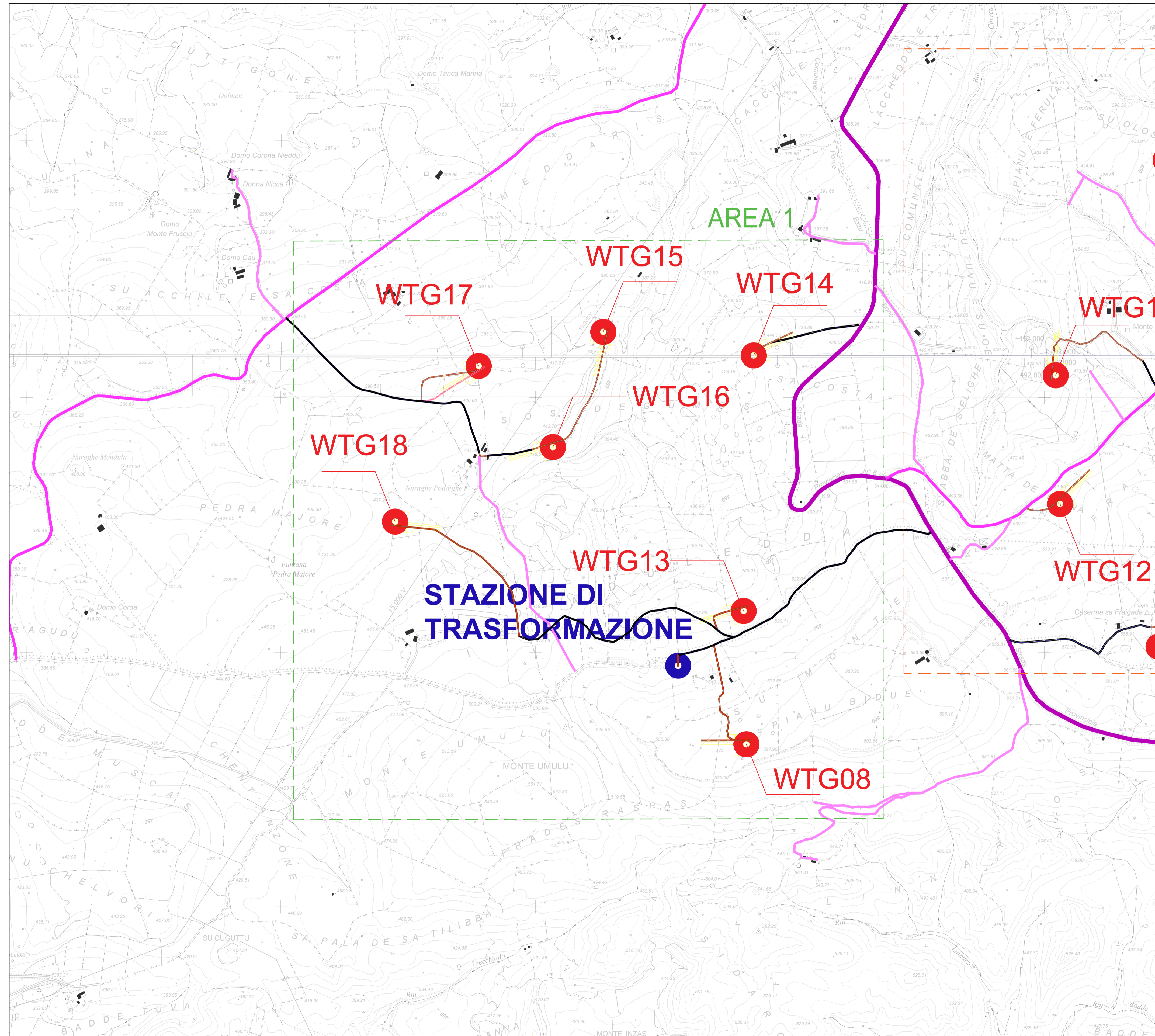
Planimetria generale
