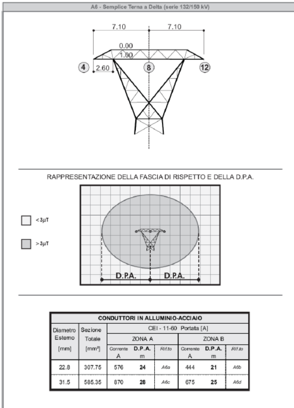
Figura 1 | Linea Guida per l'applicazione dell'Allegato al DM 29.05.08 per linea AT
