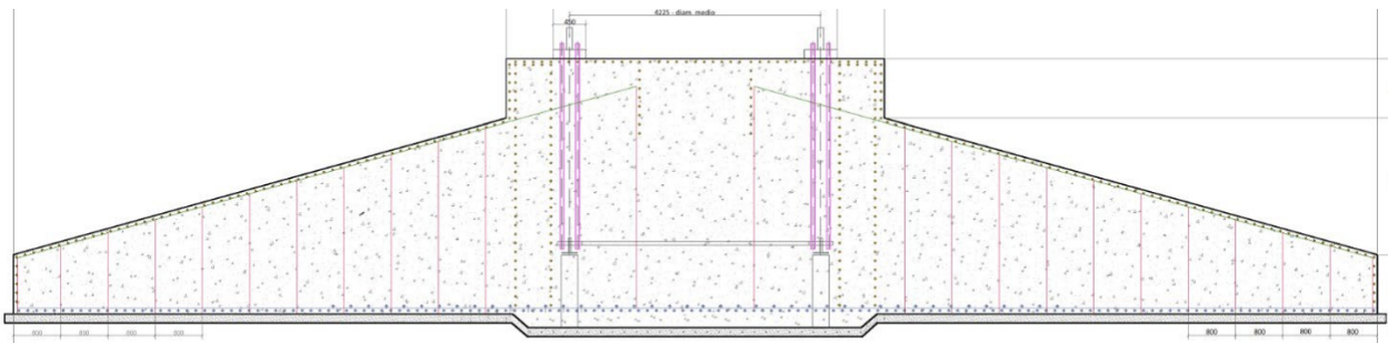
Figura 3 | Schema tipo del plinto di fondazione degli aerogeneratori
