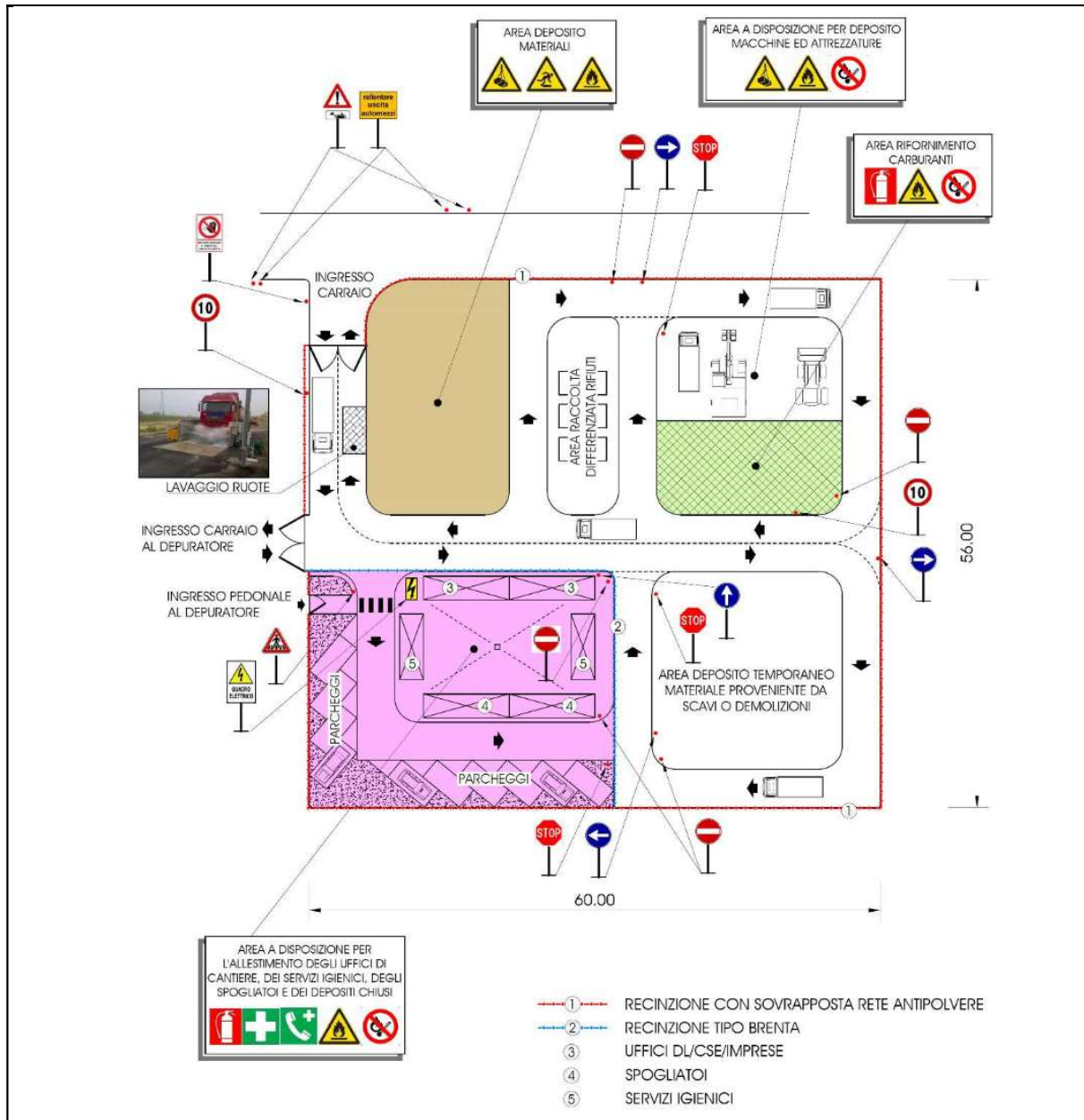
Figura 9.2.1: esempio di schema tipo planimetrico dell'area di cantiere
