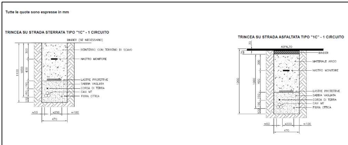
Figura 6.3.2.2: Sezioni tipiche delle trincee cavidotto per una terna di cavi in parallelo su strada sterrata e asfaltata
