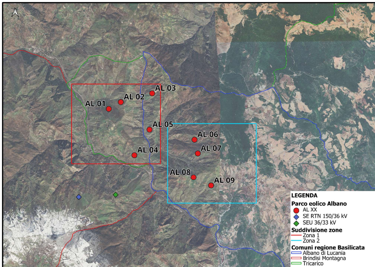
Figura 6.3: Layout d’impianto su ortofoto suddiviso in zone: Zona 1 (rettangolo rosso) e Zona 2 (rettangolo ciano)
