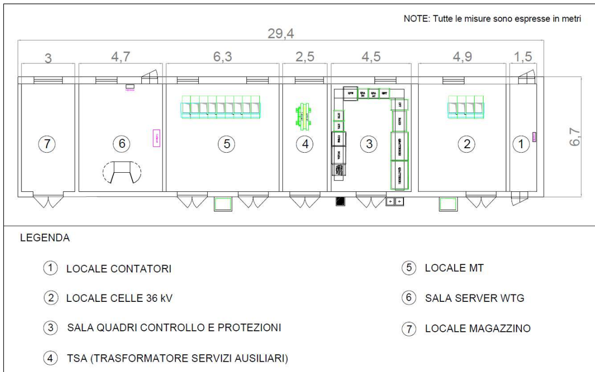
Figura 6.3.3.2: Pianta edificio di controllo SEU 36/33 kV
