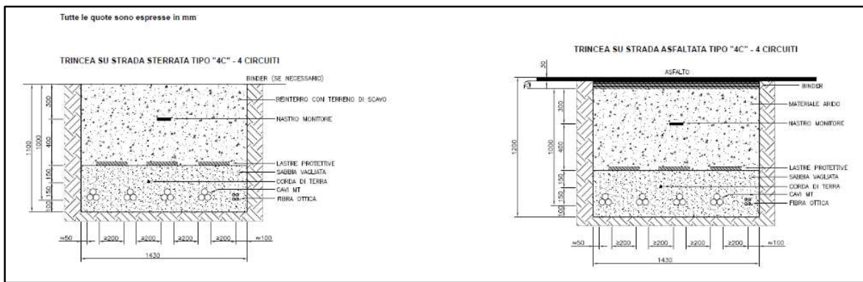
Figura 6.3.2.5: Sezioni tipiche delle trincee cavidotto per quattro terne di cavi in parallelo su strada sterrata e asfaltata
