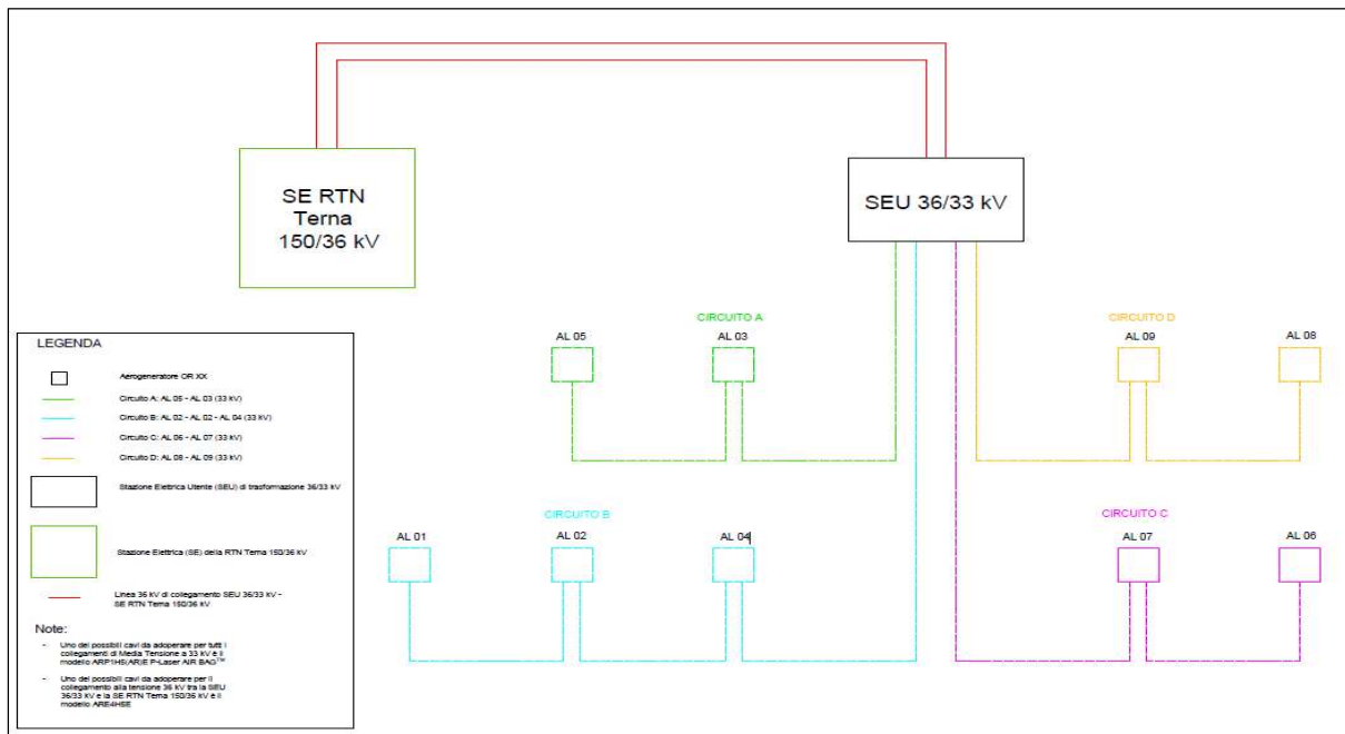
Figura 6.3.2.1: Schema a blocchi del Parco Eolico Albano
