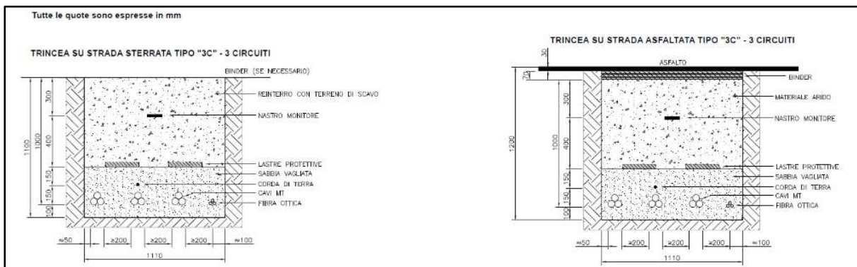
Figura 6.3.2.4: Sezioni tipiche delle trincee cavidotto per tre terne di cavi in parallelo su strada sterrata e asfaltata
