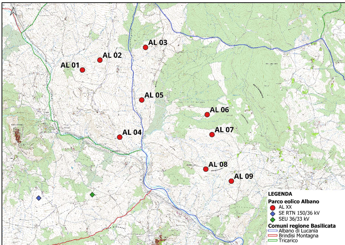
Figura 6.2: Layout d'impianto su CTR con i limiti amministrativi dei comuni interessati
