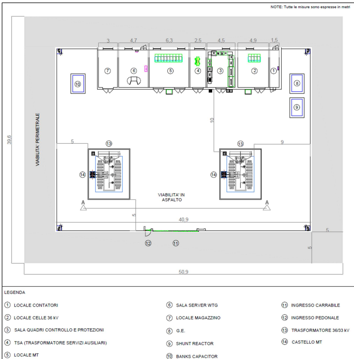
Figura 6.3.3.1: Planimetria elettromeccanica della Stazione Elettrica Utente 36/33 kV
