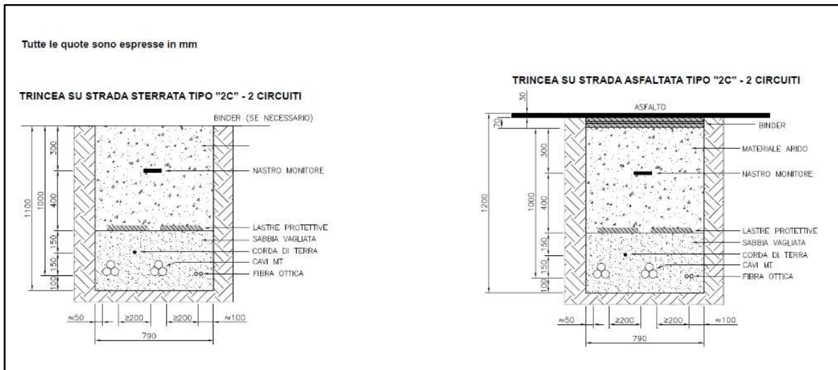
Figura 6.3.2.3: Sezioni tipiche delle trincee cavidotto per due terne di cavi in parallelo su strada sterrata e asfaltata
