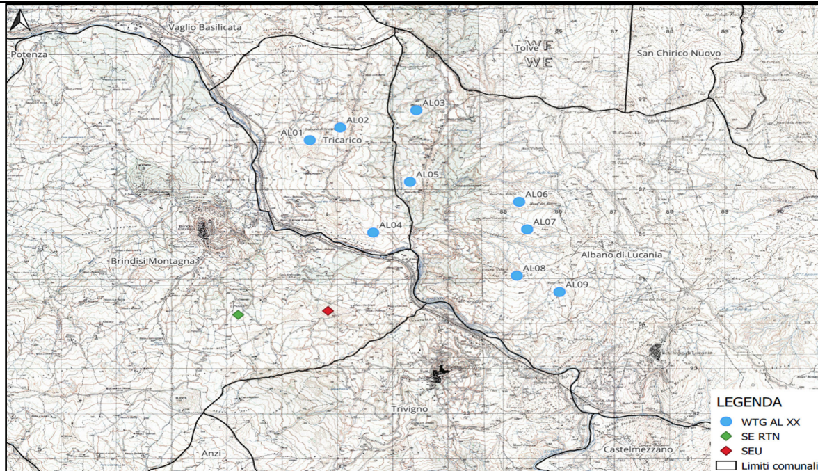
Figura 2.2: Layout d’impianto su IGM con i limiti amministrativi dei comuni interessati
