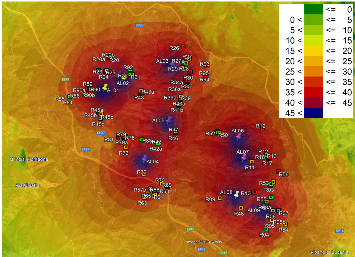
Siemens Gamesa SG 6.0 - D170 - H135: Sound Power Levels [101,0 dBA]- MAPPA VELOCITA' 7ms
