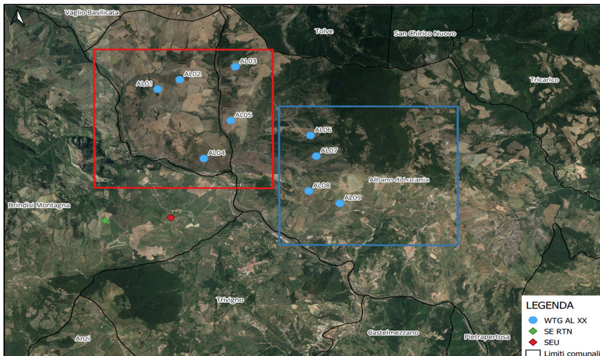
Figura 2.3: Layout d’impianto su ortofoto suddiviso in zone: Zona 1 (rosso) e Zona 2 (blu)
