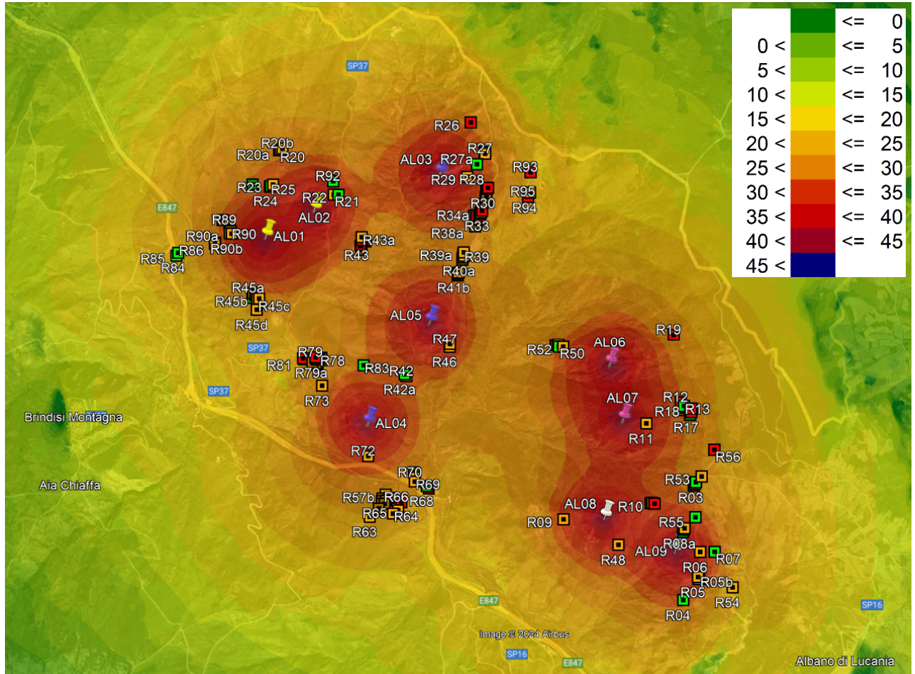
Siemens Gamesa SG 6.0 - D170 - H135: Sound Power Levels [92,2 dBA]- MAPPA VELOCITA' 5ms
