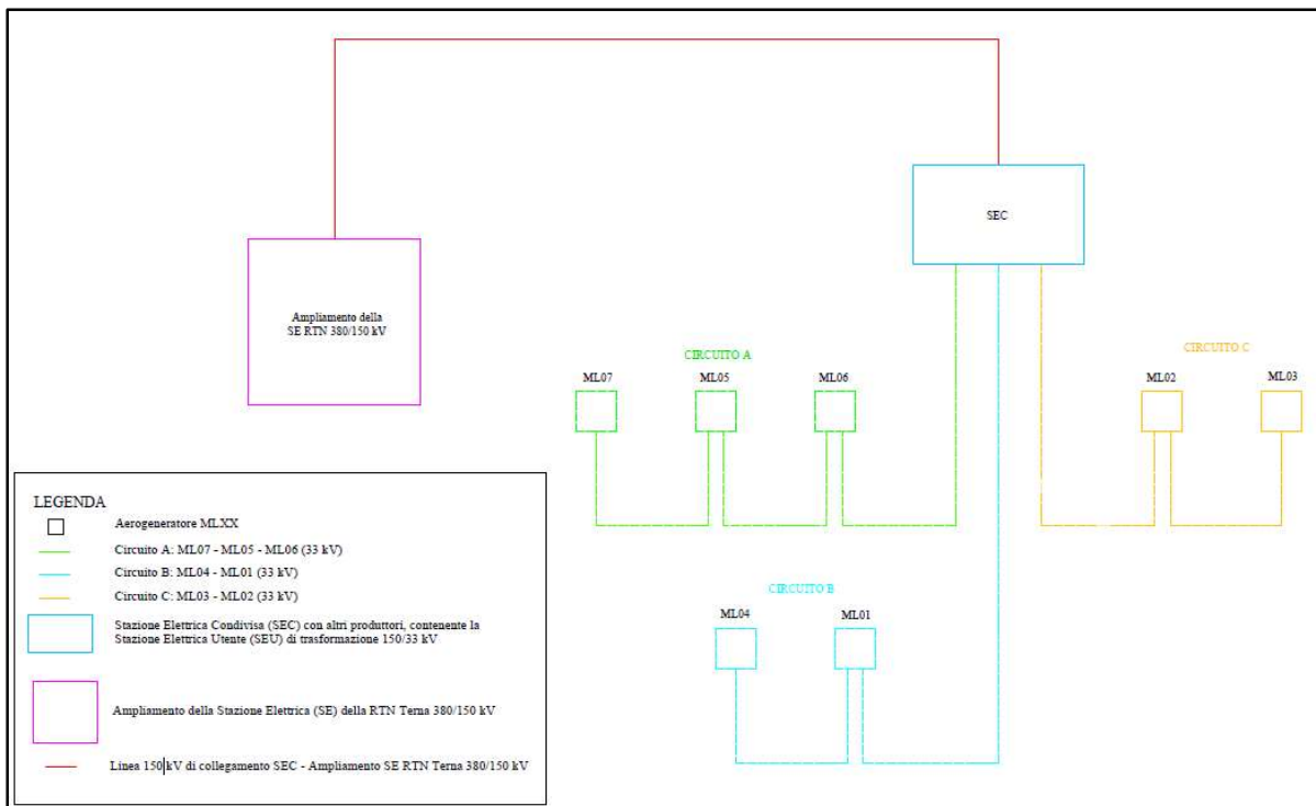
Figura 6.3.2.1: Schema a blocchi del Parco Eolico Melfi
