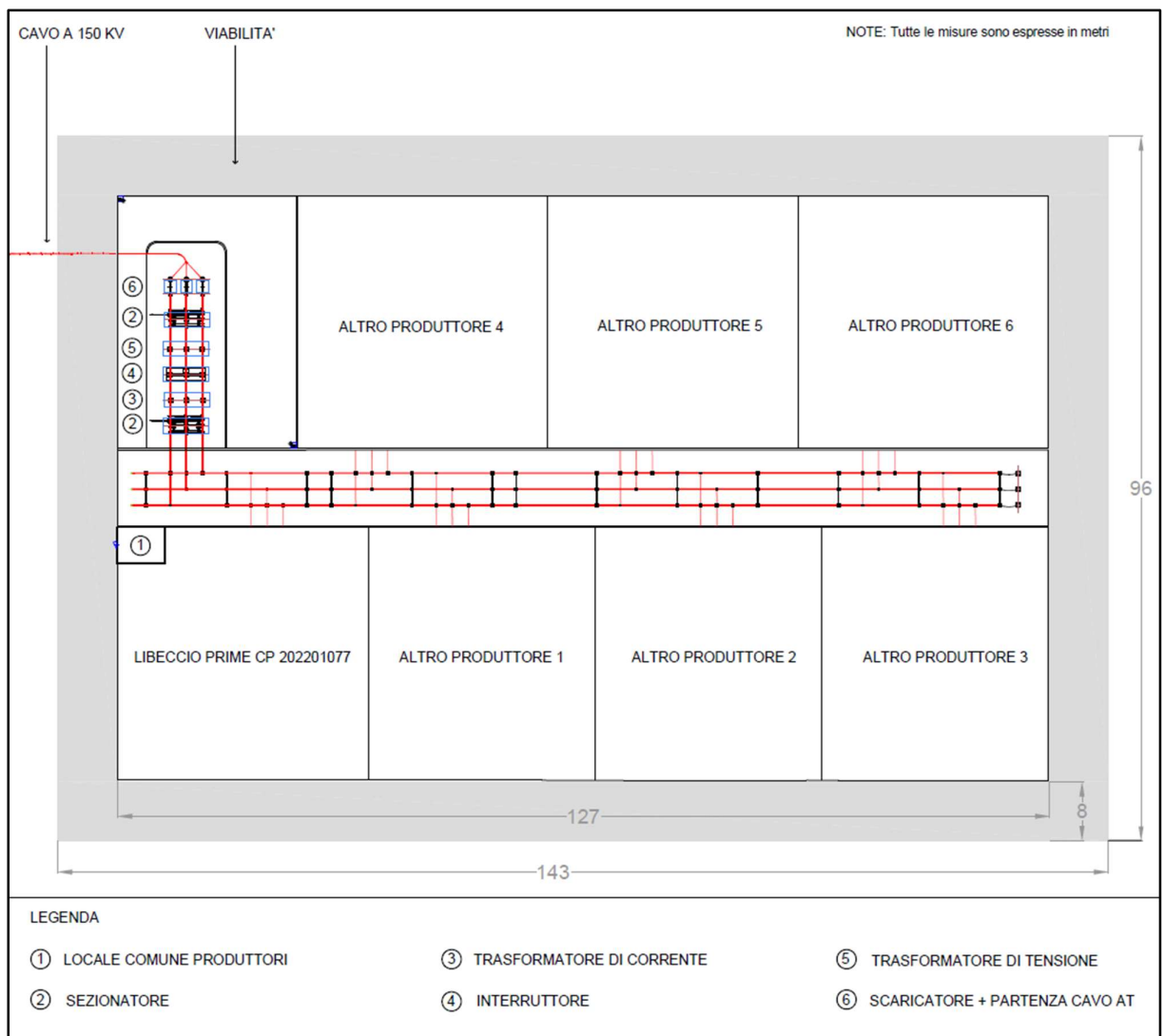
Figura 6.3.4.2: Planimetria elettromeccanica della sottostazione elettrica condivisa
