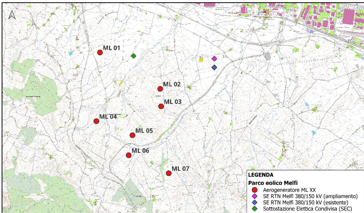
Figura 6.2: Layout d’impianto su CTR
