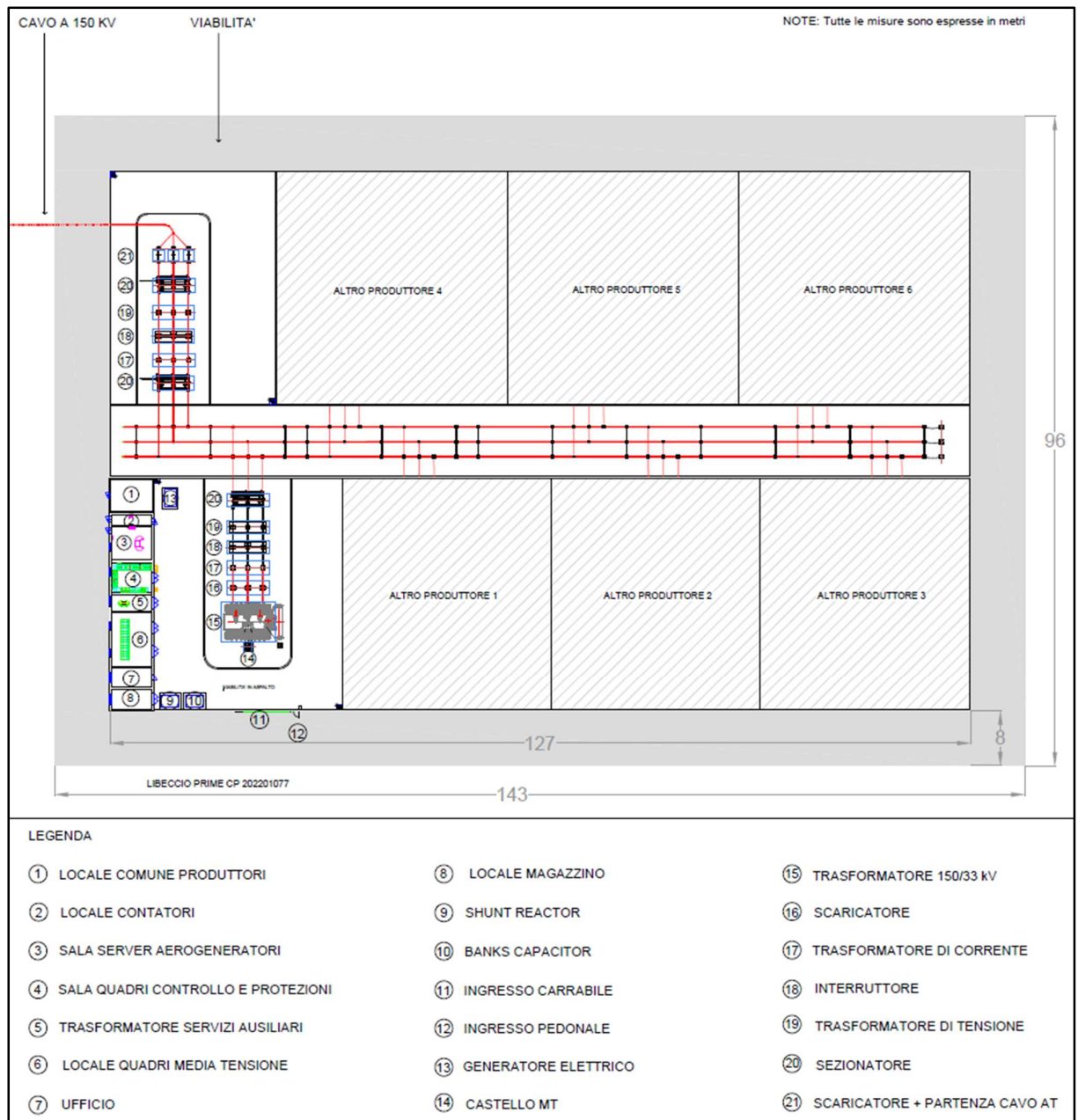
Figura 6.3.3.1: Planimetria elettromeccanica della Sottostazione Elettrica Utente 150/33 kV
