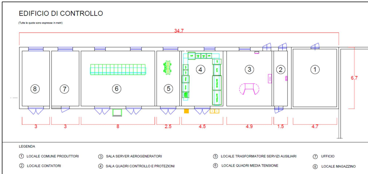
Figura 6.3.3.2: Pianta edificio di controllo SEU 150/33 kV
