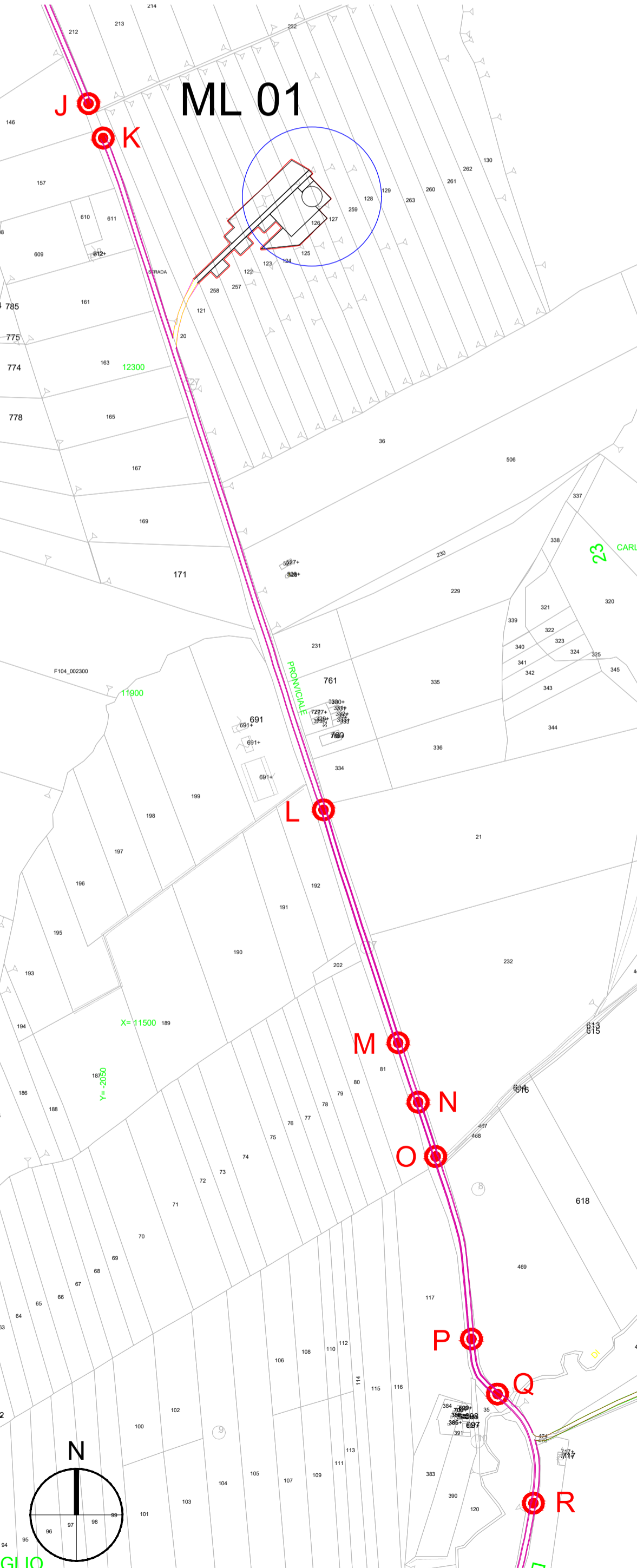
R.d_ADEGUAMENTI TRATTI K-L/L-M/M-N/N-O/O-P/P-Q/Q-R
