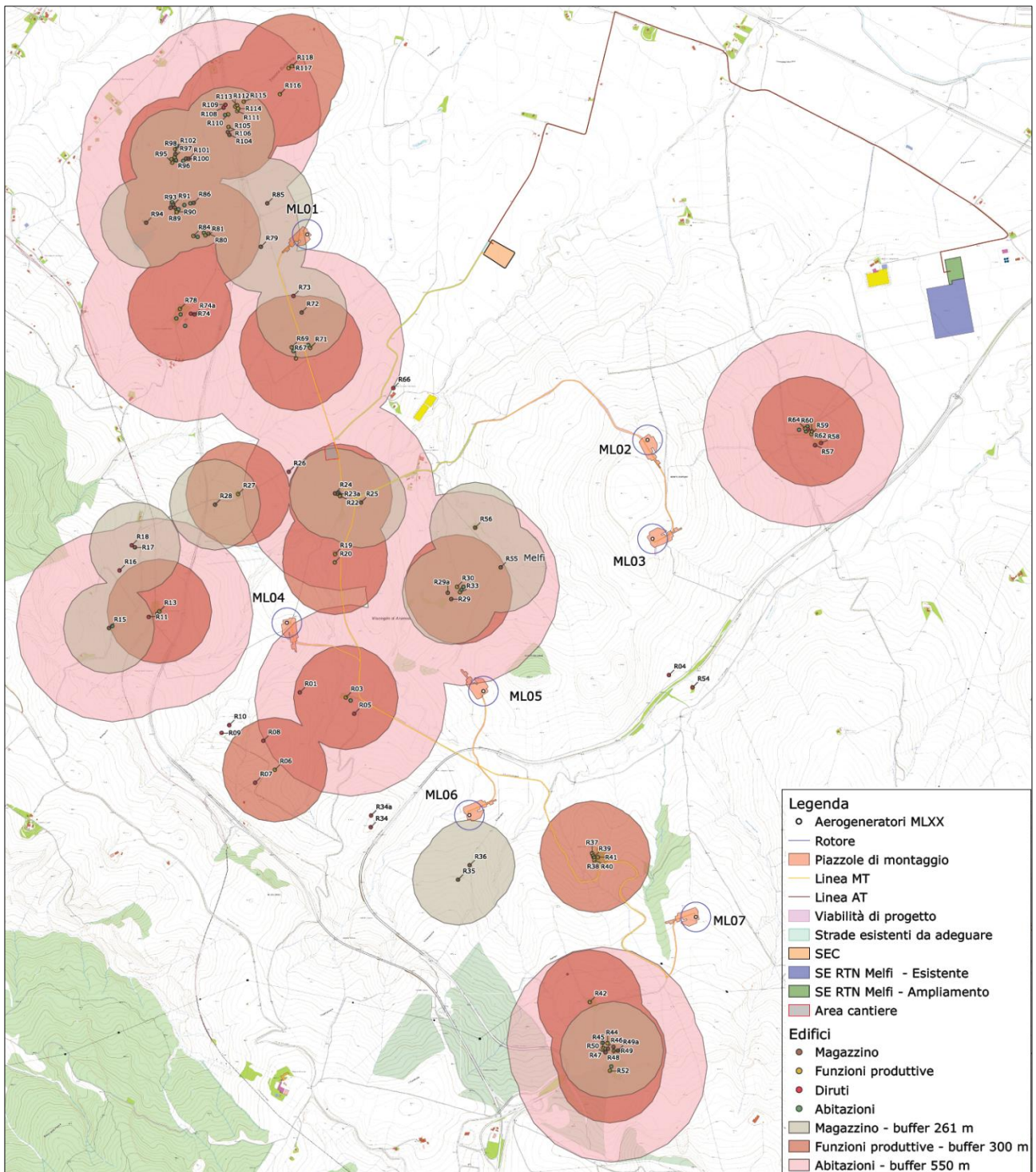
Figura 9.1: Carta delle distanze di sicurezza di edifici dagli aerogeneratori di progetto
