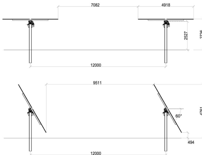
Figura 5.1: Sezione tipo delle stringhe fotovoltaiche tracker doppiavela.
