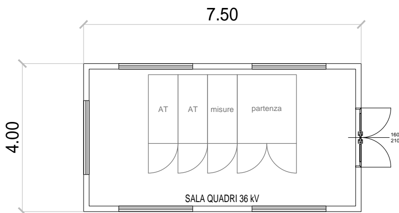
Figura 5.4: Pianta della cabina di smistamento.
