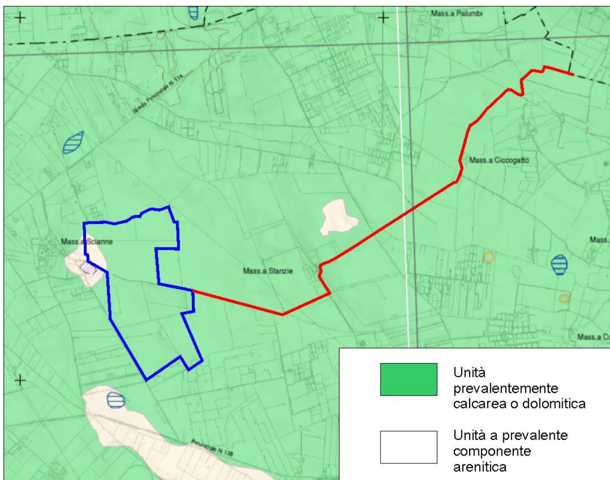
Figura 3.2: Inquadramento geologico dell'area in esame (Estratto dalla Carta Idrogeomorfologica della Regione Puglia – Fogli 511 e 512, scala 1:25.000. Blu = perimetro area impianto; rosso = tracciato cavidotto interrato).
