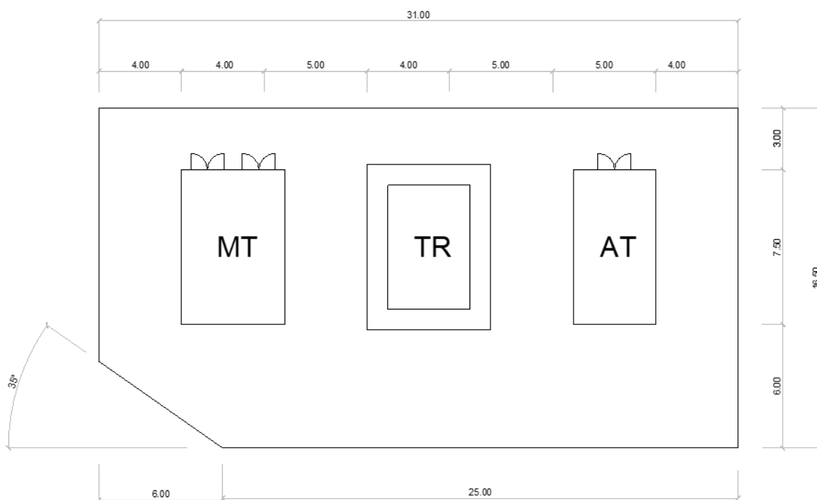
Figura 5.2: Platea di fondazione dell'area di trasformazione e disposizione cabine.
