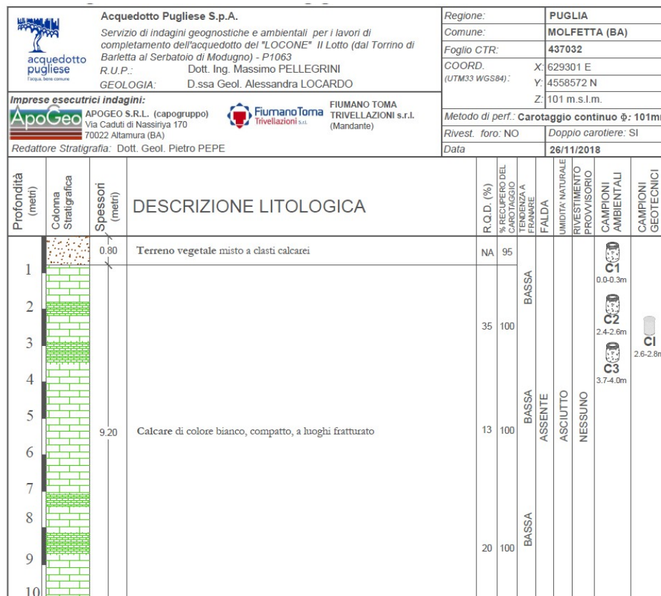
Figura 4.2 – Stratigrafia tipo lungo il tracciato di progetto
