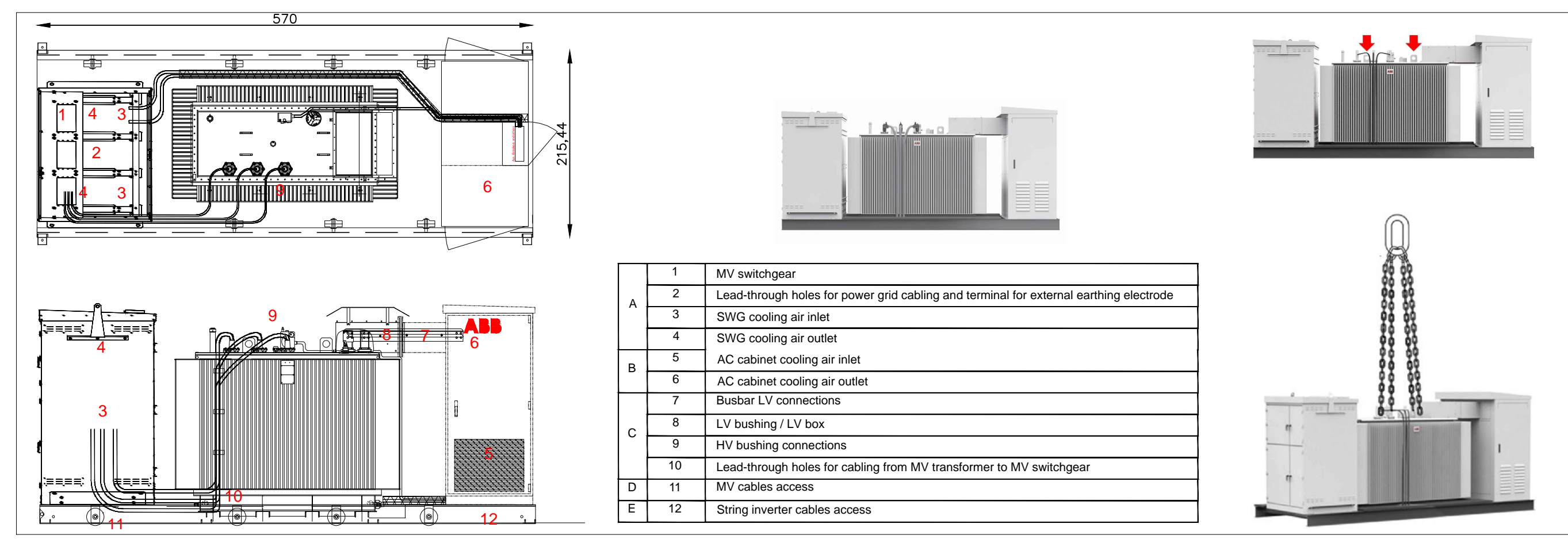
CENTRALE DI TRASFORMAZIONE B.T.M.T. ABB MV COMPACT SKID PVS-175-MVCS
