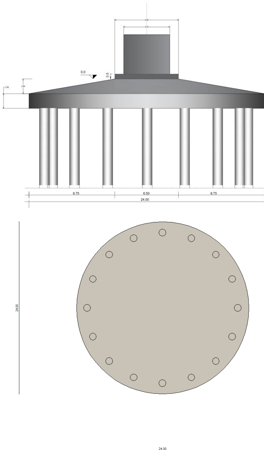
Figura 5: Sezione e fondazione tipo
