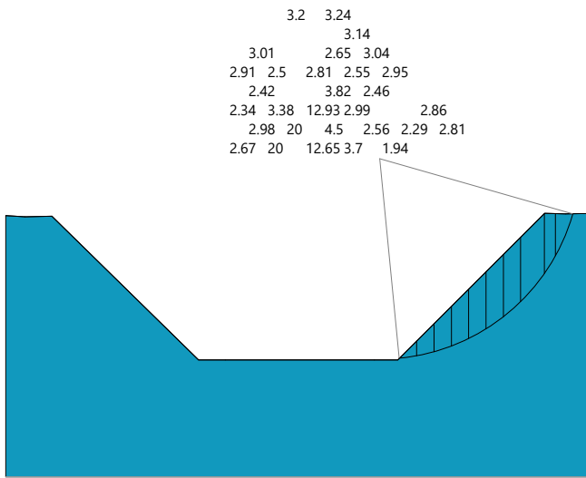
SM02 Sezione 16 fronte di scavo 5.03
