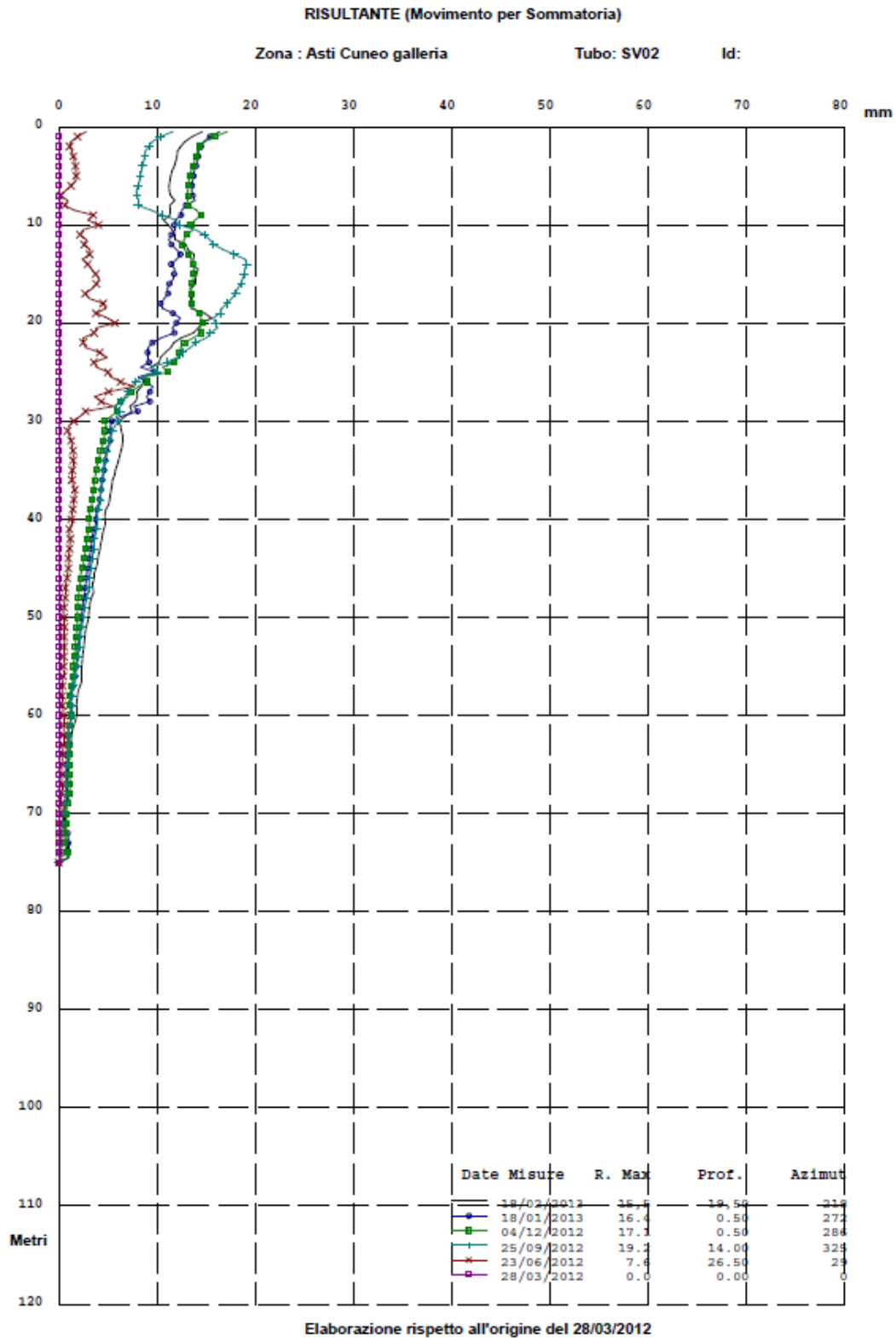
Figura 6.6B – Risultante movimenti inclinometro SOT-VE-002
