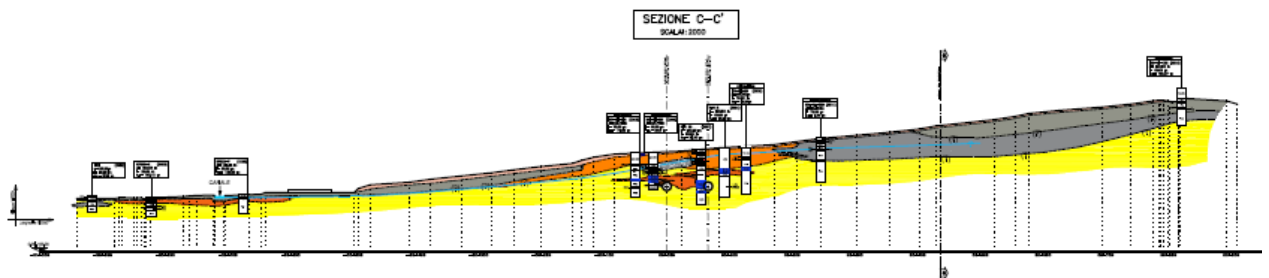
Figura 10.13_ Sezione C-C'
