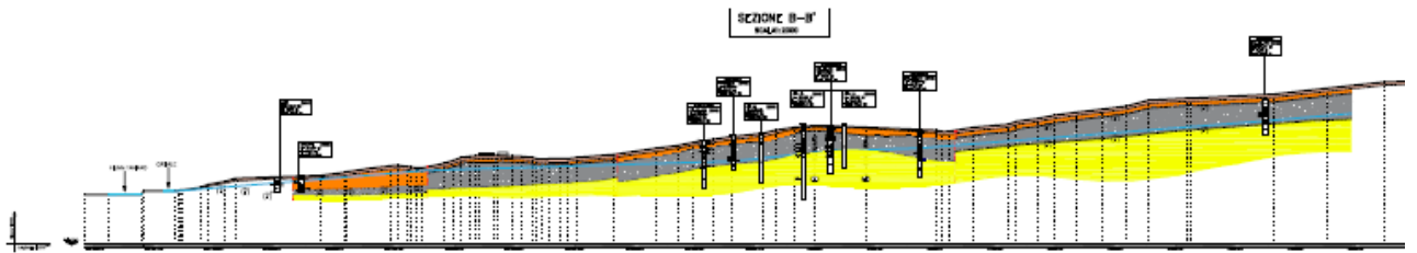
Figura 10.10 – Sezione B-B'
