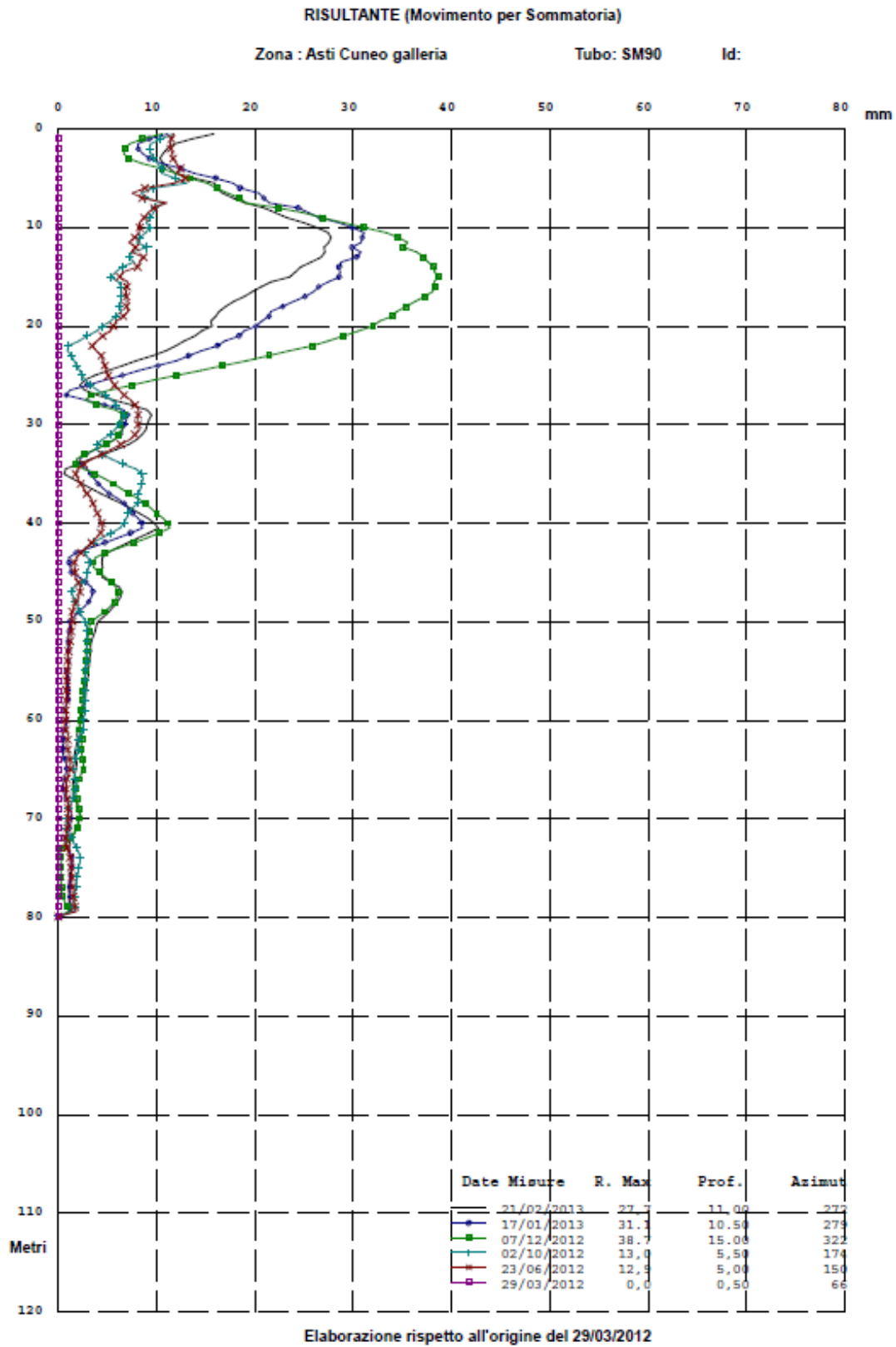
Figura 6.6A – Risultante movimenti inclinometro SOT-MO-090
