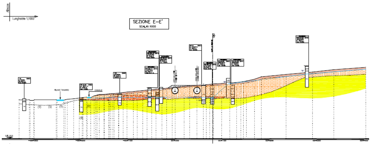
Figura 10.18 – Sezione E-E'
