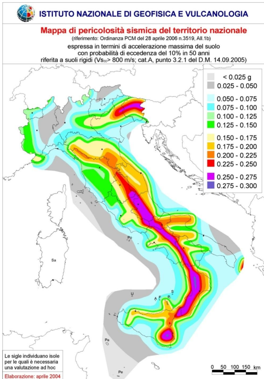
Figura 12.2 – Mapa di pericolosità sismica dell'intero territorio nazionale redatta dall'INGV. La figura è stata tratta dal sito dell'INGV: http://zonesismiche.mi.ingv.it/
