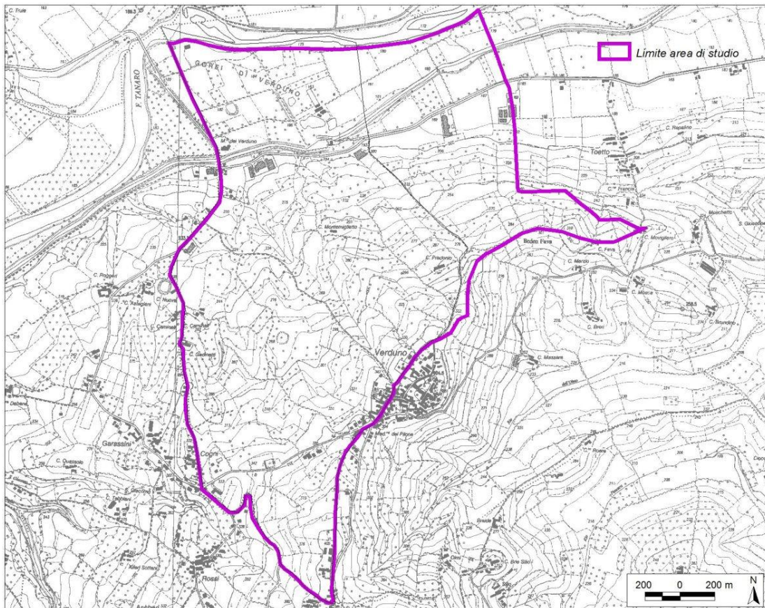
Figura 7.1 – Area di studio forme carsiche
