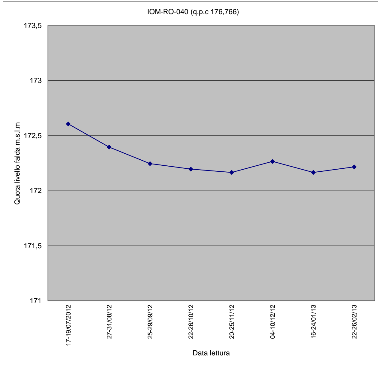
Piezometro IOM-RO-040
