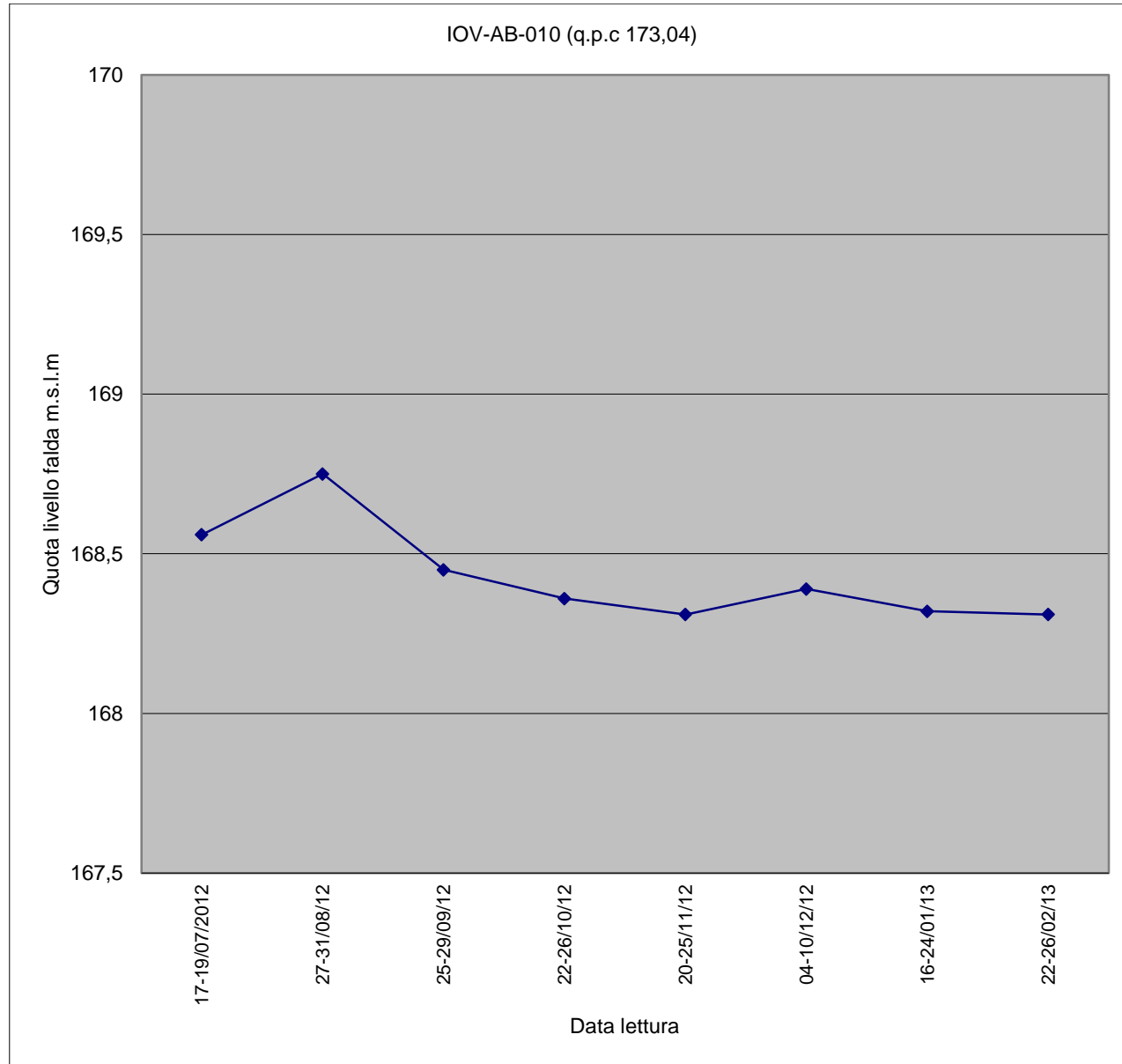
Piezometro IOV-AB-040
