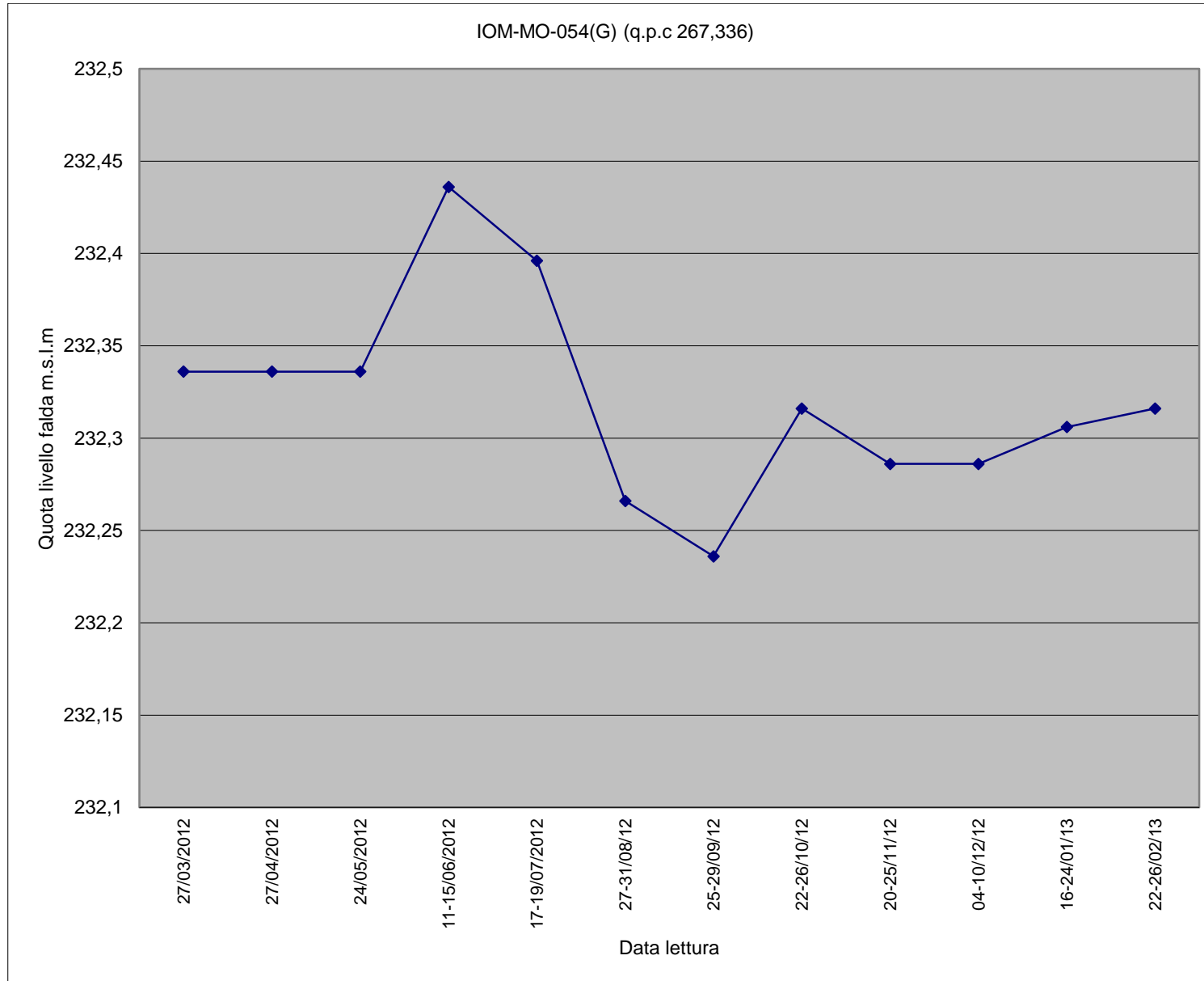
Piezometro IOM-MO-054(G)
