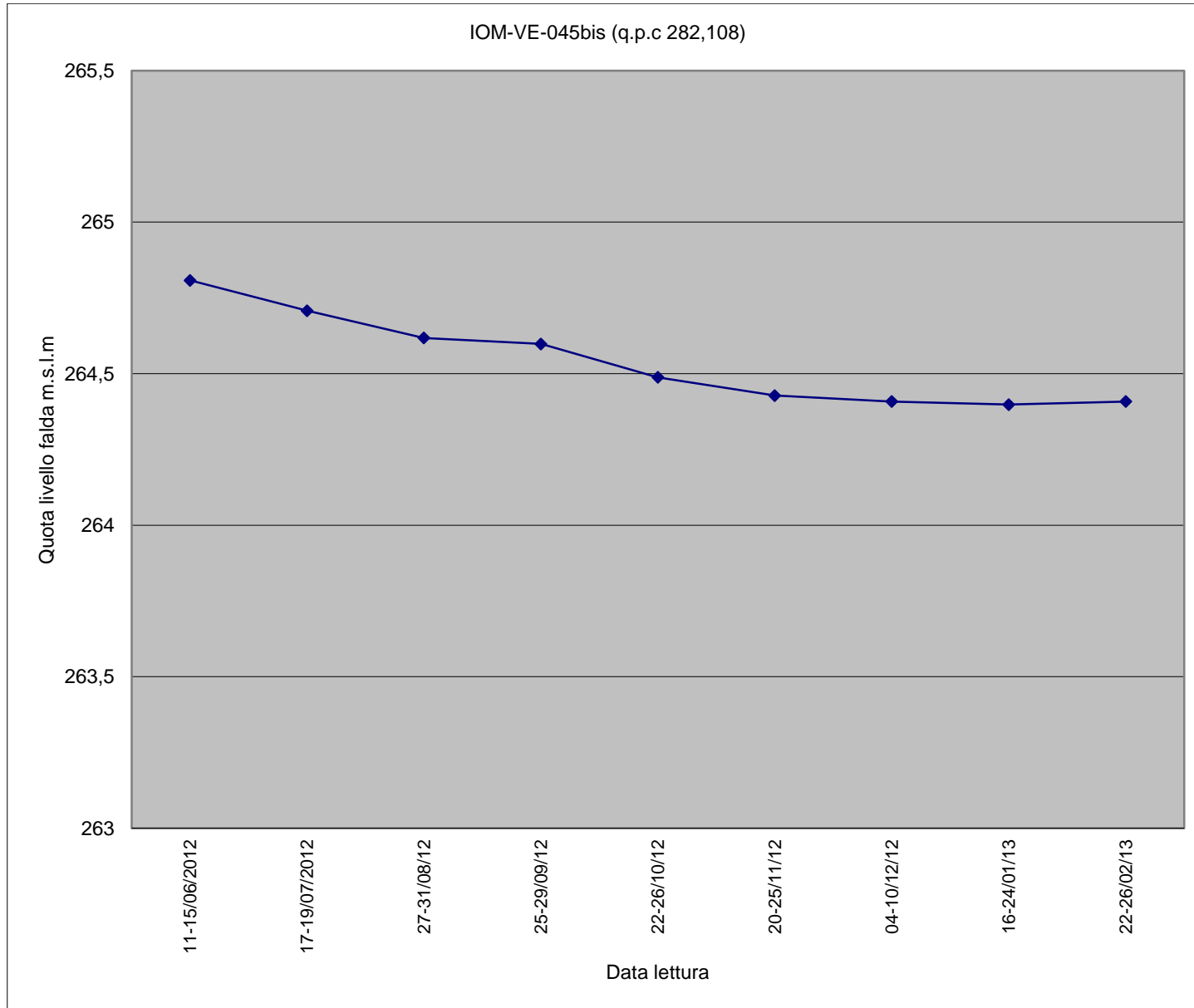
Piezometro IOM-VE-045BIS
