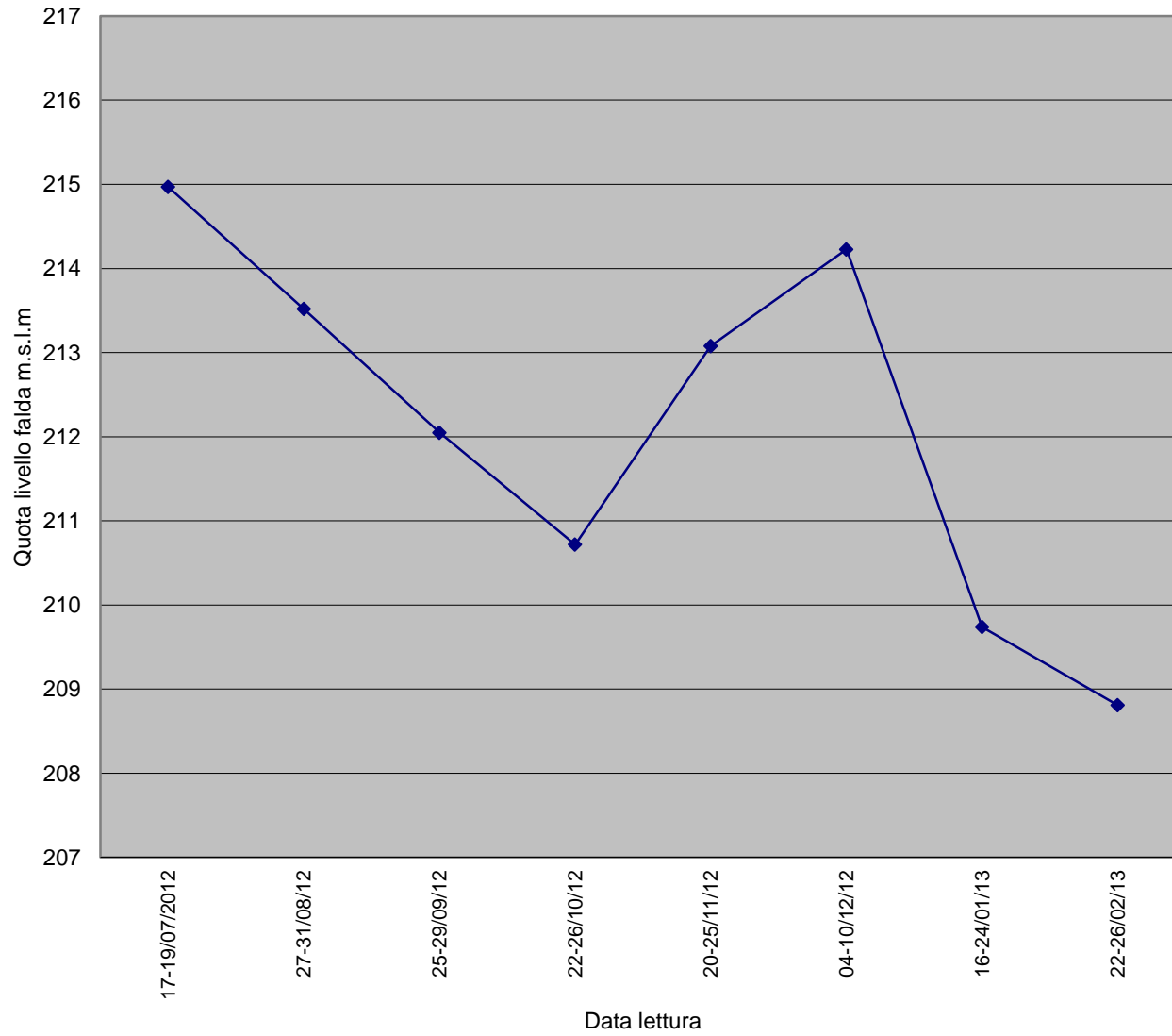
IOV-VE-010 (q.p.c 224,408)
