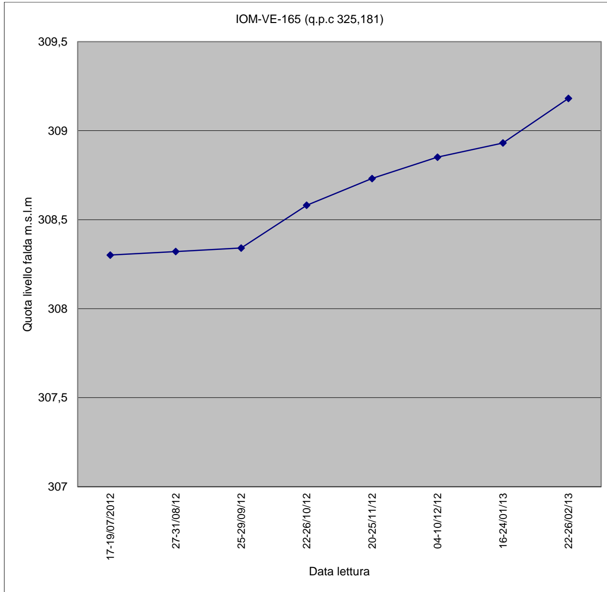
Piezometro IOM-VE-165
