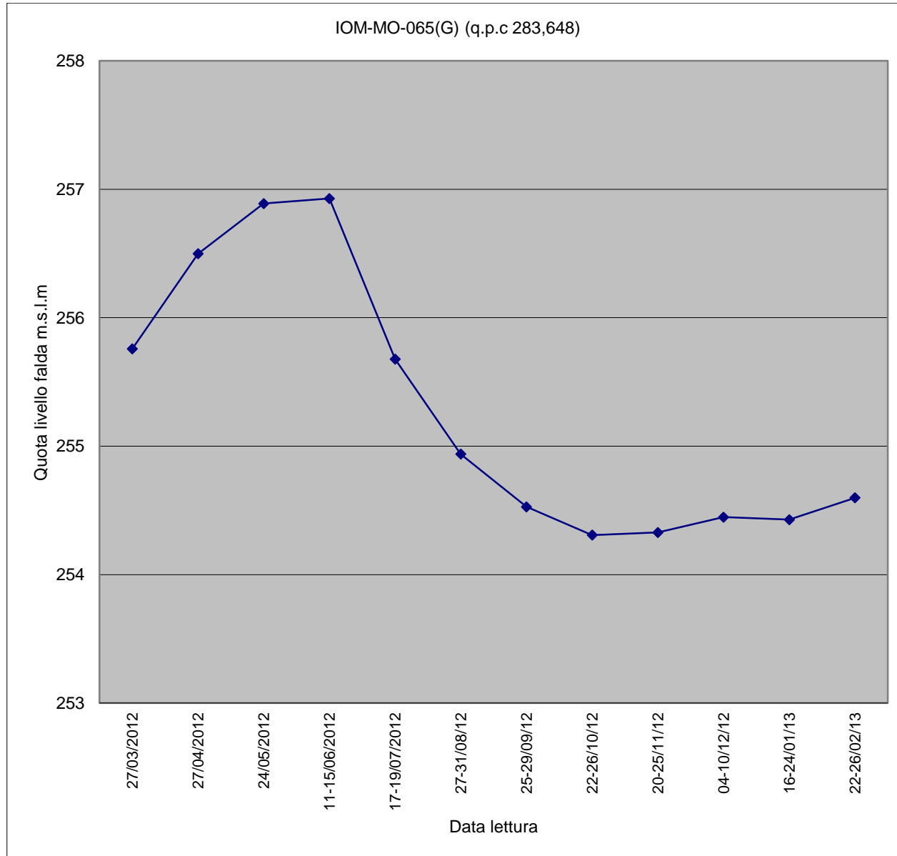
Piezometro IOM-MO-065(G)
