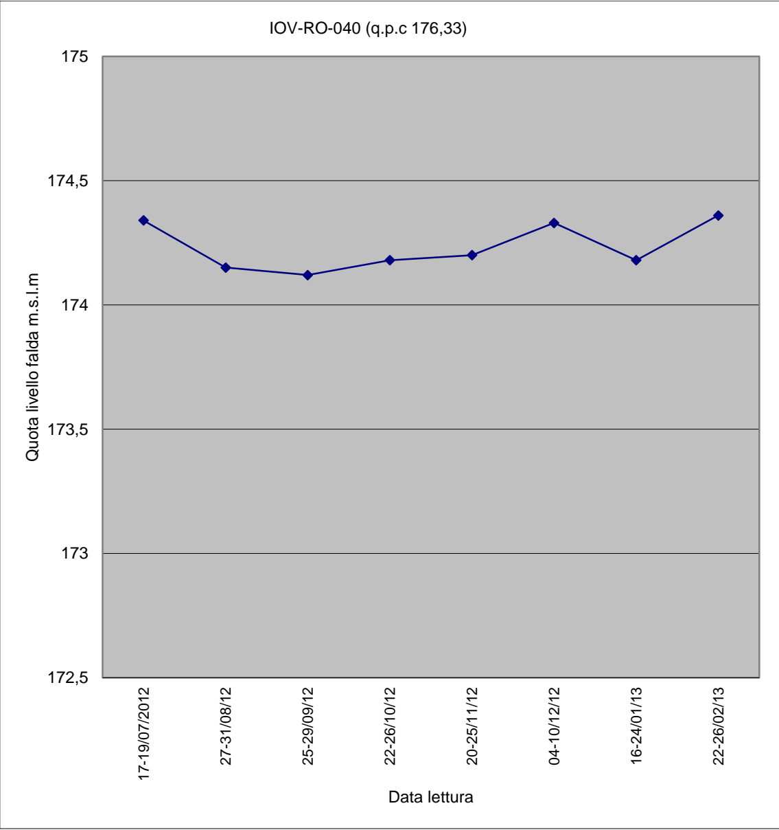
Piezometro IOV-RO-040
