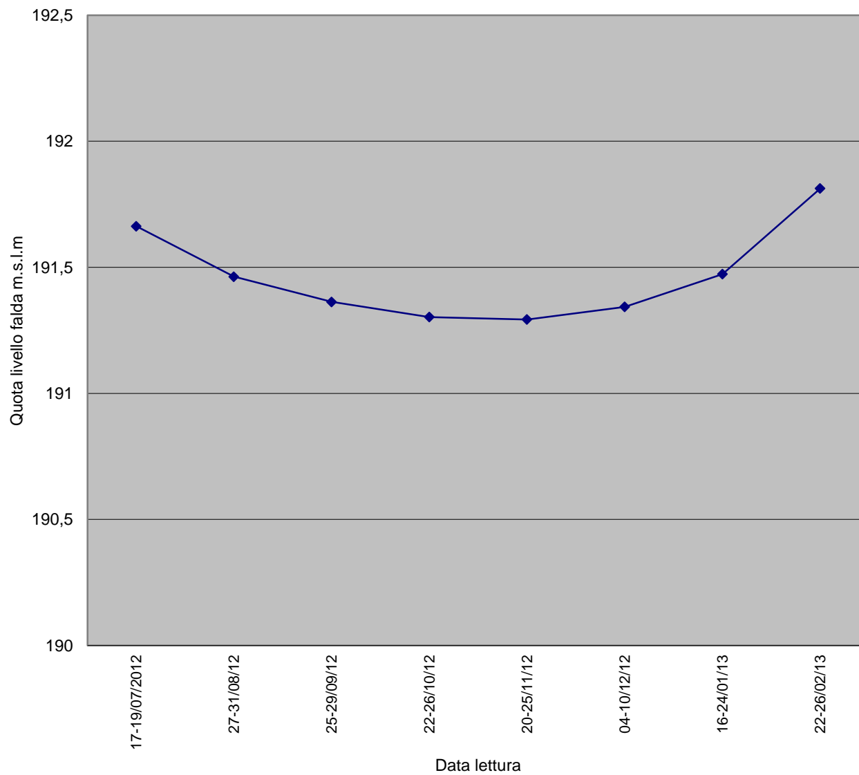
IOV-CH-020 (q.p.c 204,163)
