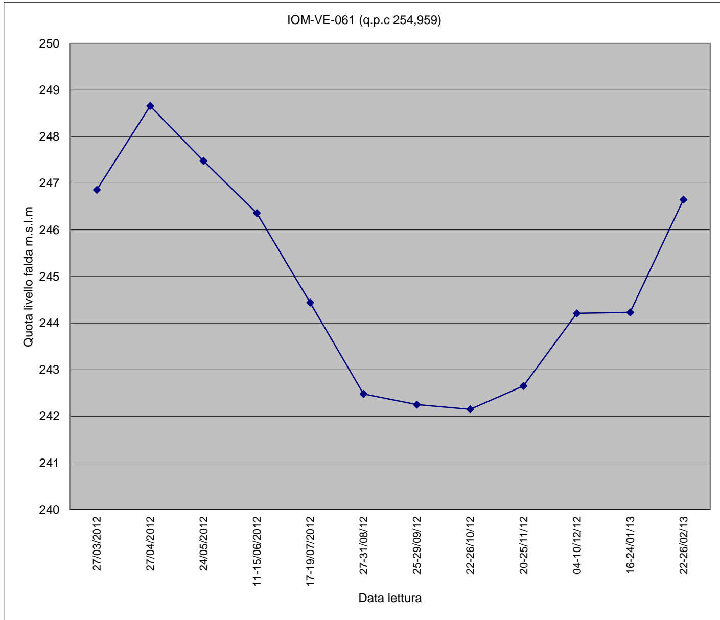
Piezometro IOM-VE-061
