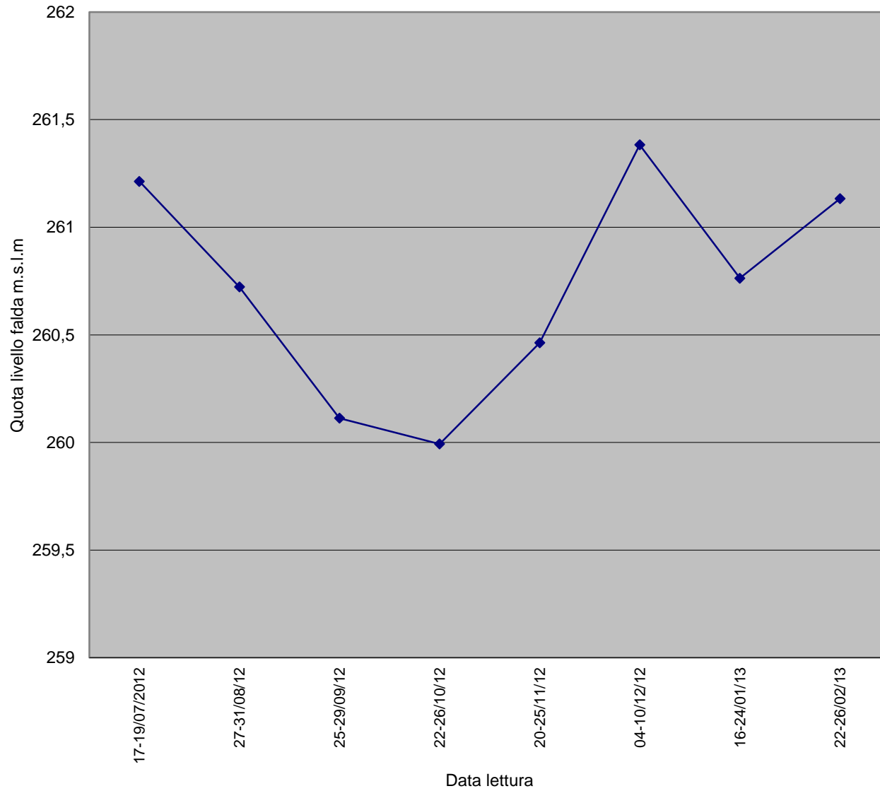
IOM-VE-050bis (q.p.c 266,063)
