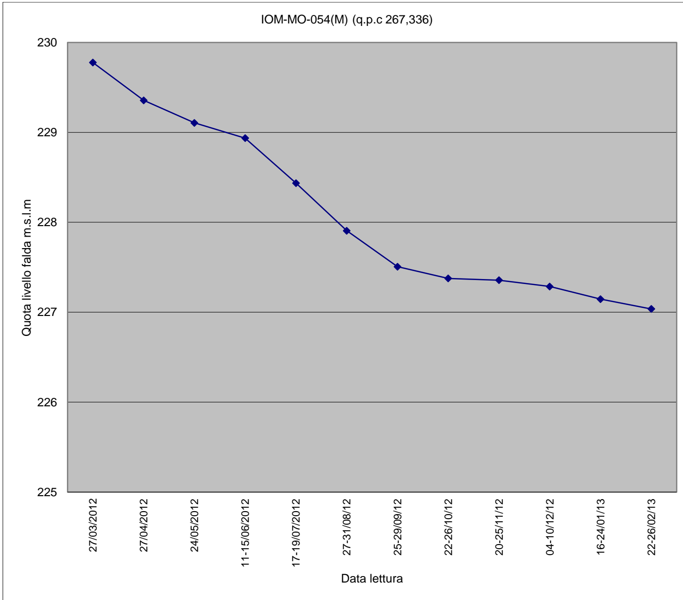
Piezometro IOM-MO-054(M)
