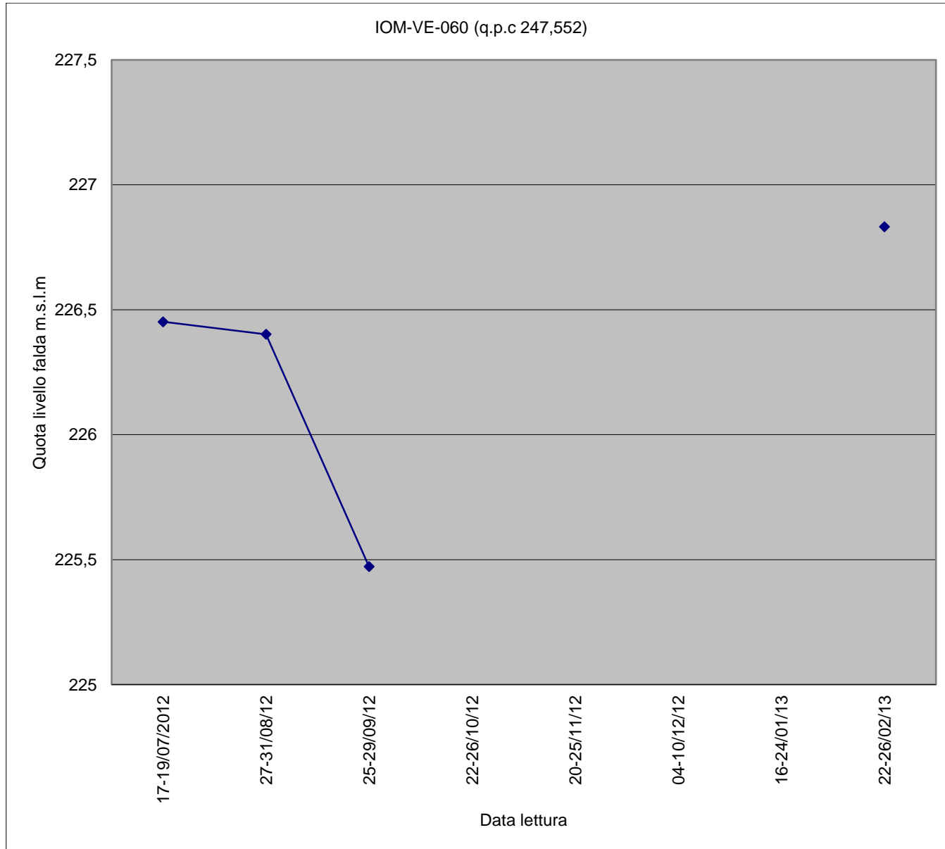
Piezometro IOM-VE-060
