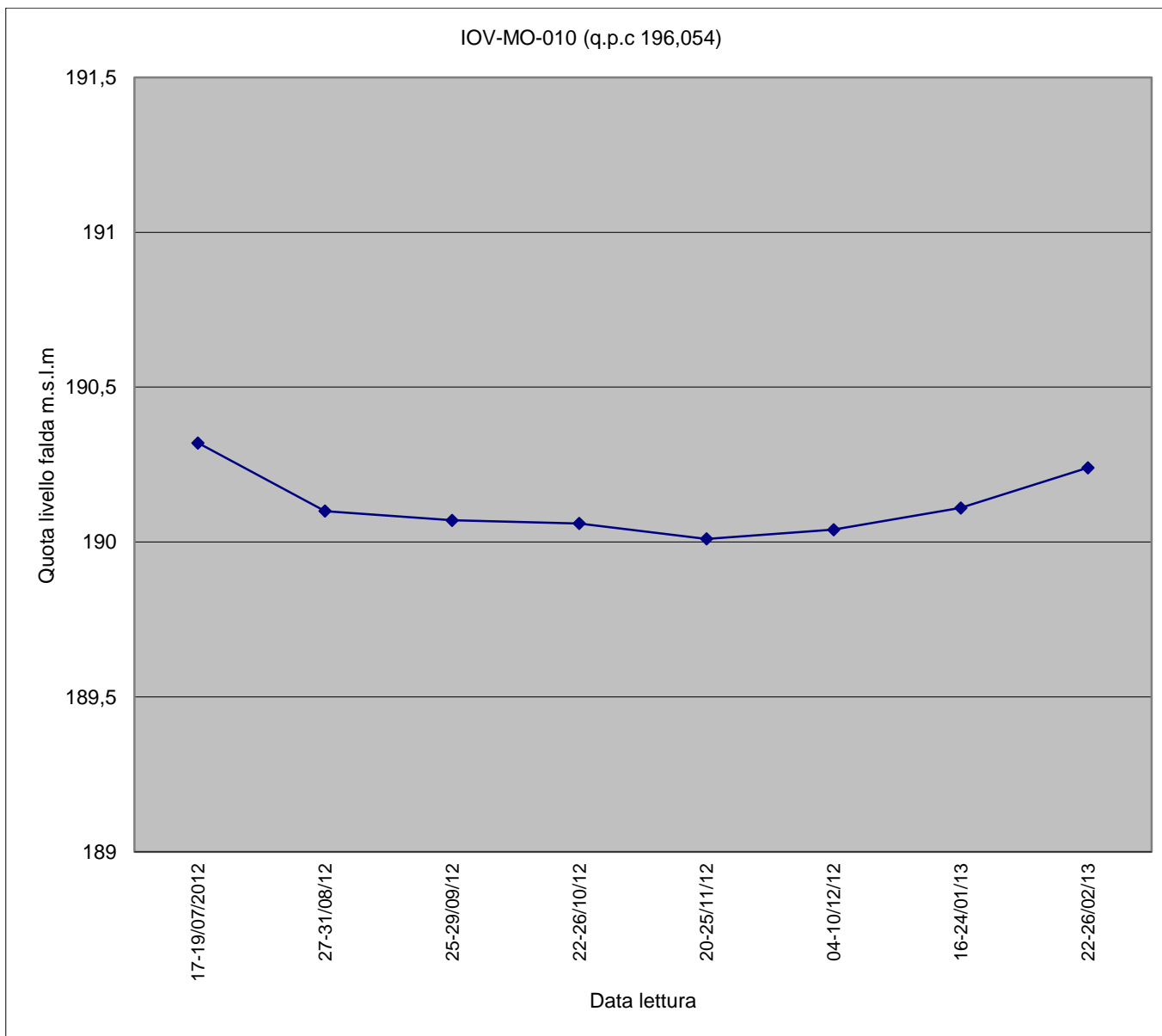
Piezometro IOV-MO-010
