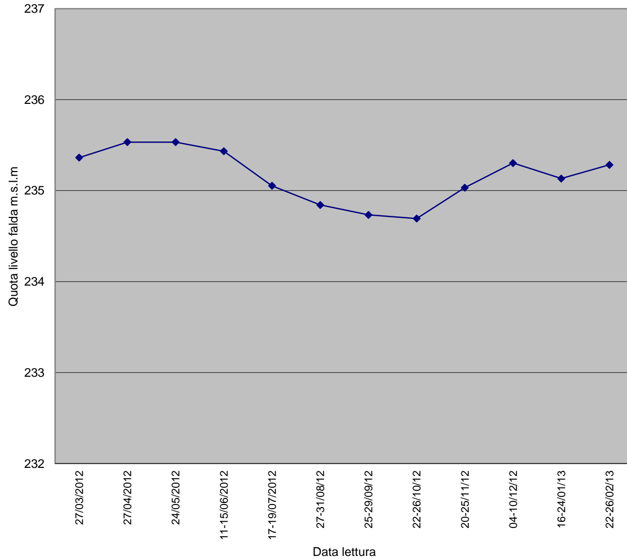
IOV-VE-040(G) (q.p.c 245,033)
