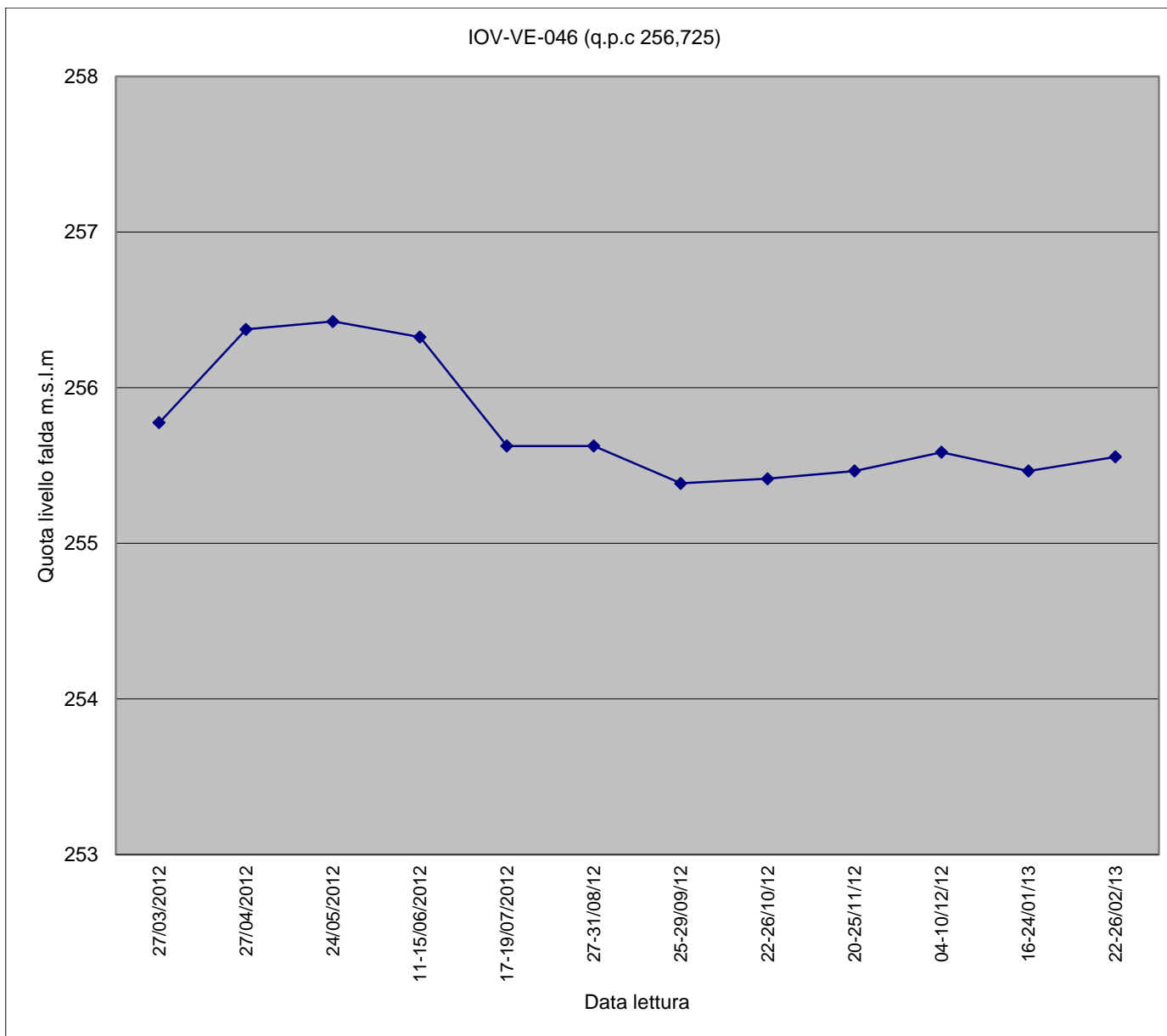
Piezometro IOV-VE-046
