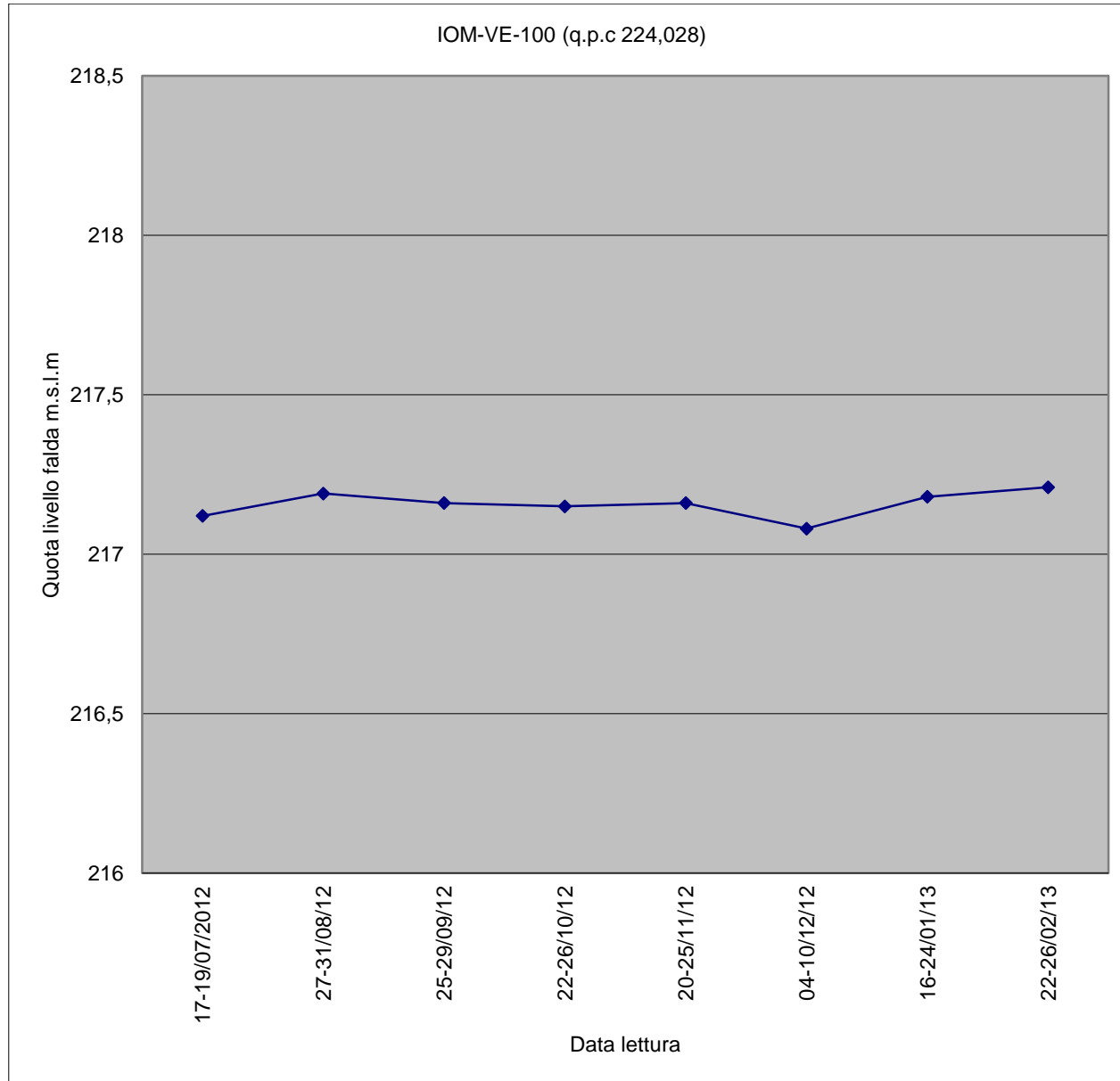
Piezometro IOM-VE-100
