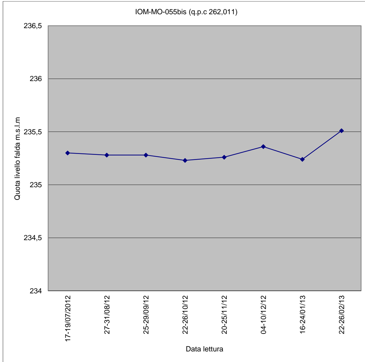
Piezometro IOM-MO-055BIS
