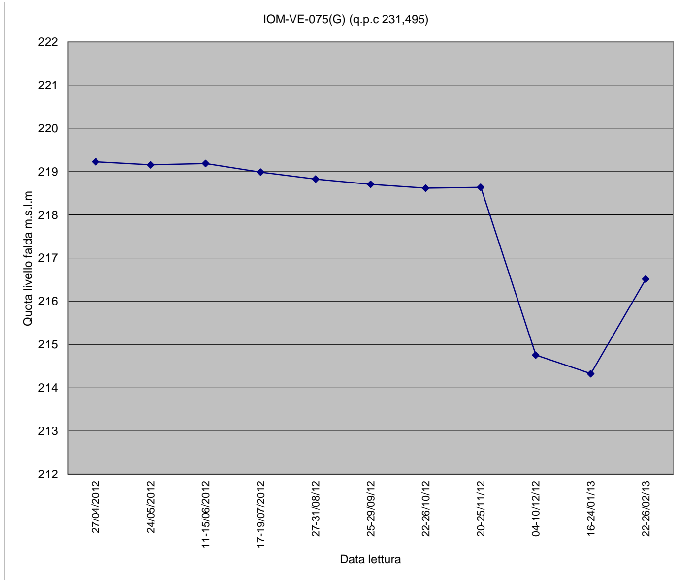
Piezometro IOM-VE-075(g)
