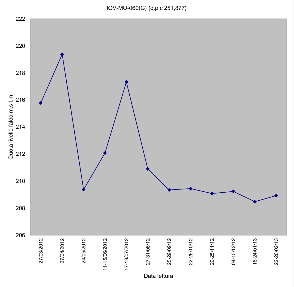
Piezometro IOV-MO-060(G)
