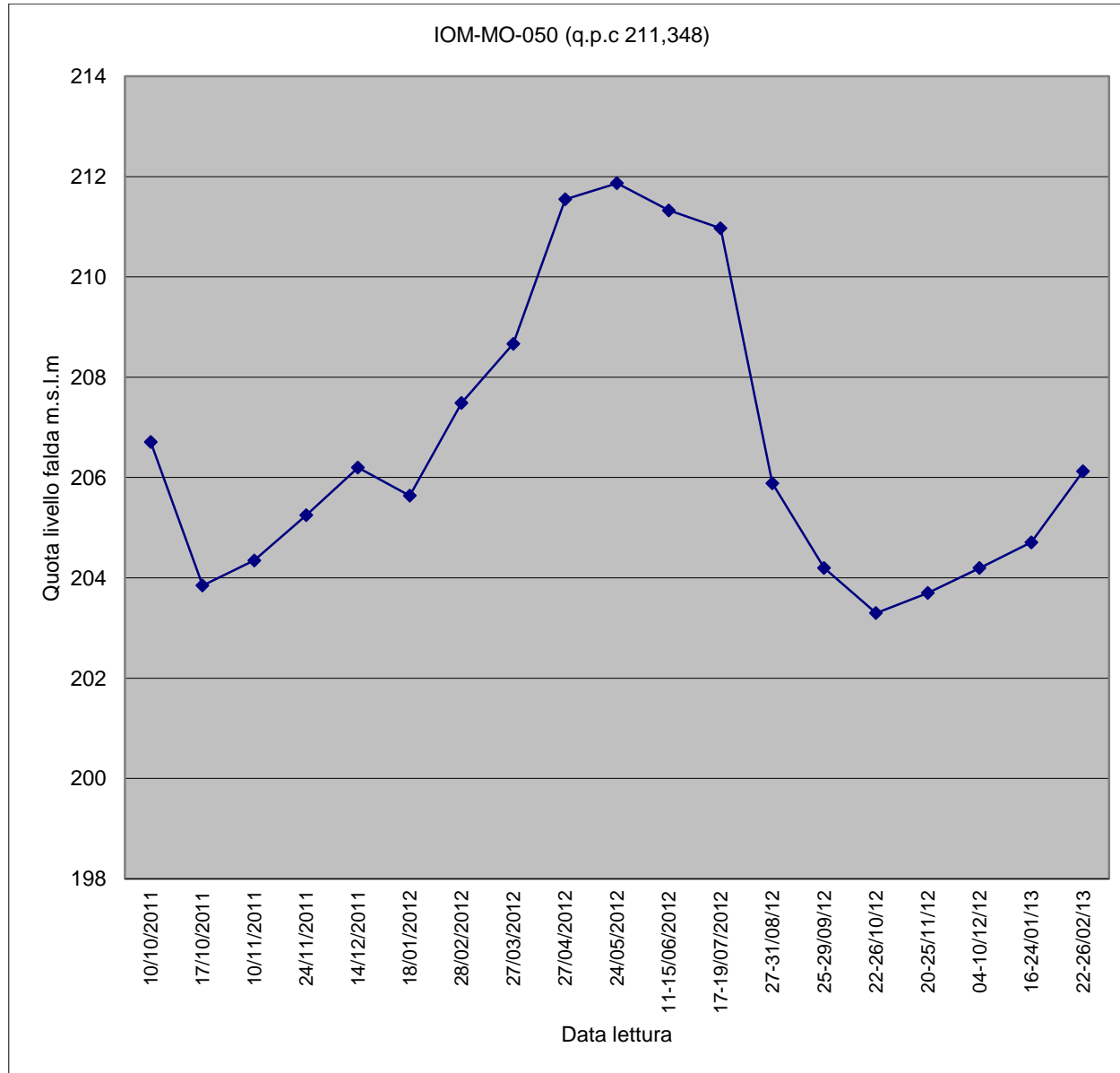
Piezometro IOM-MO-050
