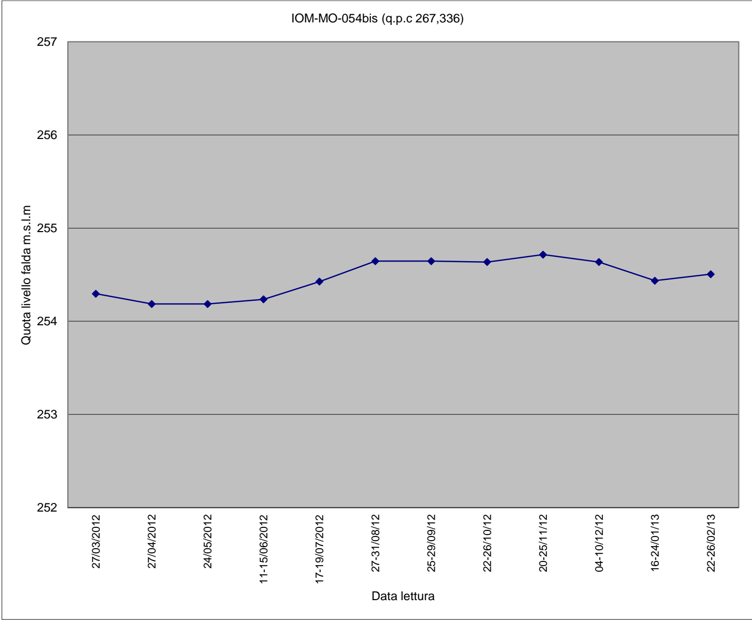
Piezometro IOM-MO-054BIS
