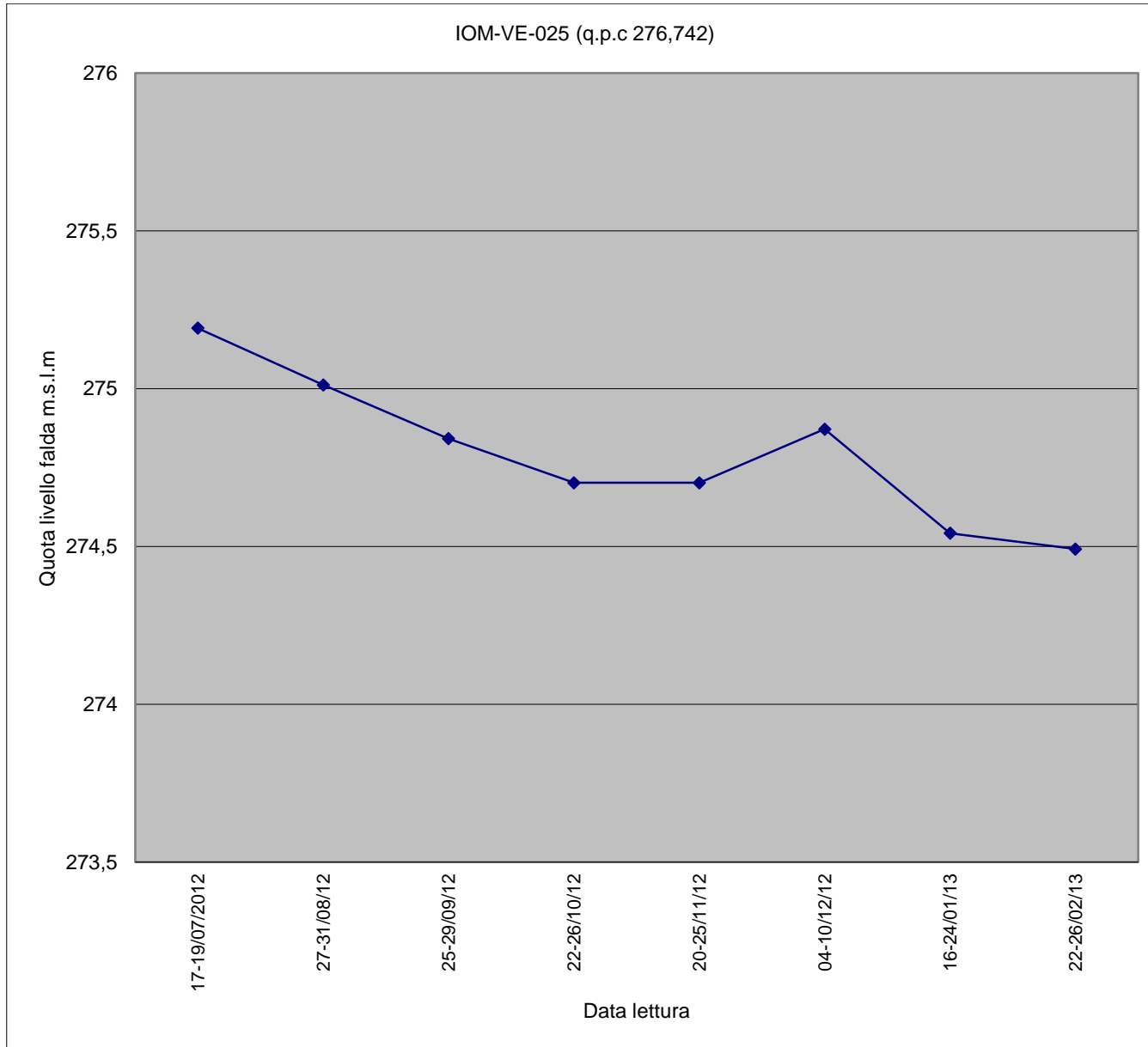
Piezometro IOM-VE-025
