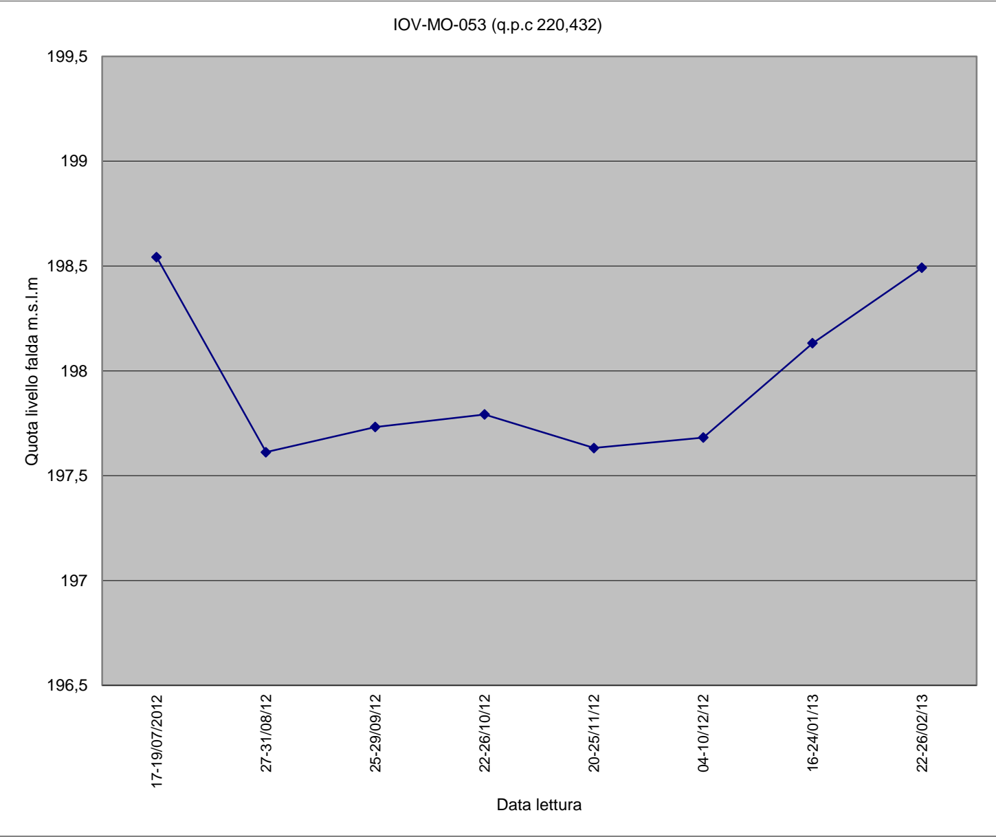
Piezometro IOV-MO-053
