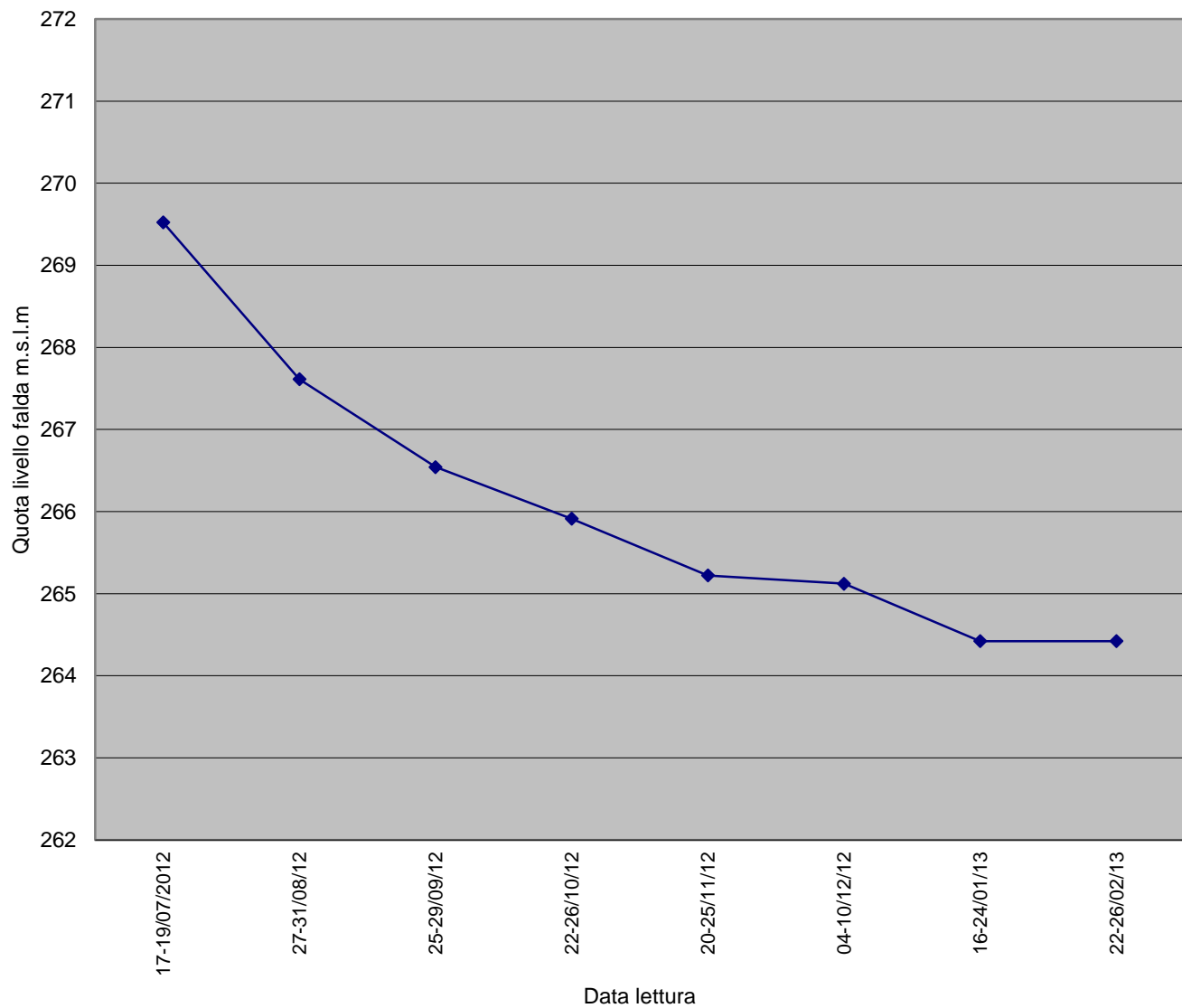
IOM-VE-185 (q.p.c 273,622)
