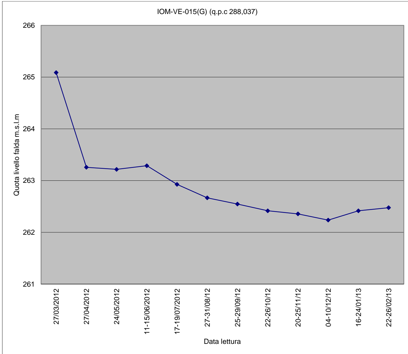
Piezometro IOM-VE-015(G)
