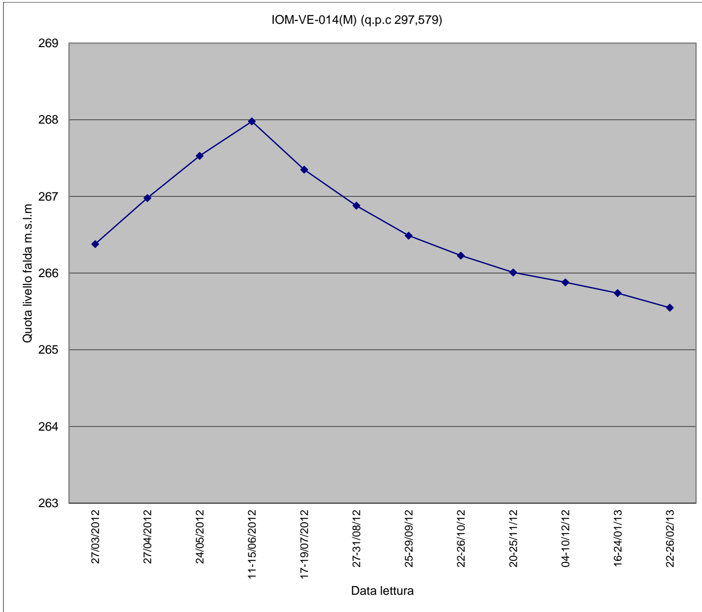
Piezometro IOM-VE-014(M)
