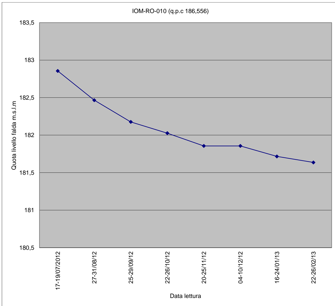
Piezometro IOM-RO-010
