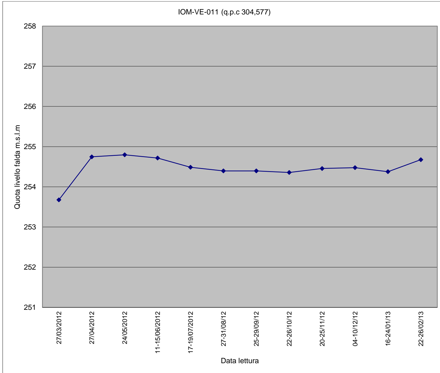
Piezometro IOM-VE-011
