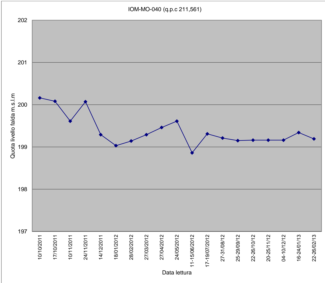
Piezometro IOM-MO-040
