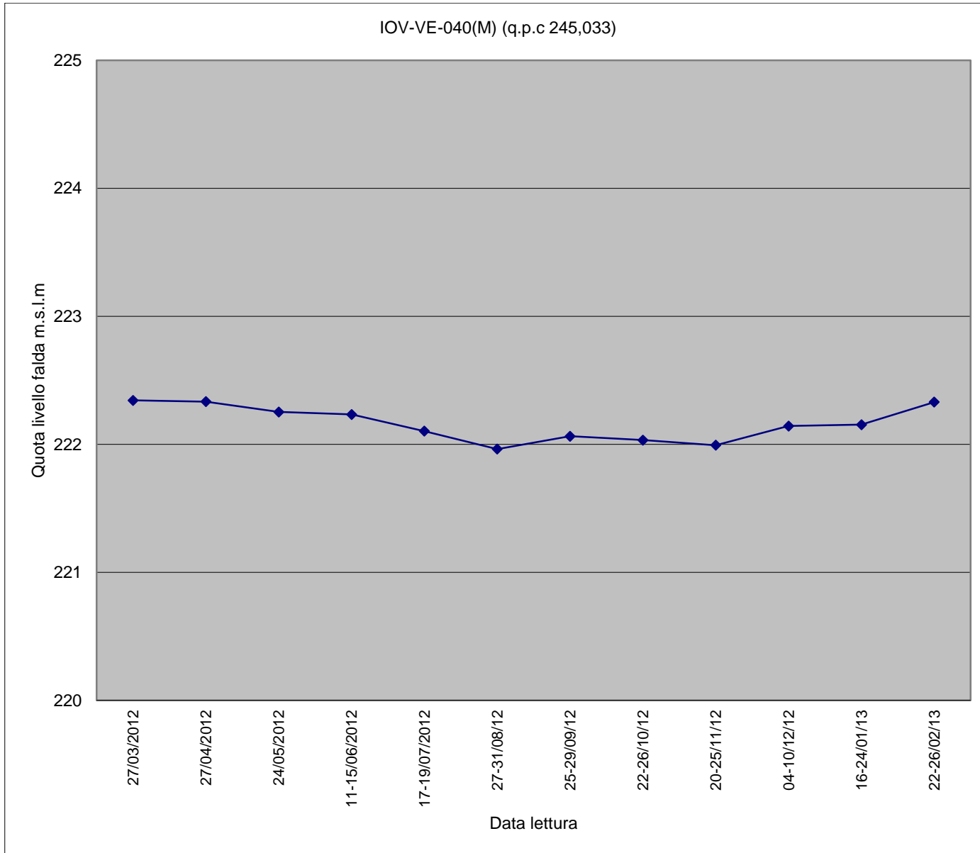
Piezometro IOV-VE-040(M)
