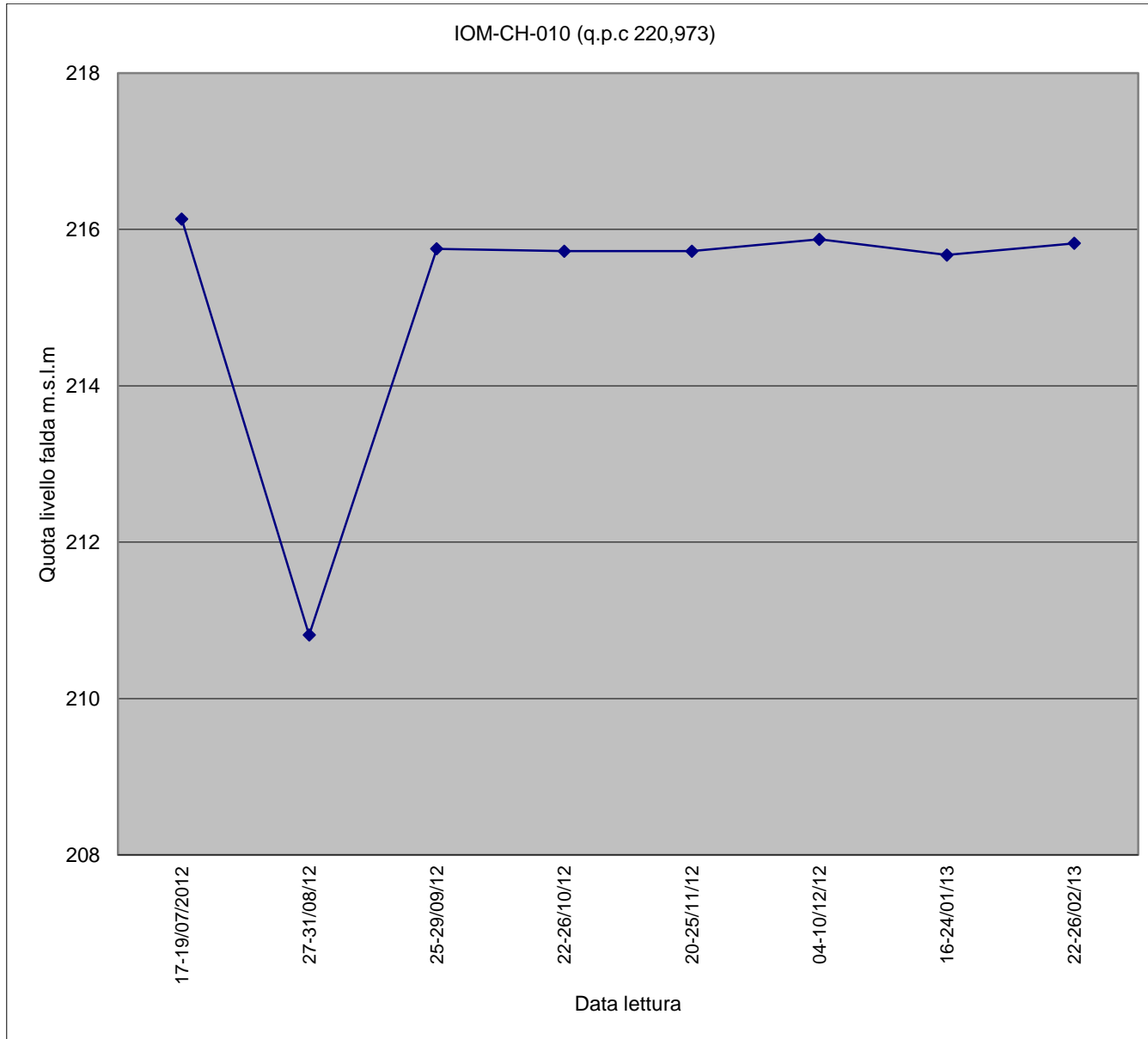
Piezometro IOM-CH-010
