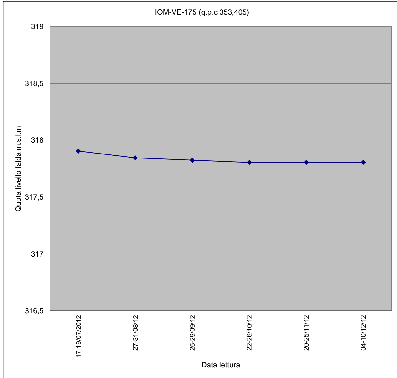
Piezometro IOM-VE-175
