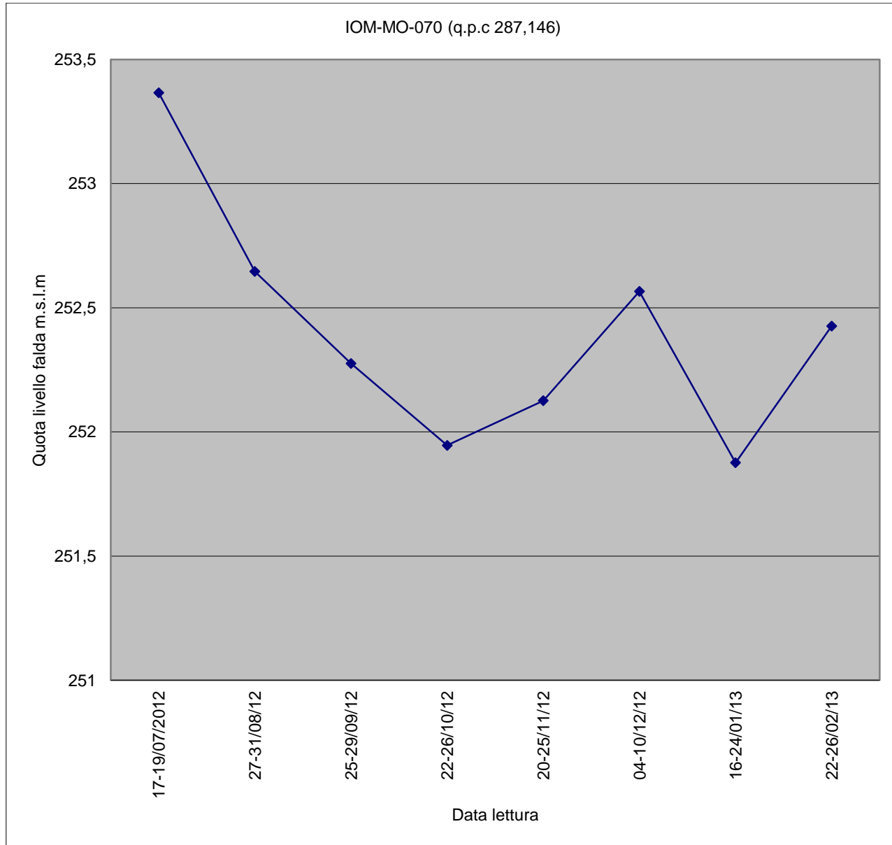
Piezometro IOM-MO-070
