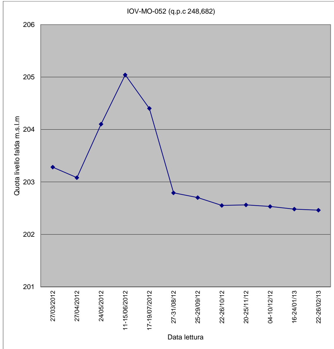
Piezometro IOV-MO-052
