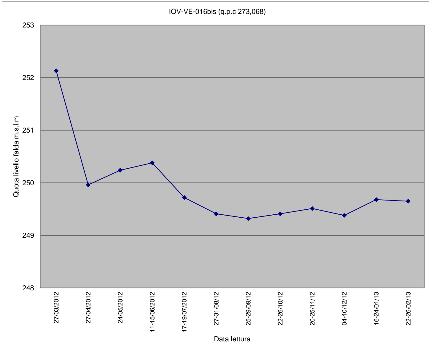
Piezometro IOV-VE-016BIS
