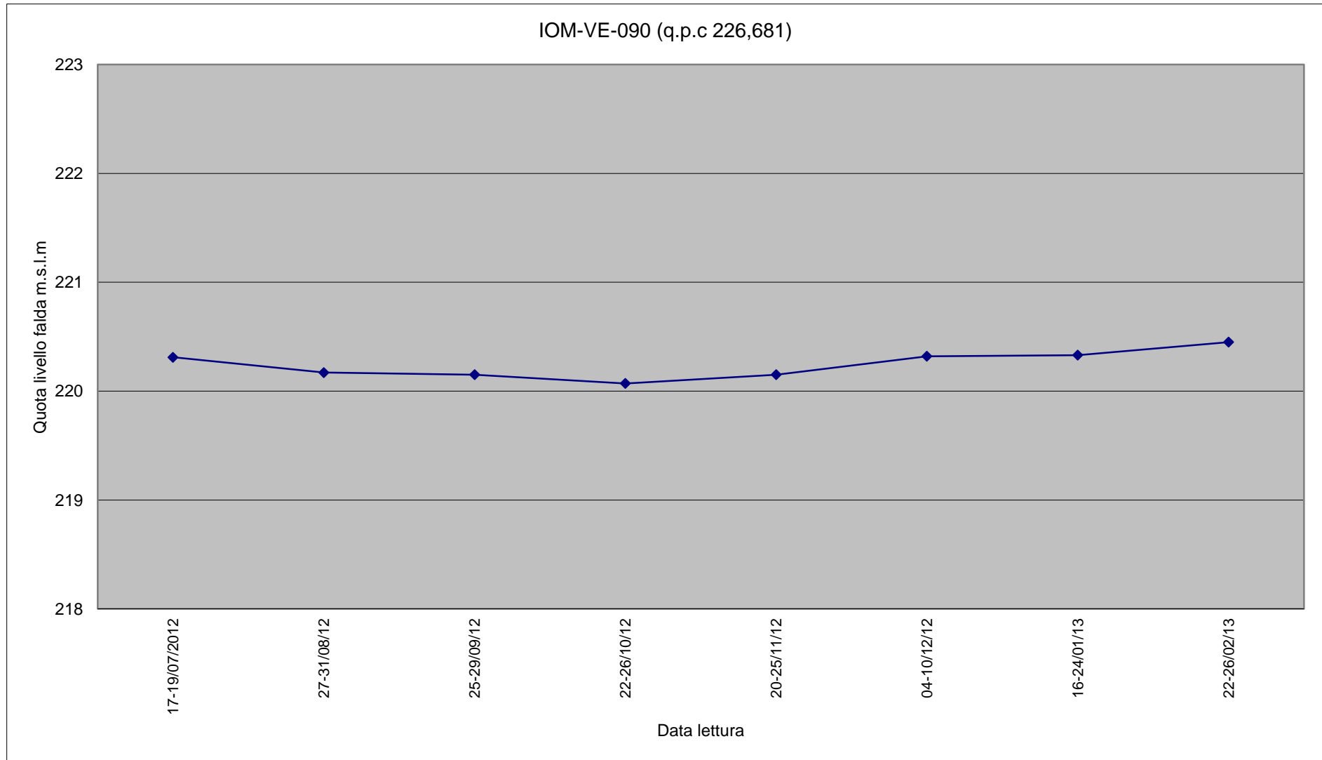
Piezometro IOM-VE-090
