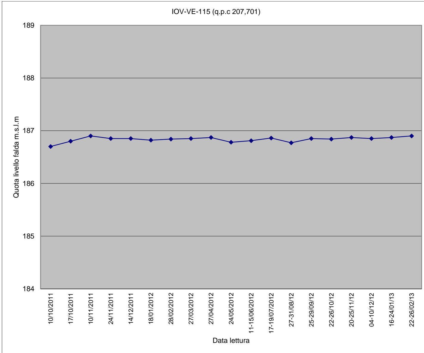
Piezometro IOM-VE-115
