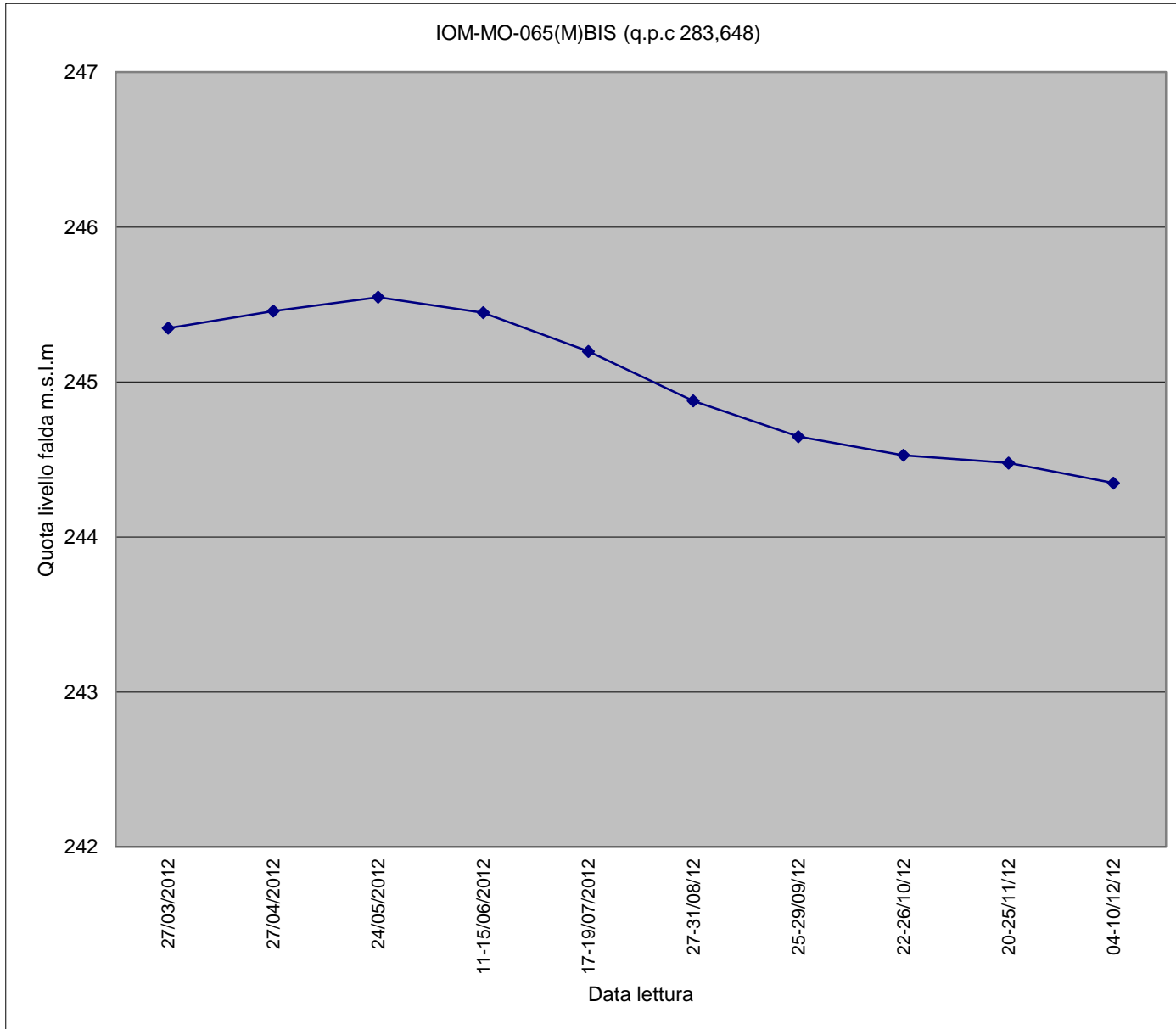
Piezometro IOM-MO-065(M)BIS
