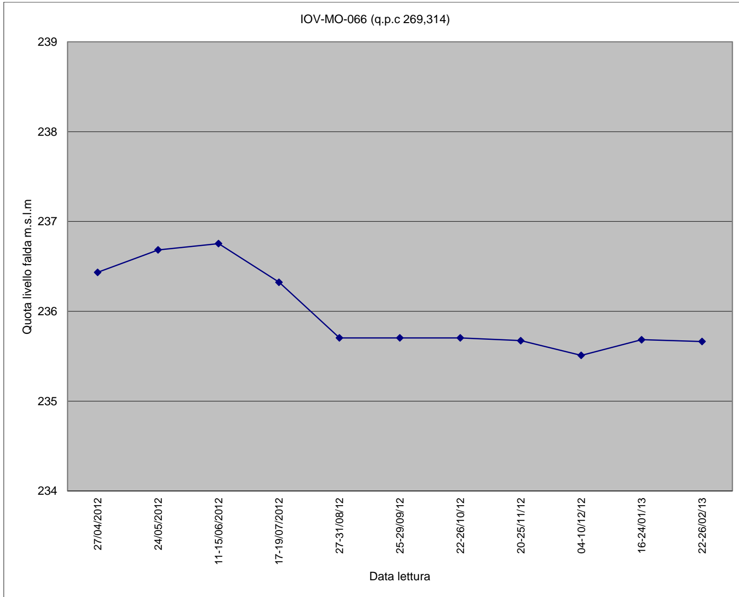
Piezometro IOV-MO-066
