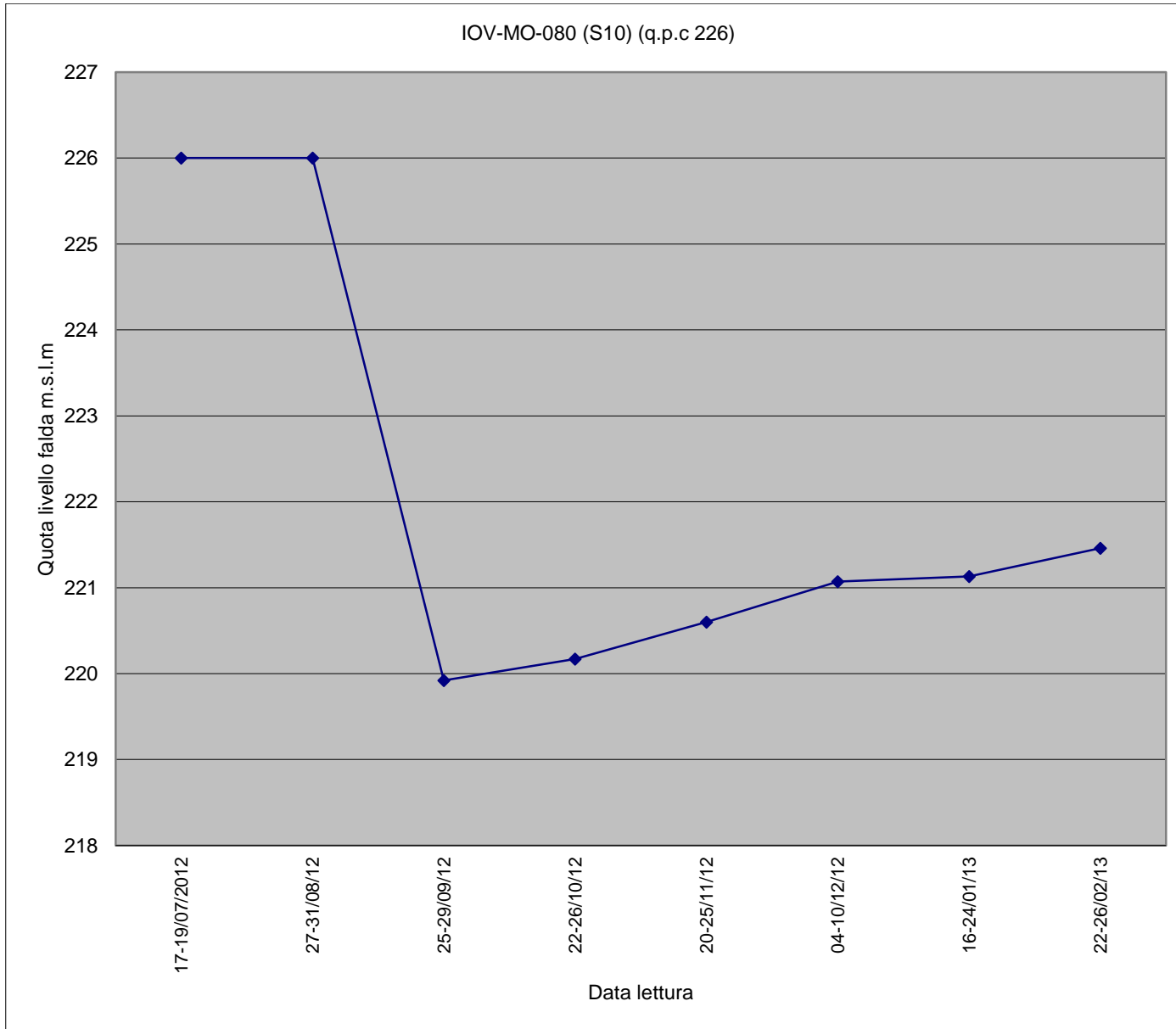
Piezometro IOV-MO-080(S10)
