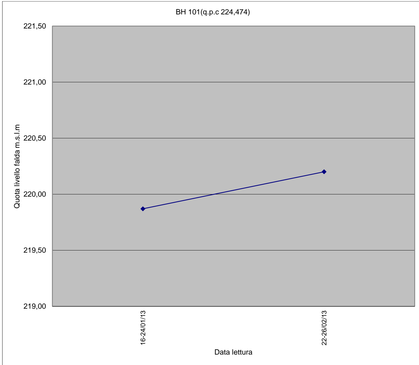
Piezometro BH-101
