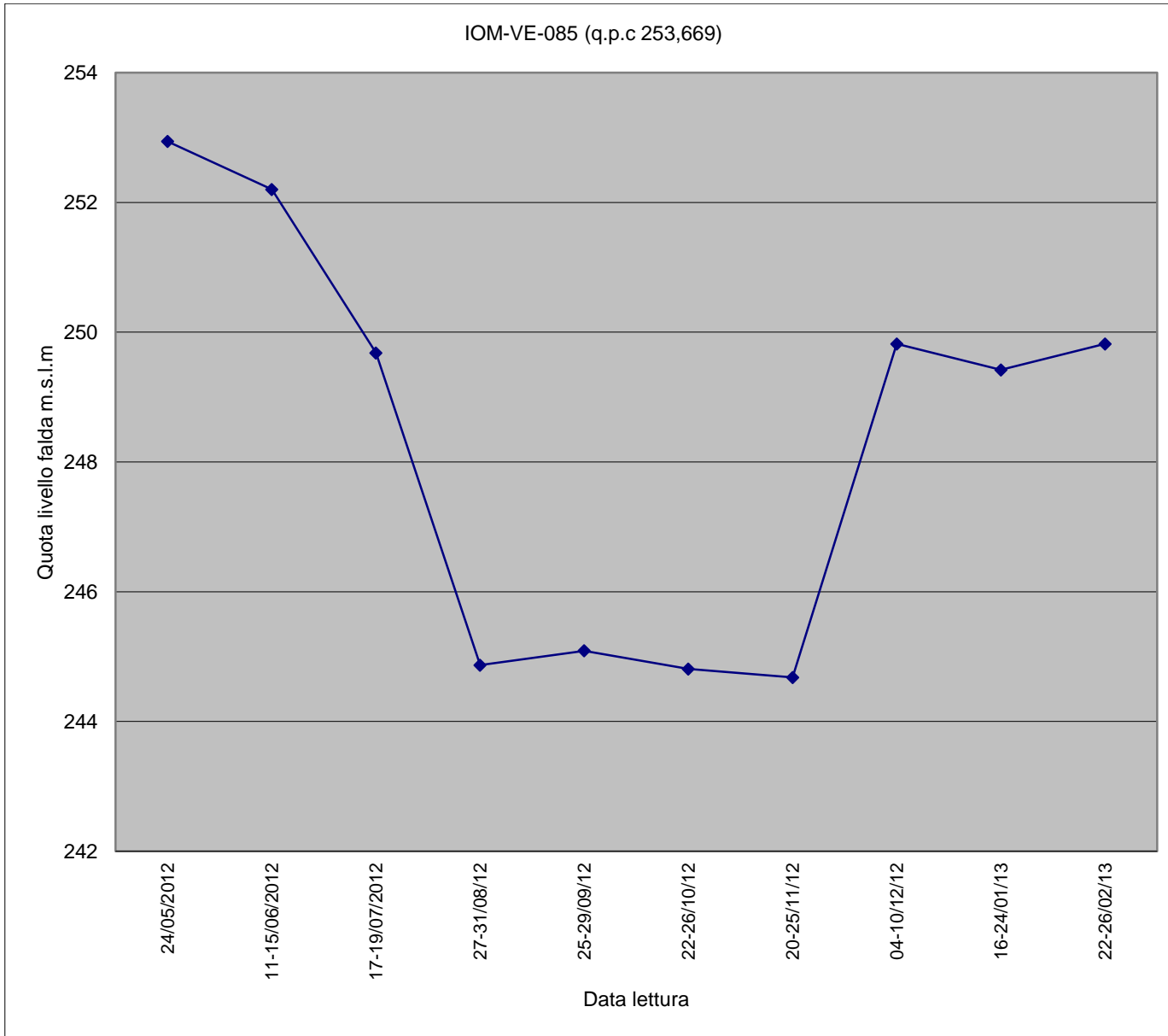
Piezometro IOM-VE-085
