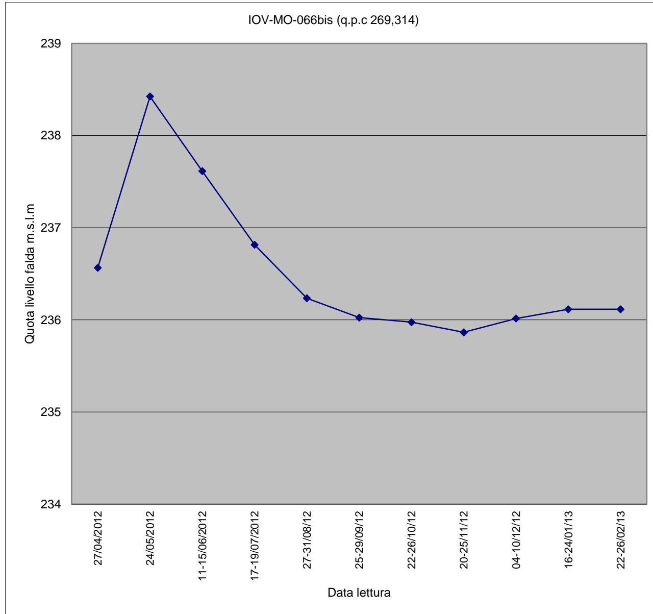
Piezometro IOV-MO-066BIS
