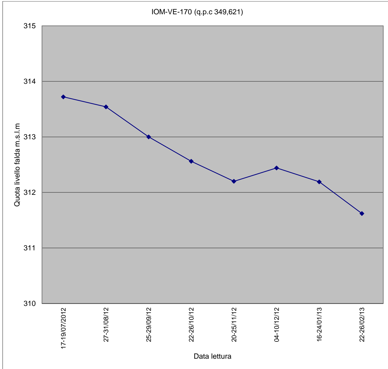
Piezometro IOM-VE-170
