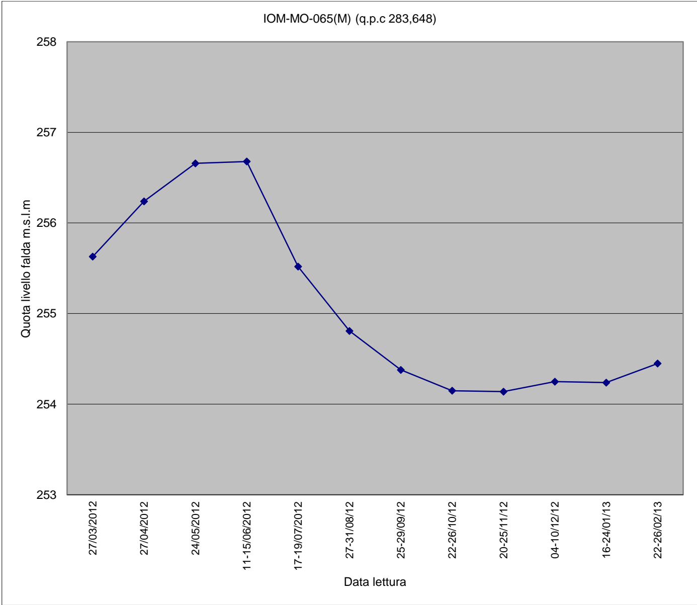
Piezometro IOM-MO-065(M)
