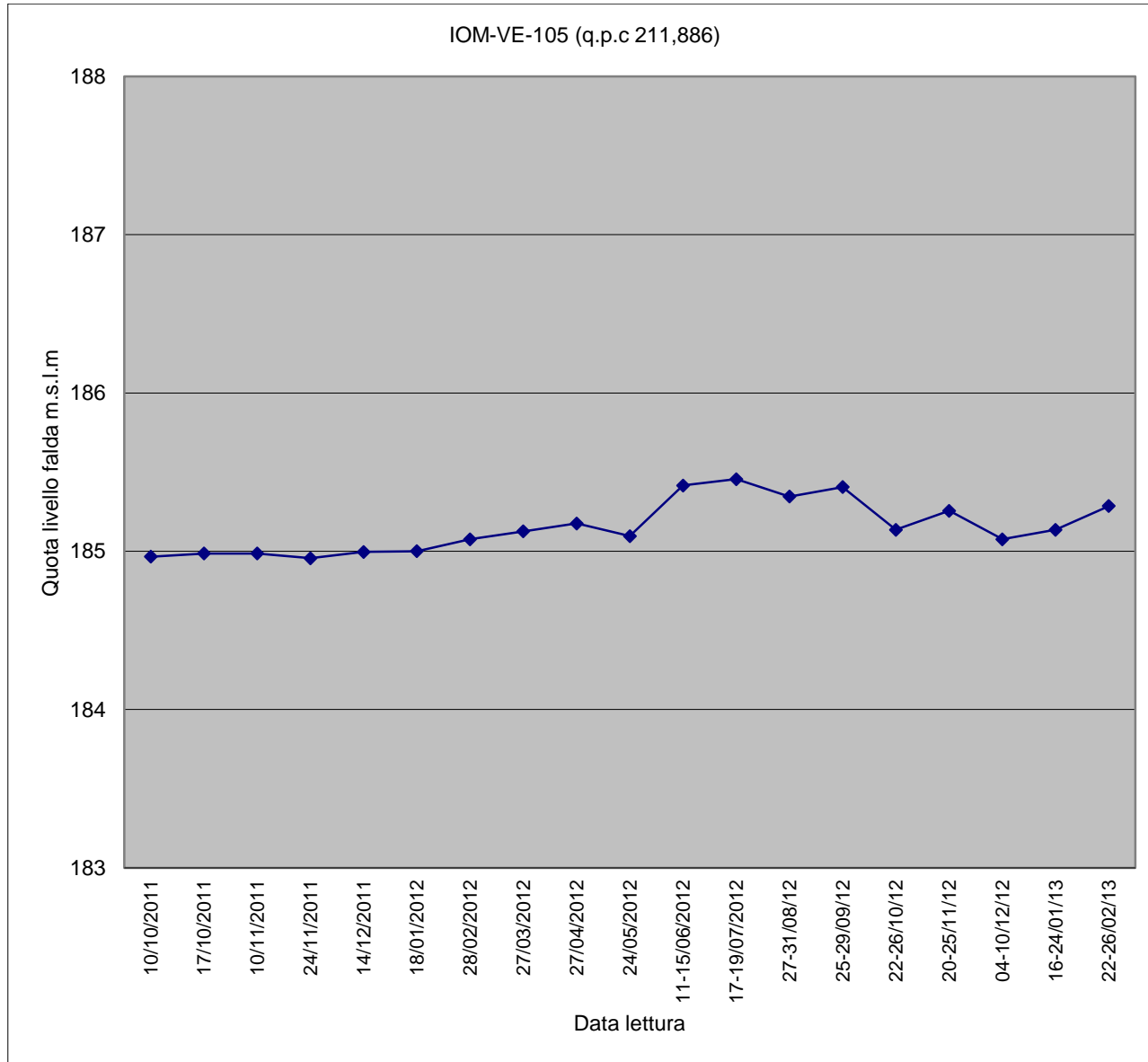
Piezometro IOM-VE-105
