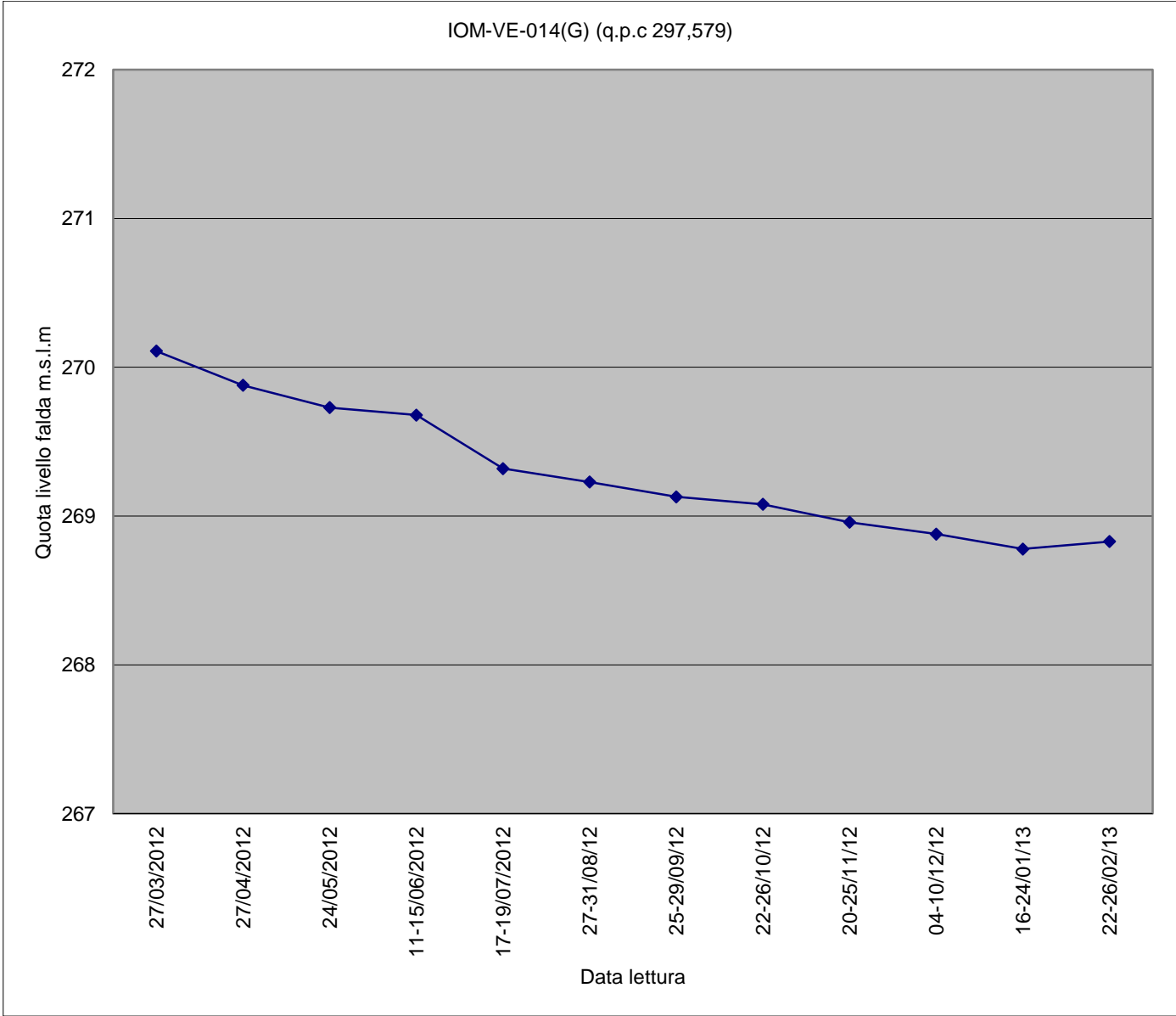
Piezometro IOM-VE-014(G)
