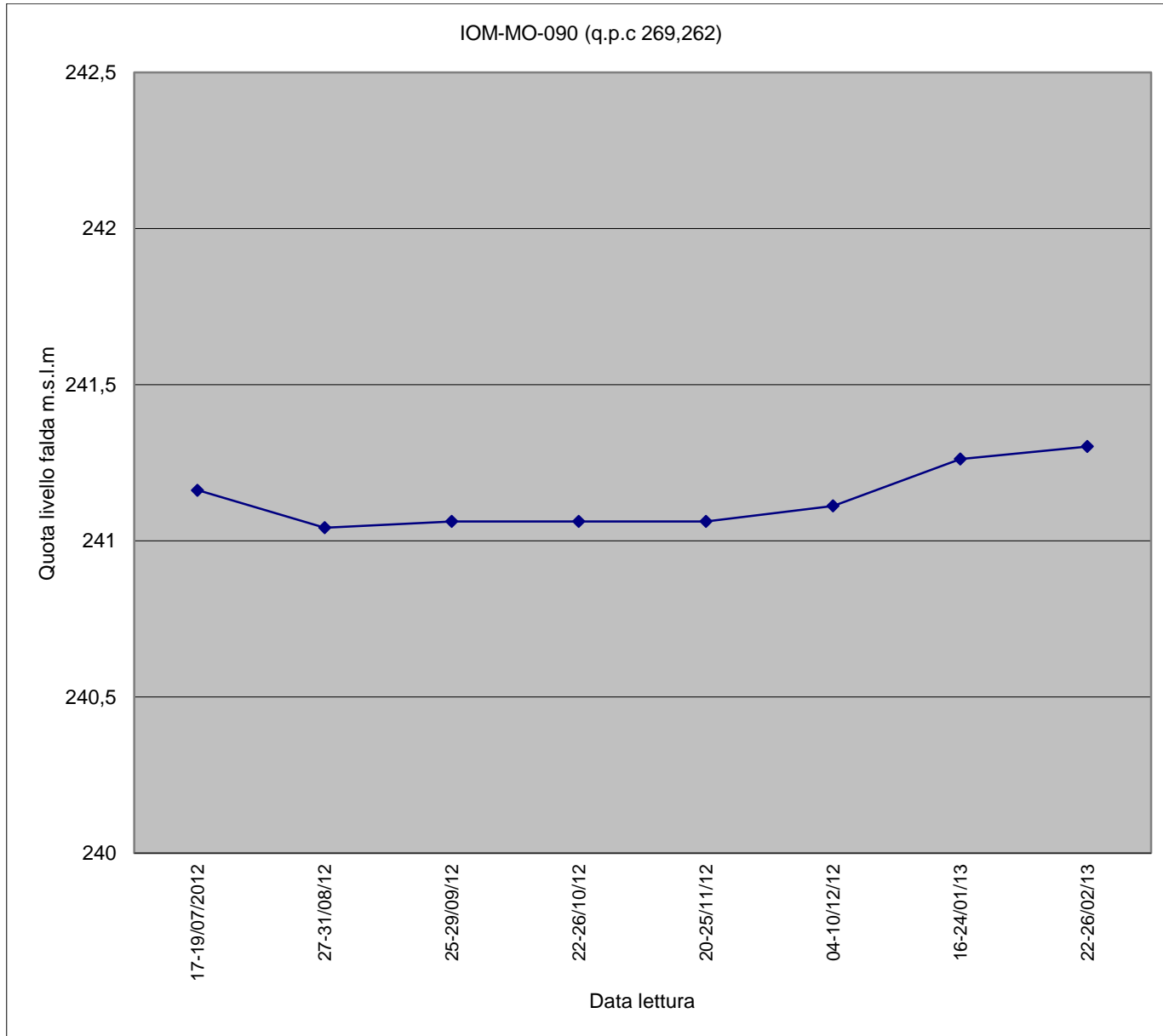
Piezometro IOM-MO-090
