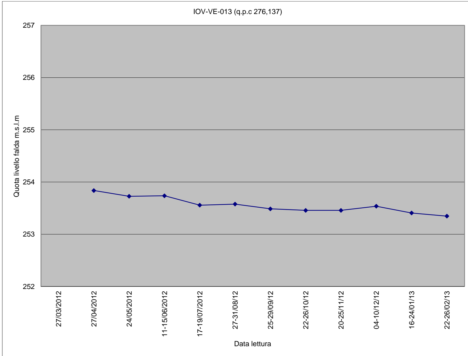
Piezometro IOV-VE-013
