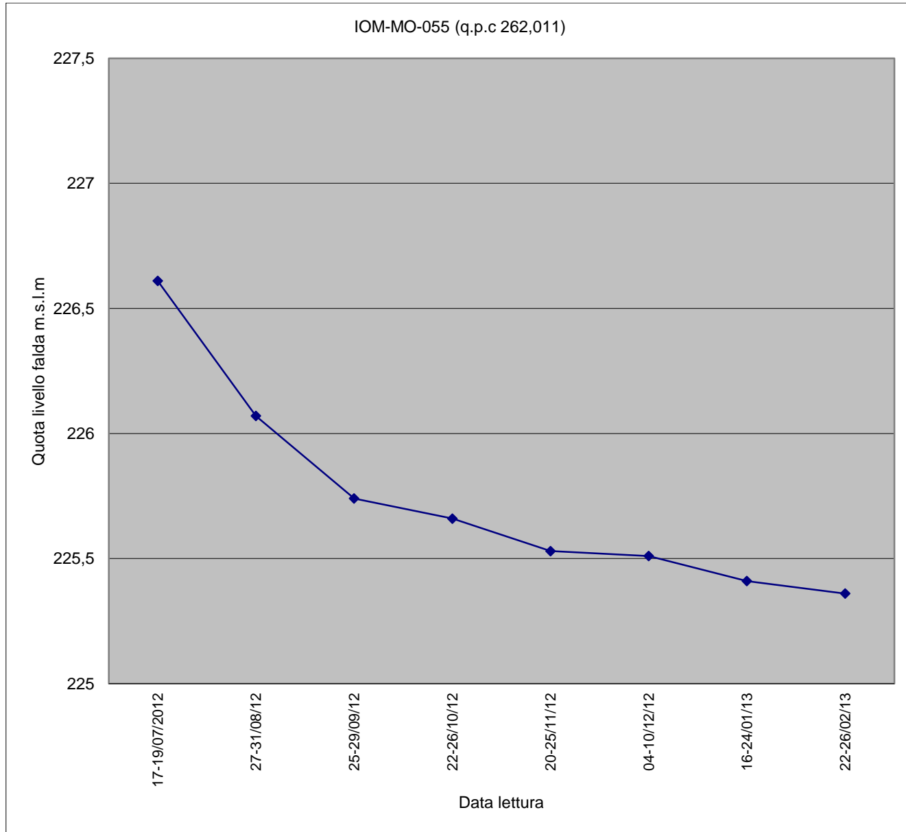
Piezometro IOM-MO-055
