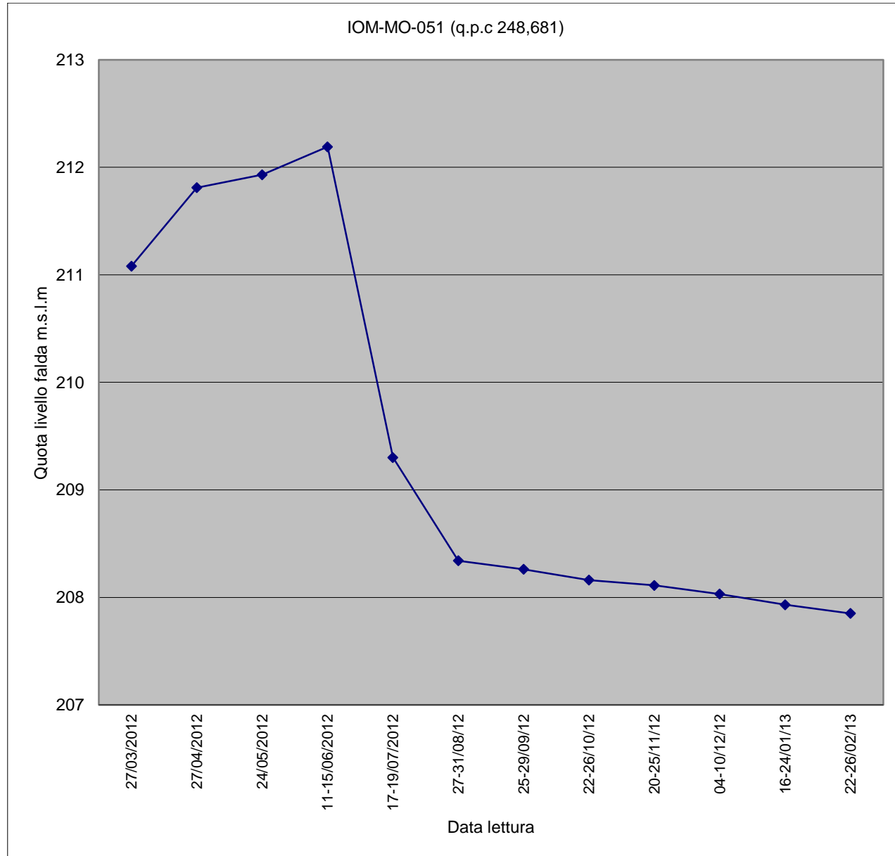
Piezometro IOM-MO-051
