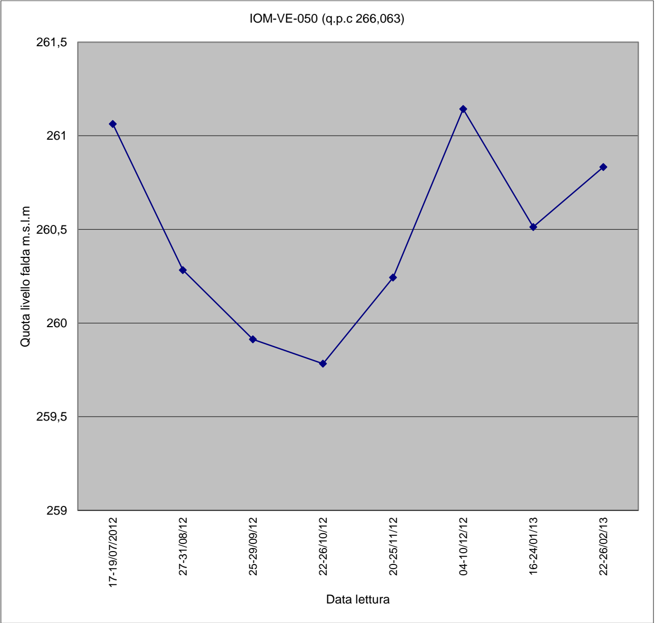
Piezometro IOM-VE-050
