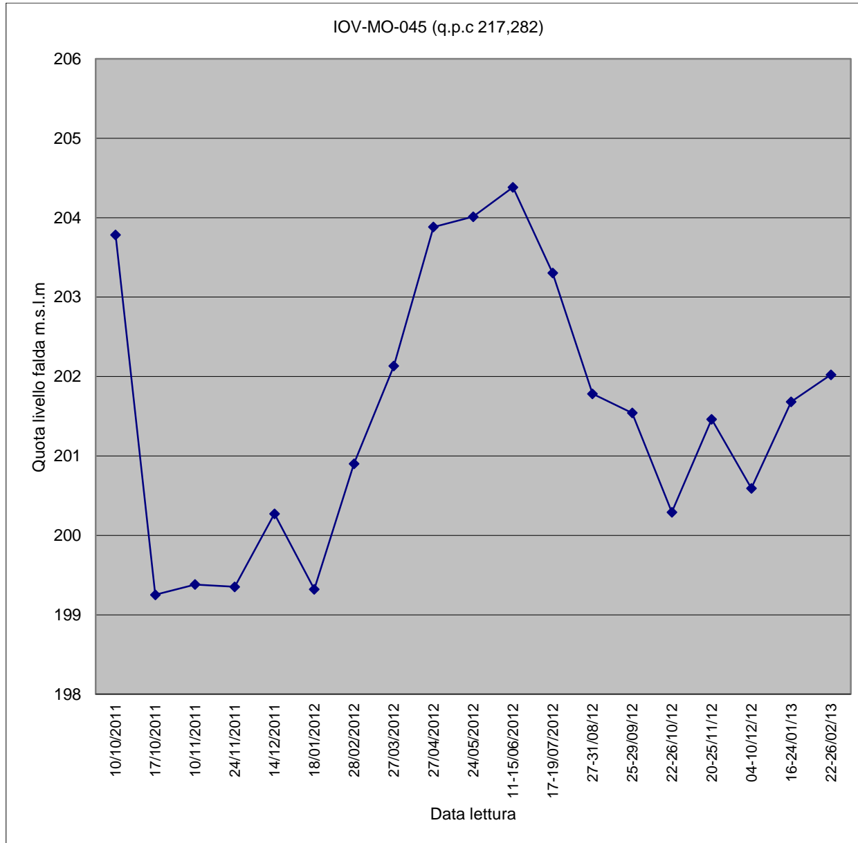
Piezometro IOV-MO-045
