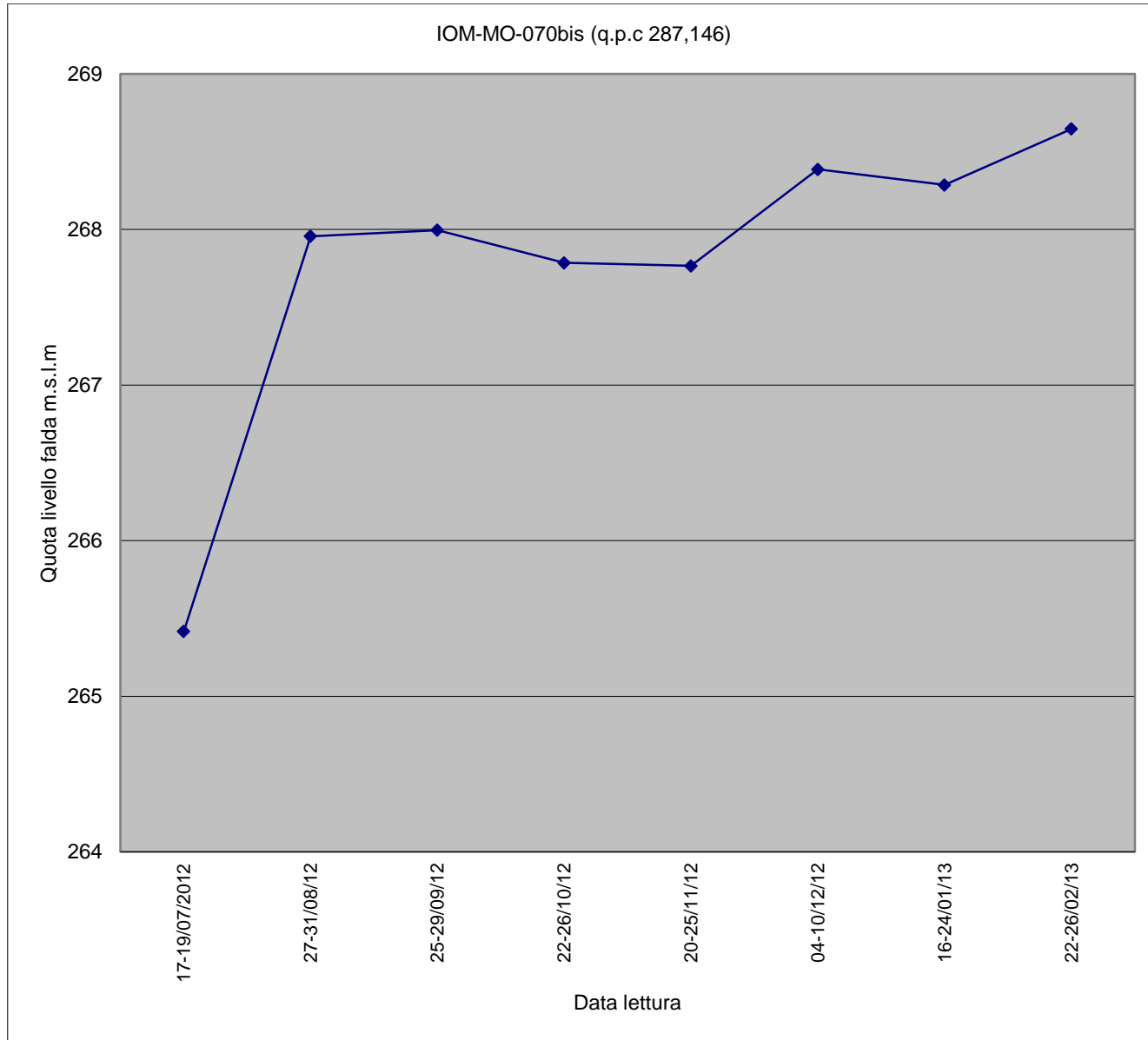
Piezometro IOM-MO-070BIS
