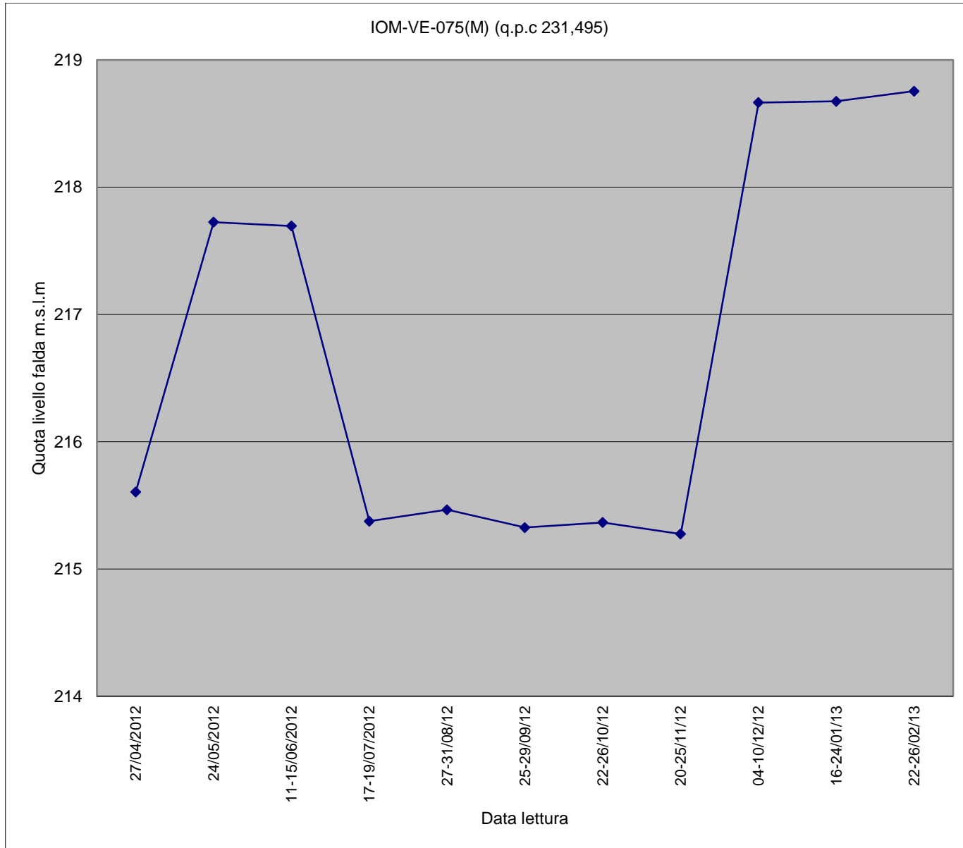
Piezometro IOM-VE-075(M)
