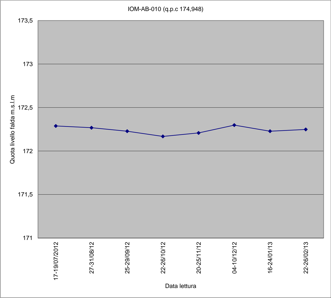
Piezometro IOM-AB-010
