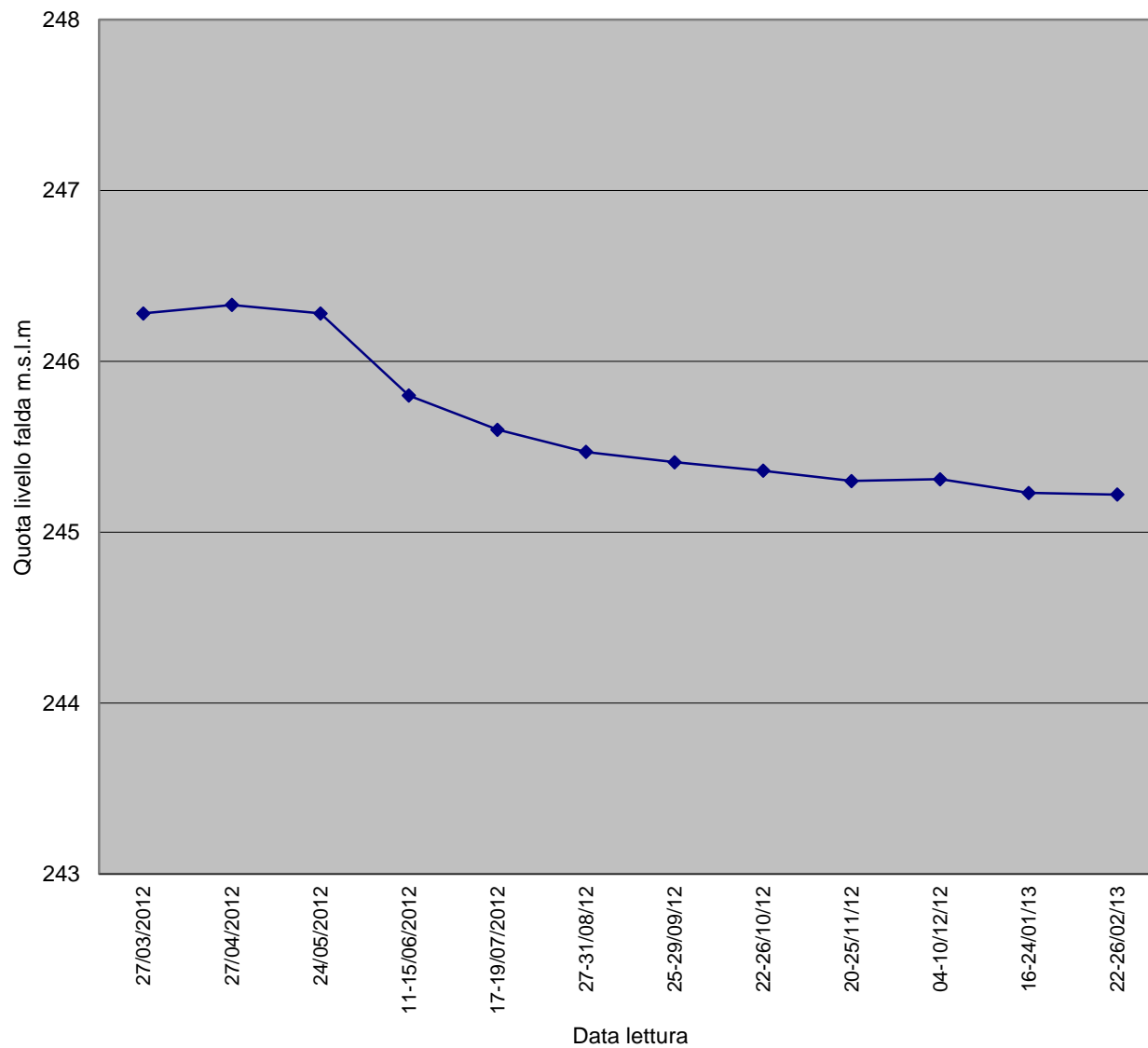
IOV-VE-016 (q.p.c 273,068)
