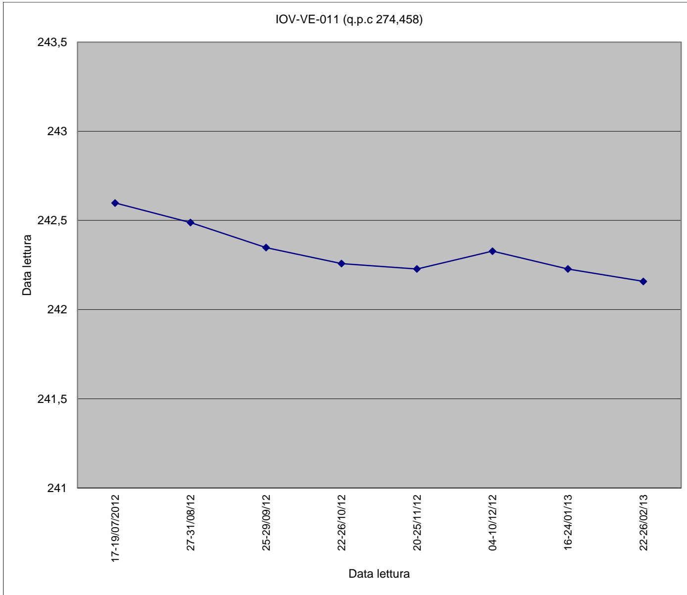
Piezometro IOV-VE-011
