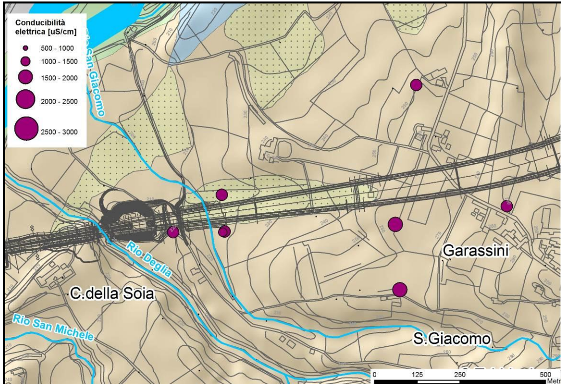
Figura 19. Distribuzione delle conducibilità elettriche medie dell'acqua di falda dalle misure dei piezometri fenestrati nei gessi.
