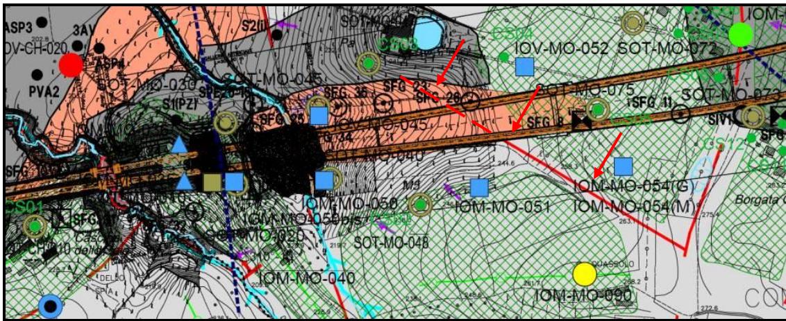
Figura 24. Ubicazione in carta della presunta faglia NW-SE lungo la quale è stato ipotizzata la presenza di un salto piezometrico.
