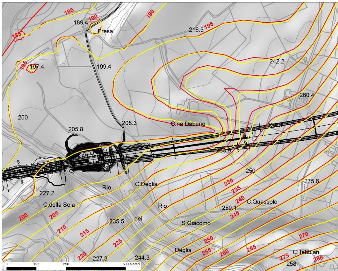
Figura 47. Confronto tra distribuzione piezometrica allo stato naturale (linee rosse) e in una situazione in cui la falda raggiunge una condizione di stabilizzazione dopo la messa in opera del cunicolo e delle due canne (linee gialle).
