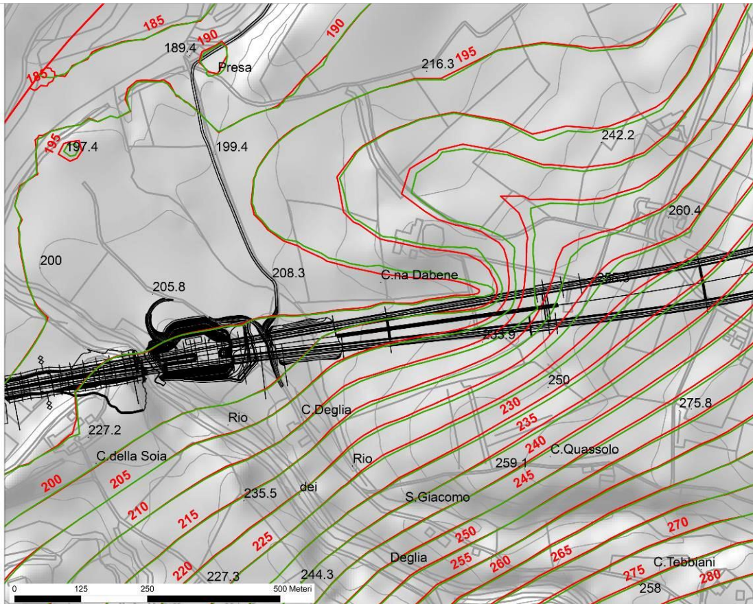
Figura 45. Confronto tra distribuzione piezometrica allo stato naturale (linee rosse) e in una situazione in cui il drenaggio del cunicolo centrale ha raggiunto una stabilizzazione dopo 1 anno dalla fine dello scavo all'interno dell'acquifero dei gessi (linee verdi).
