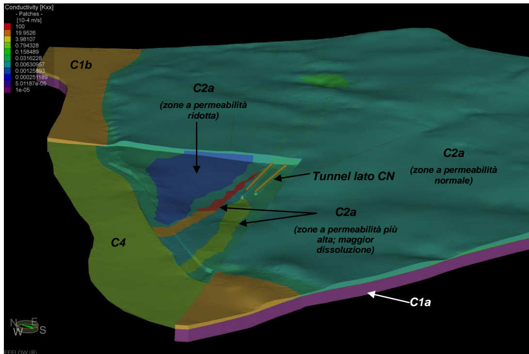
Figura 42. Distribuzione delle conducibilità idrauliche utilizzate per una calibrazione ottimale del modello numerico; C1a, C1b, C2a, C4 = complessi idrogeologici 1a, 1b, 2a e 4
