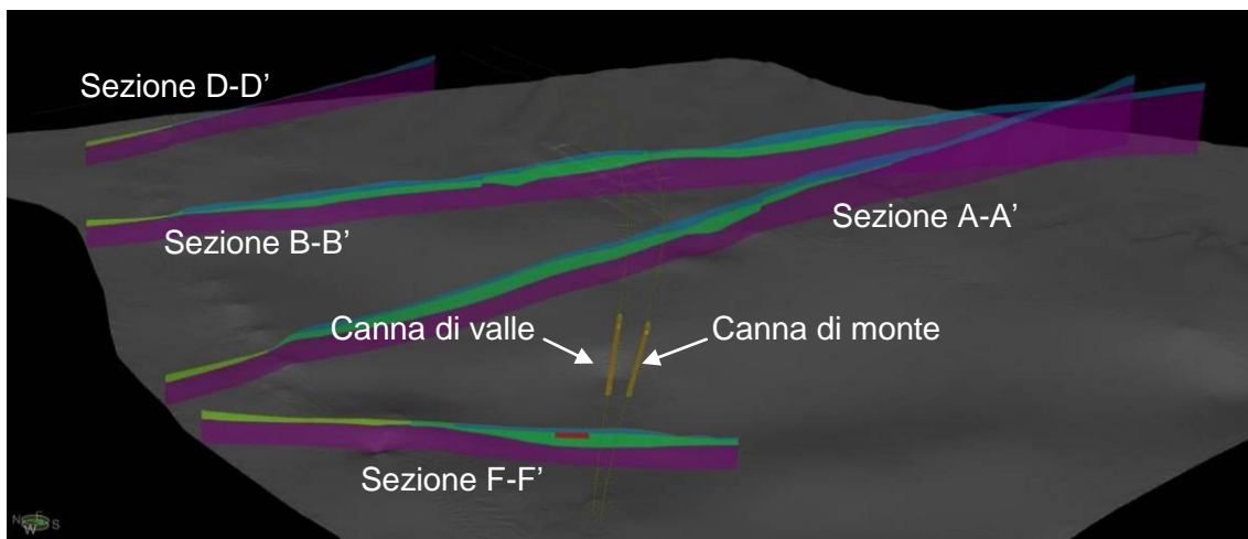
Figura 39. Visualizzazione delle sezioni trasversali al tracciato della galleria attraverso la ricostruzione geometrica dei corpi di Feflow.
