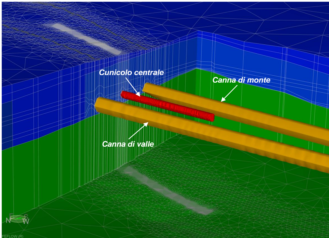
Figura 40. Dettaglio delle due canne del tunnel utilizzate e del cunicolo centrale, con spaccato utile per comprendere le geometrie interne dei layer con cui è stato costruito il modello numerico.
