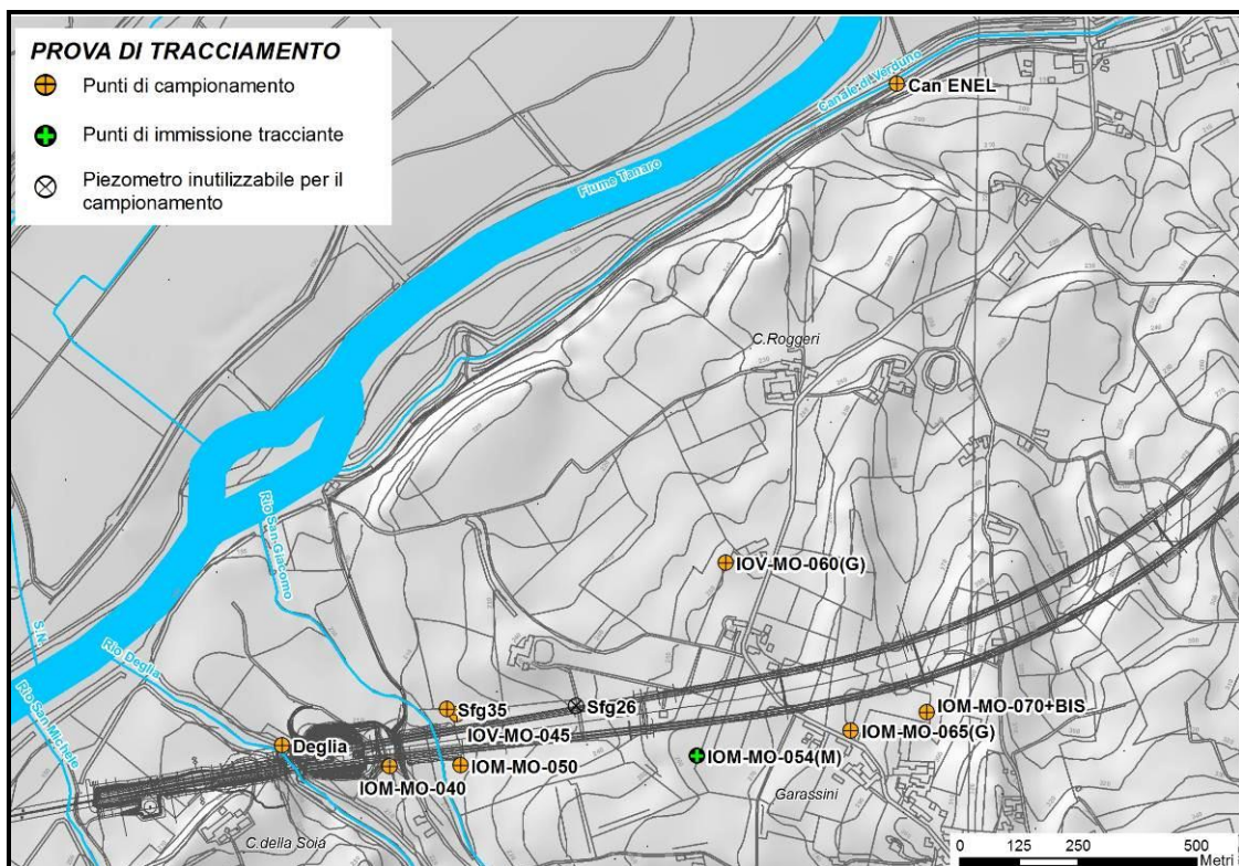
Figura 31. Ubicazione in carta del punto di immissione della fluoresceina e dei punti di campionamento.
