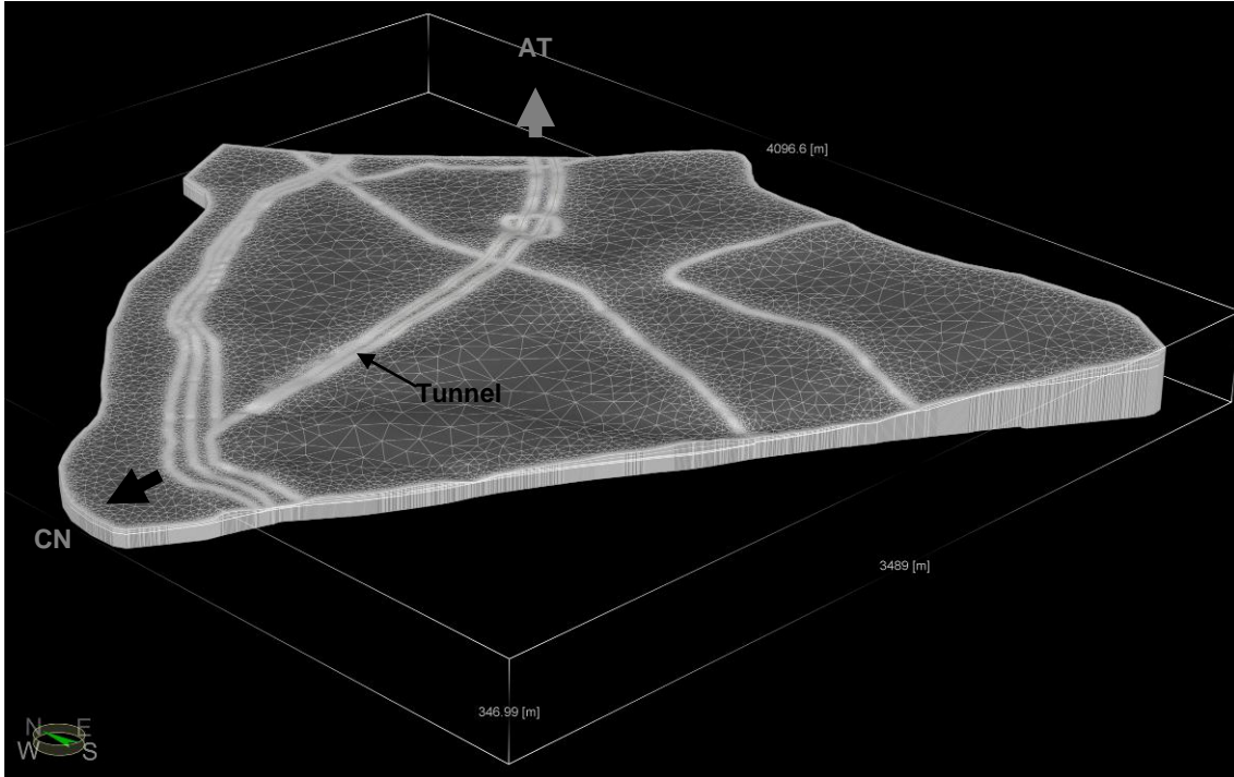
Figura 37. Visualizzazione 3D della geometria e degli elementi finiti con punto vista dall'imbocco Lato Cuneo.
