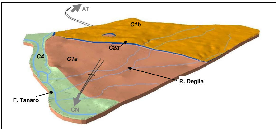
Figura 36. Dettaglio del substrato marnoso relativamente al settore Ovest del modello; rispetto alle immagini precedenti è stata parzialmente esclusa dalla visualizzazione sia la copertura affiorante dei materiali appartenenti al Complesso 1b, sia l'acquifero dei gessi del Complesso 2a.
