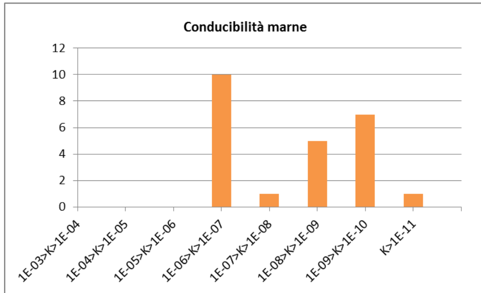
Figura 10. Diagramma di frequenza delle conducibilità idrauliche delle marne del Complesso 1a (Marne di S. Agata); conducibilità idrauliche in m/s.
