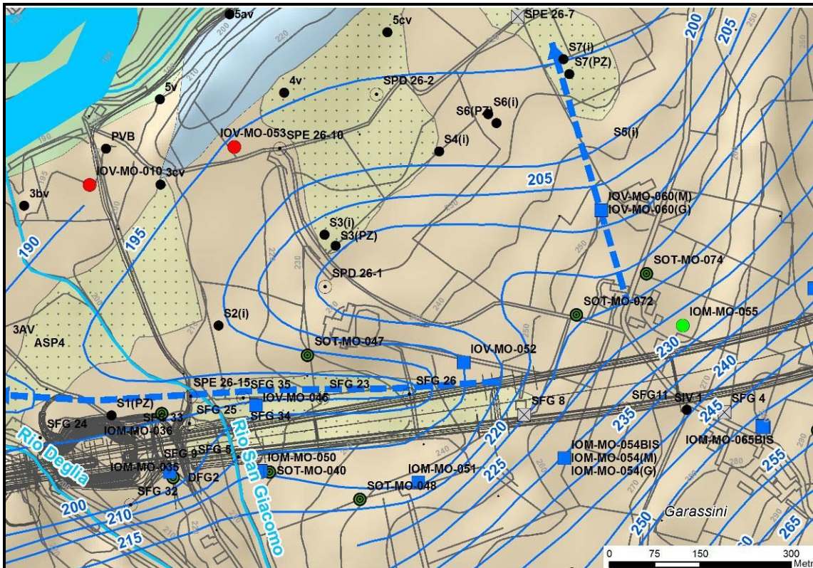
Figura 22. Distribuzione piezometrica nell'intorno del settore di attraversamento dei gessi.
