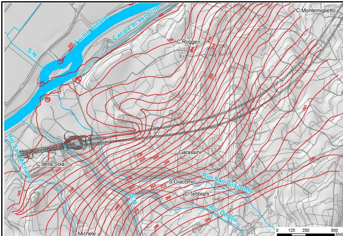
Figura 44. Distribuzione piezometrica relativa all'acquifero dei gessi ottenuta tramite la simulazione numerica.
