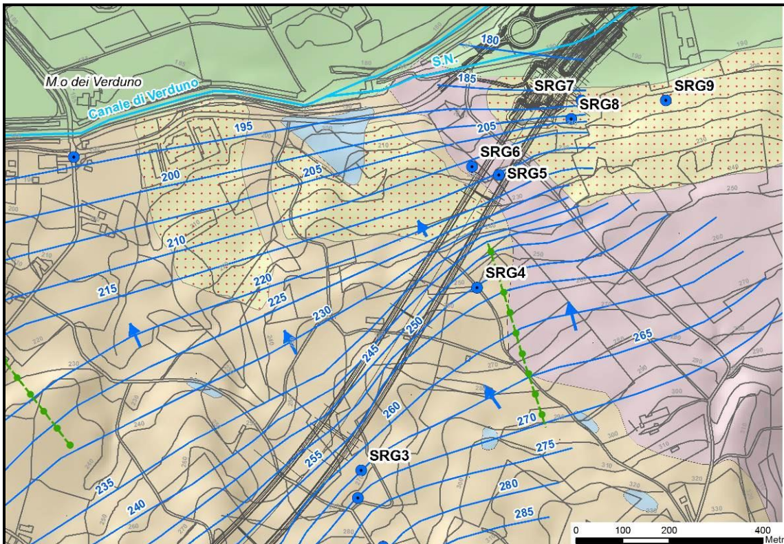
Figura 29. Distribuzione piezometrica del sistema di circolazione principale. Con i cerchi blu è riportata l'ubicazione delle principali sorgenti di questo settore; per la legenda fare riferimento alla Carta Idrogeologica.
