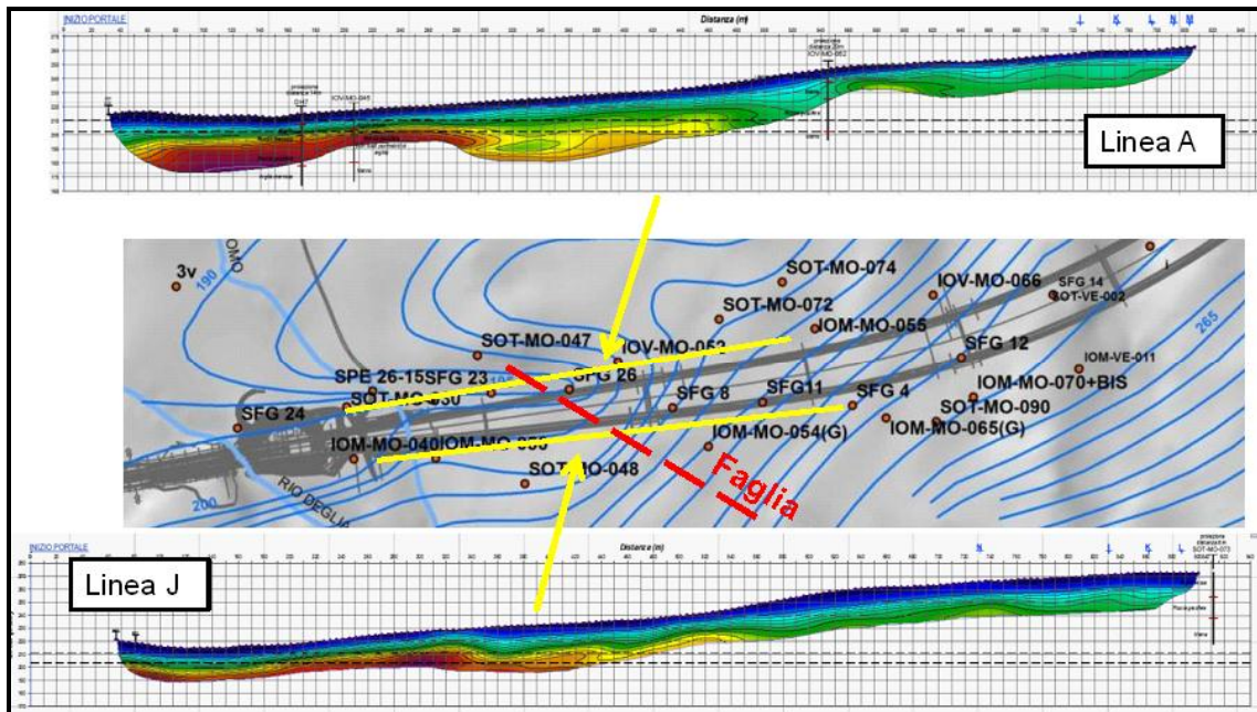
Figura 27. Profili di tomografia sismica relativi a linee di indagine tracciate a monte (Linea J) della canna di monte e a valle (Linea A) della canna di valle.
