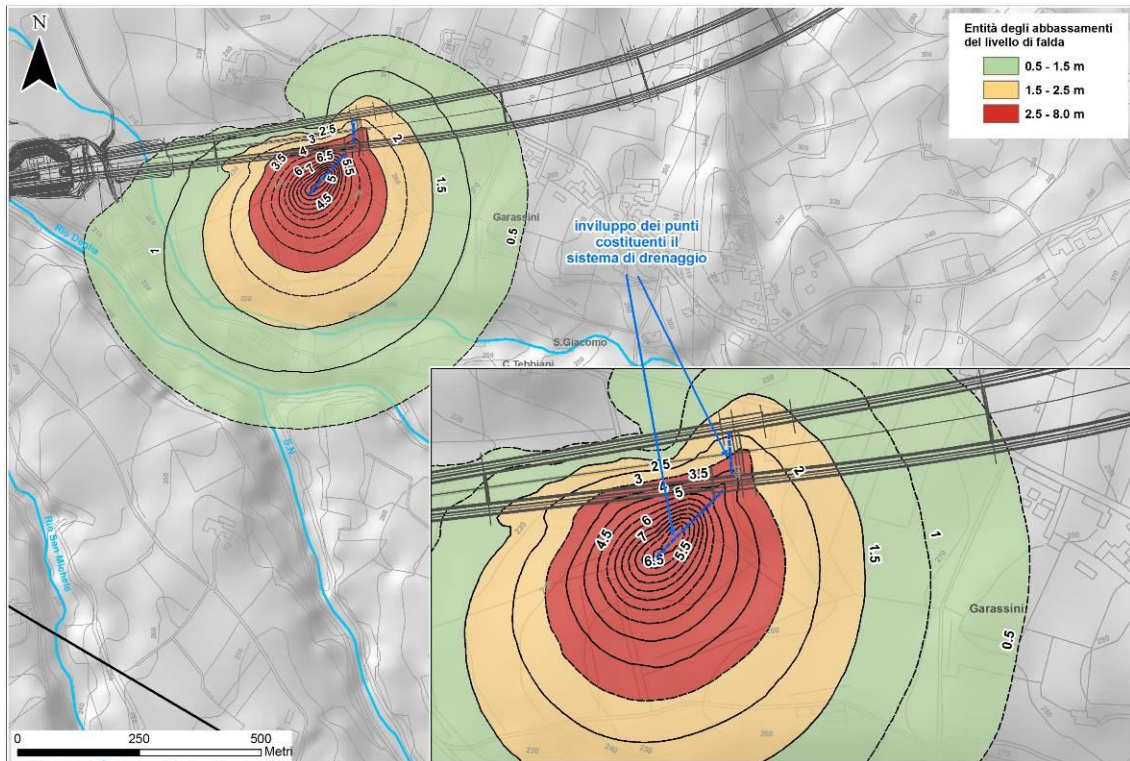
Figura 55. Rappresentazione delle variazioni di livello piezometrico dovute in seguito alla somma degli effetti derivanti dalla messa in funzione del sistema di fasci di fori drenanti; ingrandimento del settore con il massimo abbassamento nel riquadro a destra.
