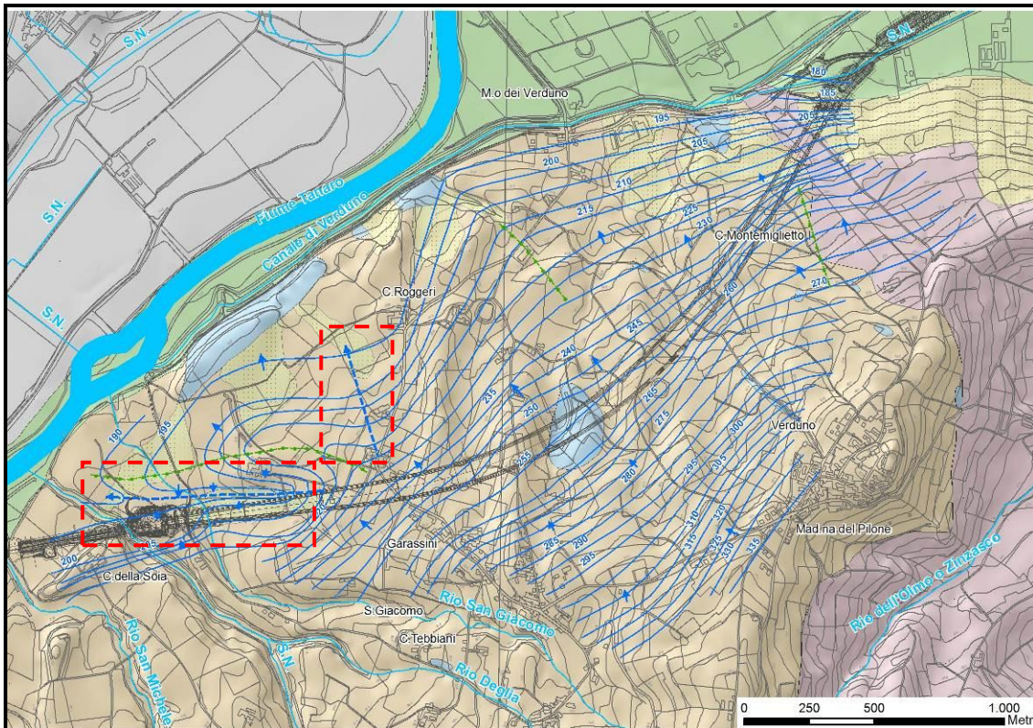
Figura 17. Ricostruzione della piezometria di falda dell'acquifero principale. Le frecce blu indicano gli assi di drenaggio principali desunti dalle caratteristiche morfologiche della falda. I due settori nel riquadro rosso sono quelli in cui sono riconoscibili due assi di drenaggio principali (tratteggio blu).
