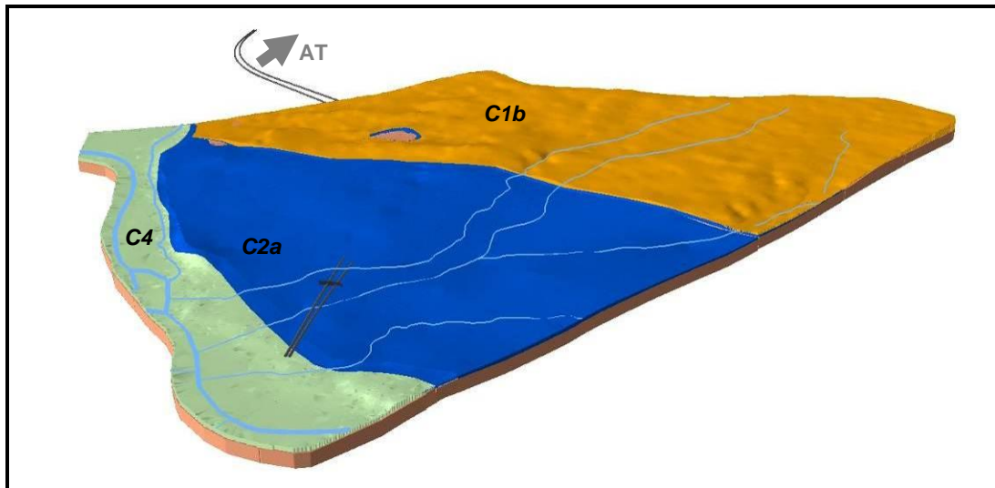
Figura 35. Dettaglio dell'acquifero dei gessi relativamente al settore Ovest del modello; rispetto all'immagine precedente è stata parzialmente esclusa dalla visualizzazione la copertura affiorante dei materiali appartenenti al Complesso 1b.
