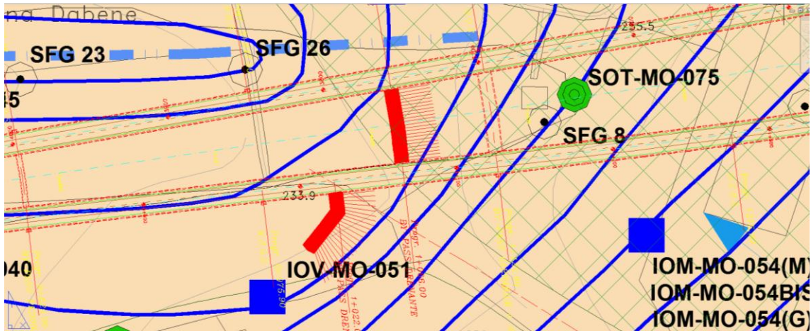
Figura 50. Estratto dello schema di realizzazione del sistema di drenaggi. I bypass sono rappresentati con le linee rosse spesse, mentre i dreni microfessurati sono rappresentati con le linee rosse sottili.
