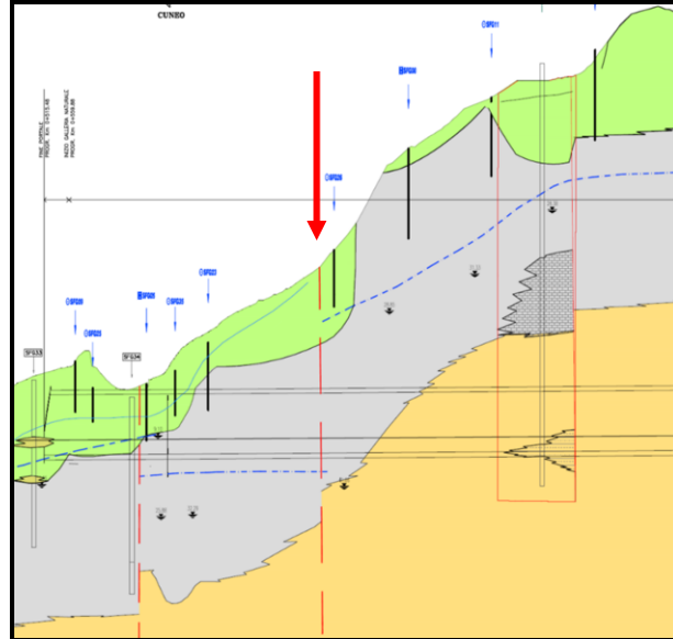
Figura 23. Profilo Geomeccanico del Progetto Definitivo con indicazione della faglia (freccia rossa) in corrispondenza della quale è stato ipotizzata la presenza di un presunto salto piezometrico.
