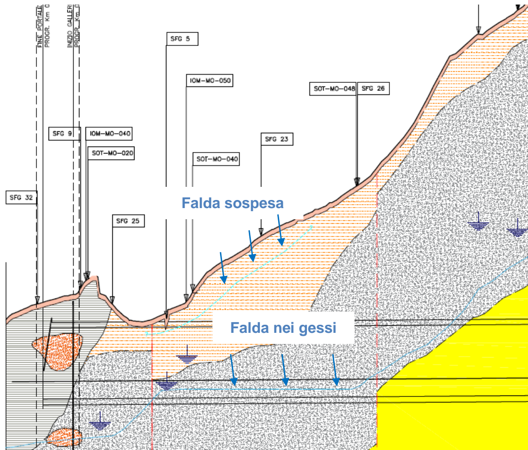
Figura 20. Rappresentazione del profilo geomeccanico della canna di monte nei settori dell'imbocco lato Cuneo e dell'attraversamento dell'acquifero dei gessi.
