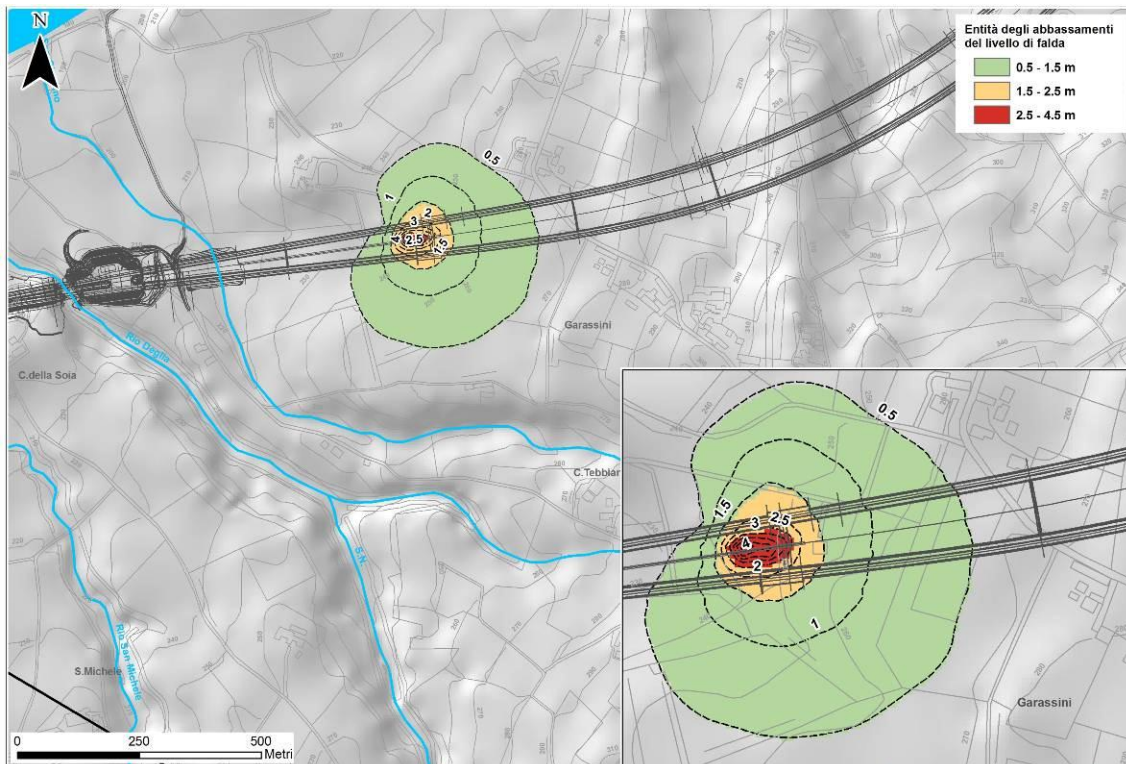
Figura 52. Rappresentazione degli abbassamenti attesi del livello piezometrico dovuto al drenaggio del cunicolo centrale all'asse delle due canne, successivamente all'attraversamento dell'acquifero dei gessi; ingrandimento del settore con il massimo abbassamento nel riquadro a destra.
