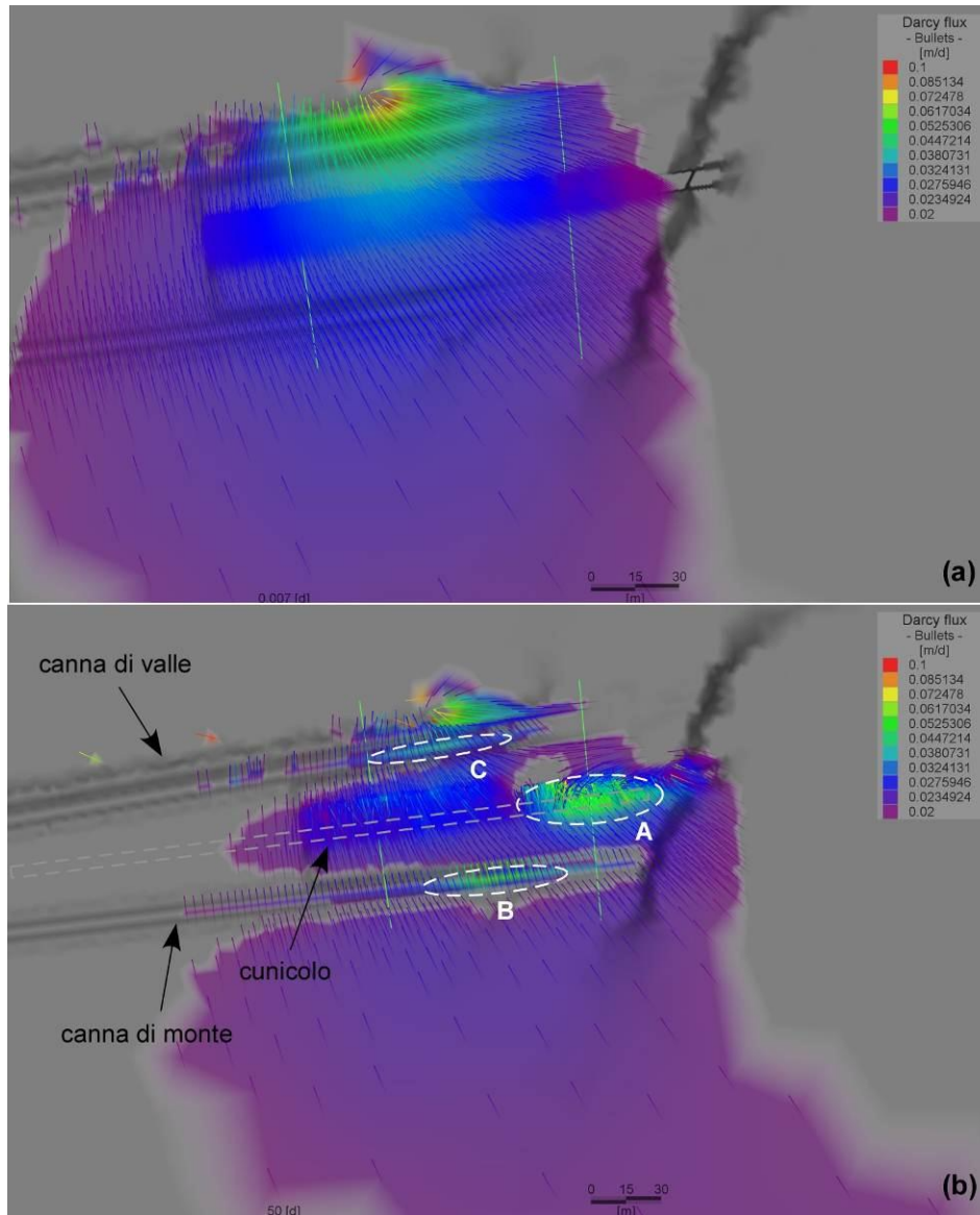
Figura 49. Confronto tra distribuzione del campo di flusso in condizioni naturali (a), ed in presenza del cunicolo drenante e delle due canne impermeabilizzate (b); i campi tratteggiati e codificati A, B e C mostrano i settori in cui vi è un locale aumento di flusso rispetto alla situazione al naturale. Nel settore a monte della galleria di valle le zone non coperte da colorazione indicano prevalentemente situazioni di deflusso di bassa entità (< 2 cm/giorno).
