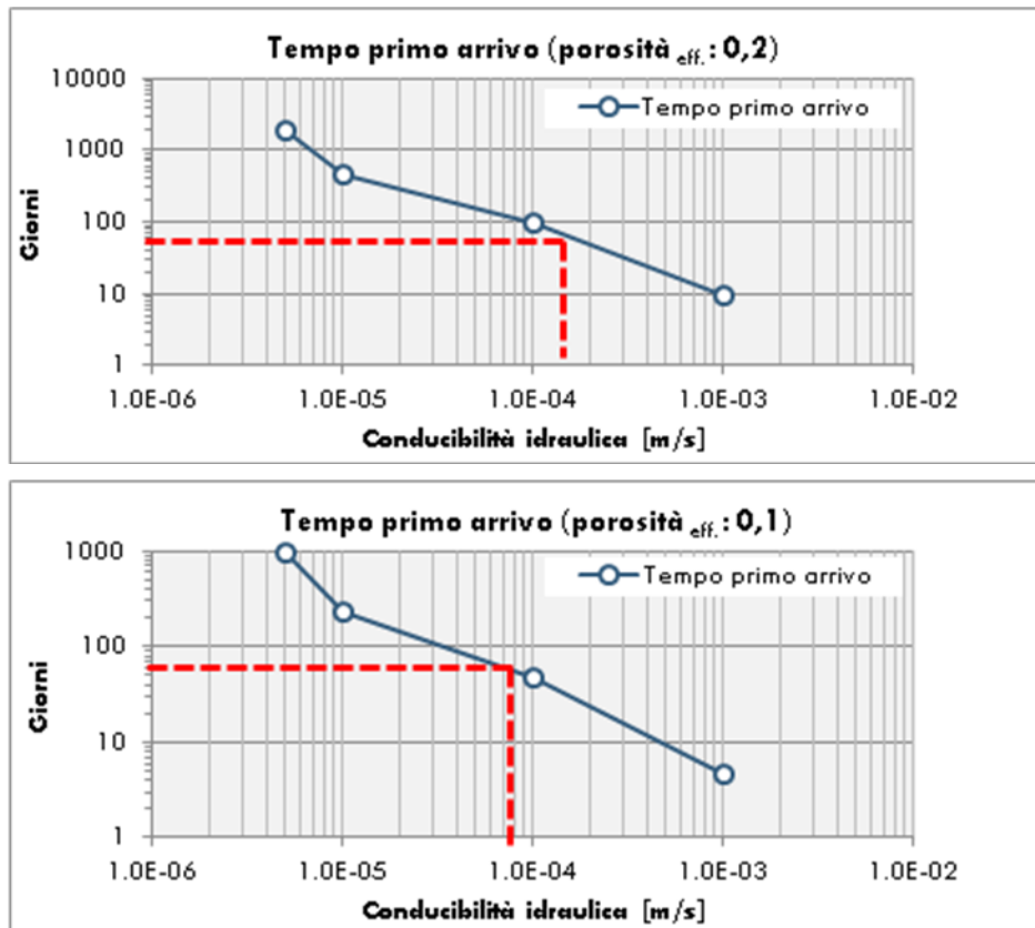
Figura 32. Diagrammi tempo di arrivo tracciante vs. conducibilità idraulica per un acquifero con porosità efficace media del 20% (diagramma in alto) e del 10% (diagramma in basso). Il diagrammi si riferiscono al caso del piezometro IOM-MO-050, che si trova a circa 500m dal piezometro di immissione IOM-MO-054. La linea tratteggiata rossa orizzontale è un'isocrona a 50gg dall'immissione, tempo circa corrispondente al periodo trascorso fino all'ultimo prelievo di fluocaptori disponibile.
