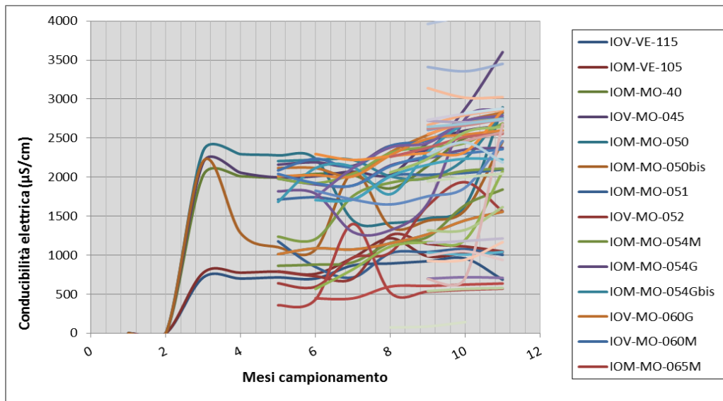
Figura 18. Variazioni delle conducibilità elettrica misurate attraverso i piezometri della rete di Monitoraggio Ambientale (Mesi di campionamento 2011-2012).
