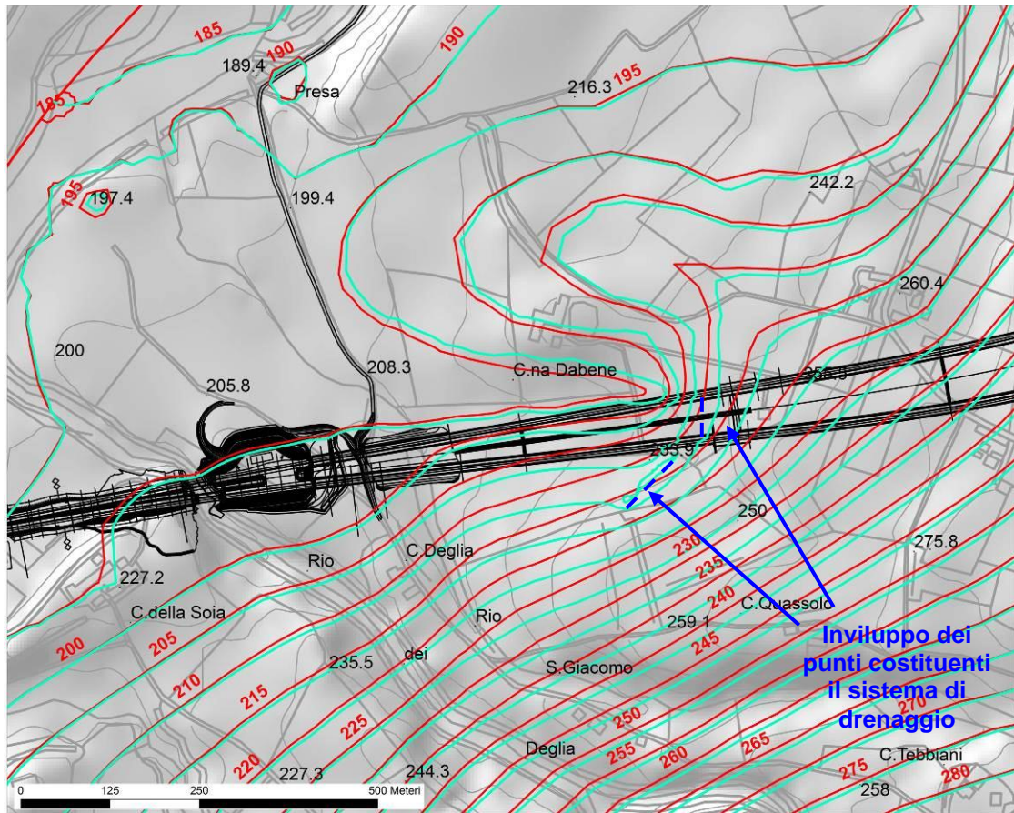
Figura 51. Confronto tra distribuzione piezometrica allo stato naturale (linee rosse) e in una situazione in cui la falda raggiunge una condizione di stabilizzazione dopo la messa in opera dei fasci di dreni connessi ai due by-pass drenanti (linee azzurre).
