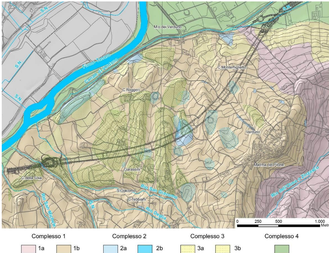
Figura 15. Rappresentazione dei Complessi Idrogeologici (il complesso 2b non è affiorante). I retini verdi e azzurri rappresentano rispettivamente zone in cui la permeabilità è tendenzialmente maggiore per effetto di una disarticolazione del substrato e della presenza di fenomeni carsici.
