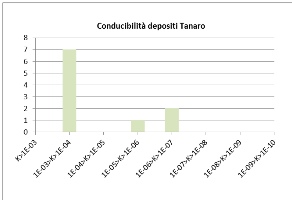
Figura 14. Diagramma di frequenza delle conducibilità idrauliche relative ai depositi alluvionali del Tanaro (Complesso 4); conducibilità idrauliche in m/s.
