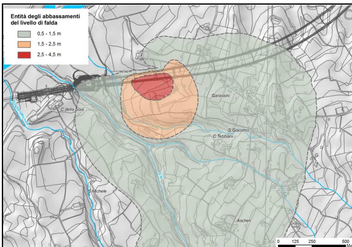
Figura 54. Rappresentazione degli abbassamenti attesi del livello piezometrico dovuto al drenaggio delle due canne della galleria successivamente all'attraversamento dell'acquifero dei gessi.
