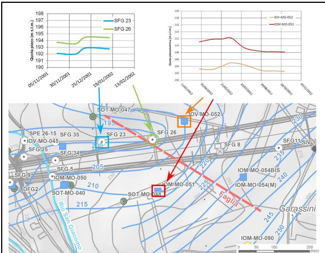
Figura 25. Confronto dell'evoluzione piezometrica tra piezometri selezionati sui due lati della presunta faglia.
