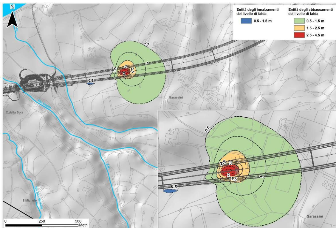
Figura 53. Rappresentazione delle variazioni (abbassamenti e innalzamenti) di livello piezometrico dovute in seguito alla somma degli effetti del drenaggio del cunicolo centrale e alla realizzazione delle due canne impermeabilizzate; ingrandimento del settore con il massimo abbassamento nel riquadro a destra.
