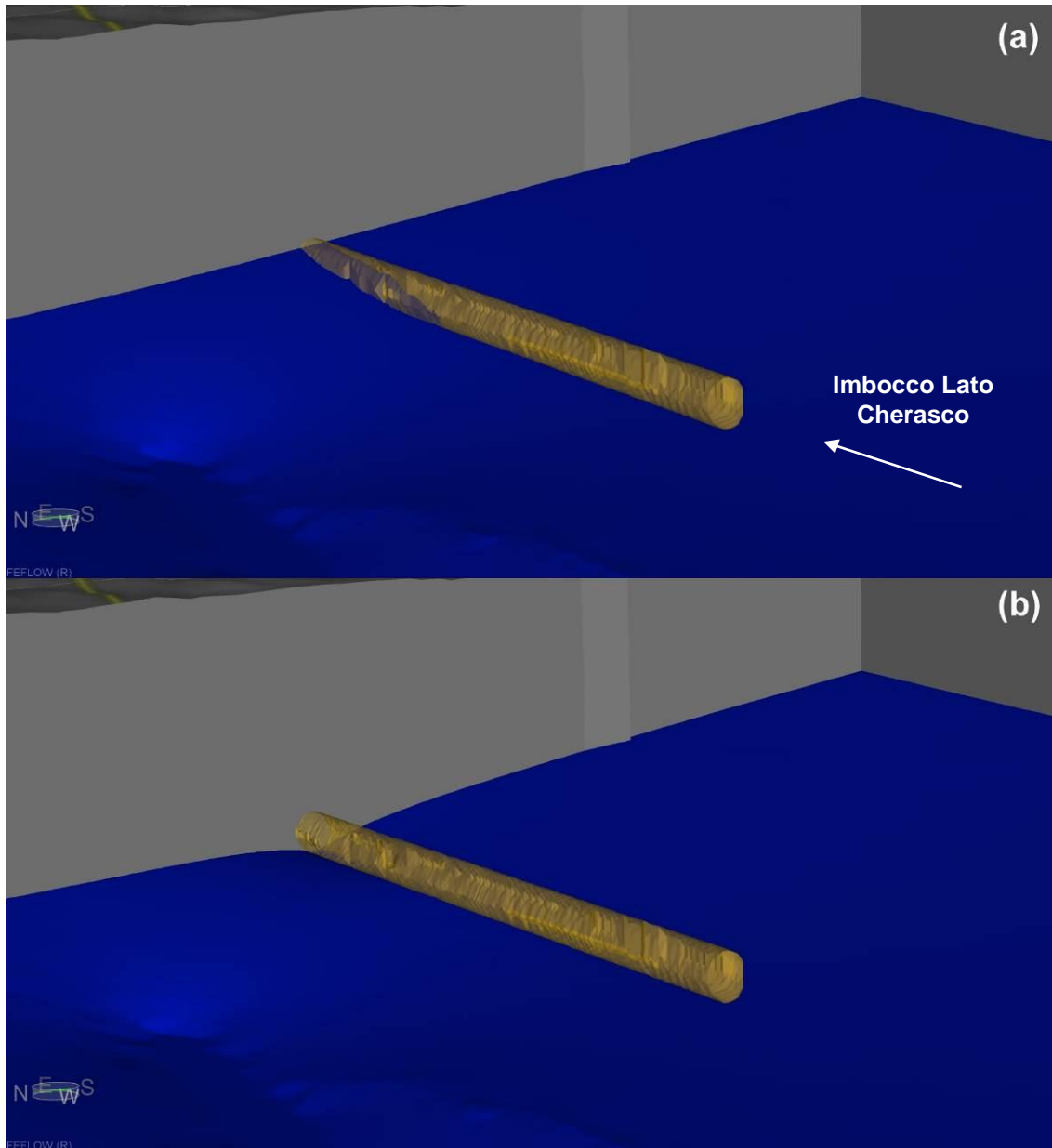
Figura 46. Visualizzazione prospettica del cunicolo con confronto tra la superficie piezometrica (a) prima del drenaggio ad opera del cunicolo (situazione ante-operam) e (b) in seguito al drenaggio della falda da parte del cunicolo (situazione stabilizzata).
