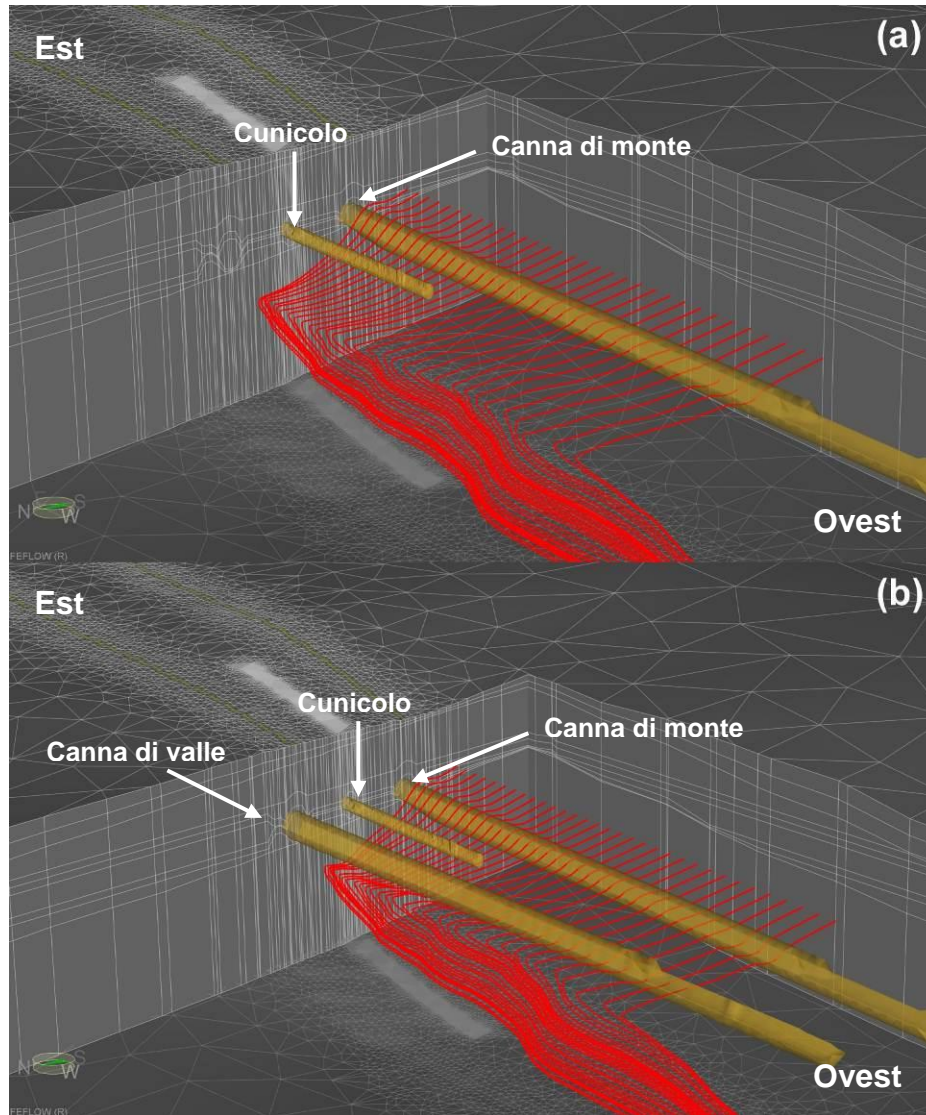
Figura 48. Rappresentazione delle linee di flusso (in rosso) nell'acquifero dei gessi relativamente alla fase di realizzazione della galleria di monte (a) e, successivamente, della galleria di valle (b).
