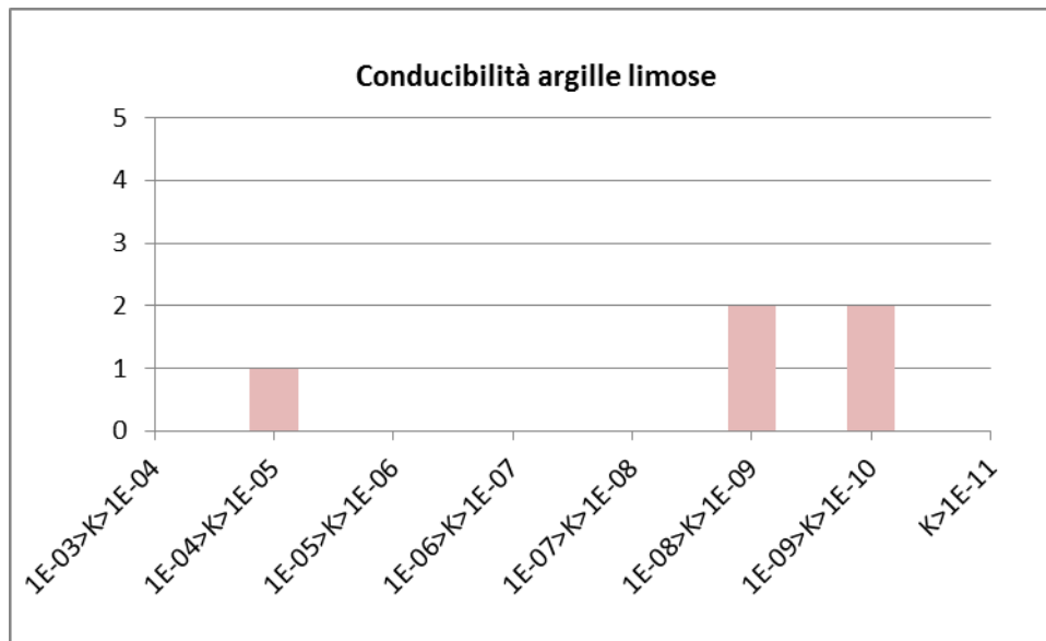
Figura 11. Diagramma di frequenza delle conducibilità idrauliche relative ai limi argillosi e alle argille marnose del Complesso 1b; conducibilità idrauliche in m/s.
