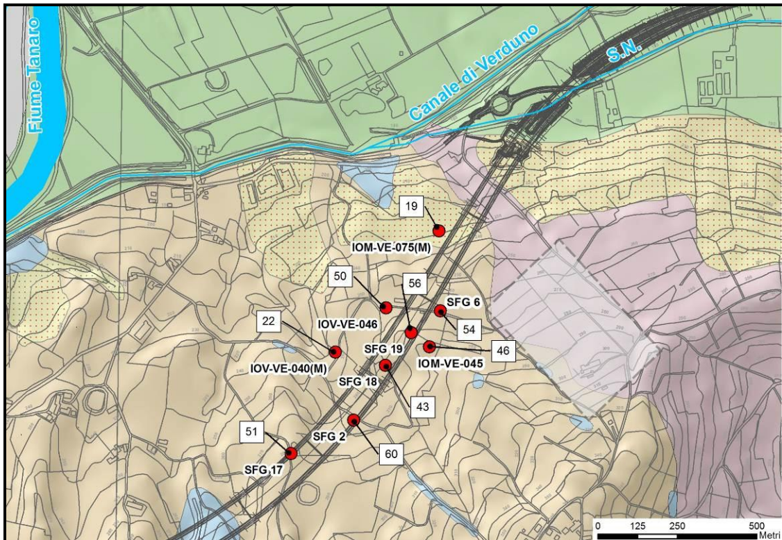
Figura 28. Carta con ubicazione dei piezometri con fenestratura nelle intercalazioni detritiche. Il valore riportato è relativo al carico idraulico medio [m] misurato rispetto alla quota di progetto della galleria.
