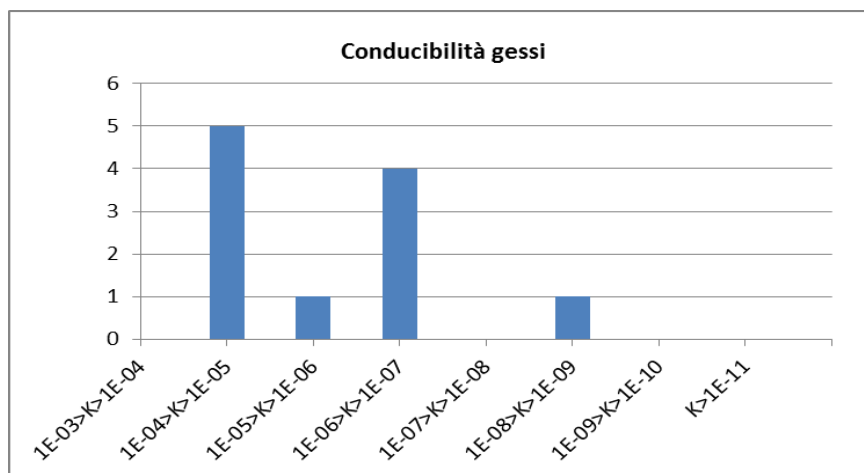
Figura 12. Diagramma di frequenza delle conducibilità idrauliche relative ai gessi del Complesso 2a; conducibilità idrauliche in m/s.
