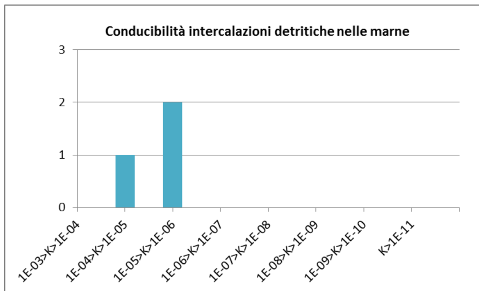
Figura 13. Diagramma di frequenza delle conducibilità idrauliche relative alle intercalazioni ghiaioso-sabbiose del Complesso 2b; conducibilità idrauliche in m/s.
