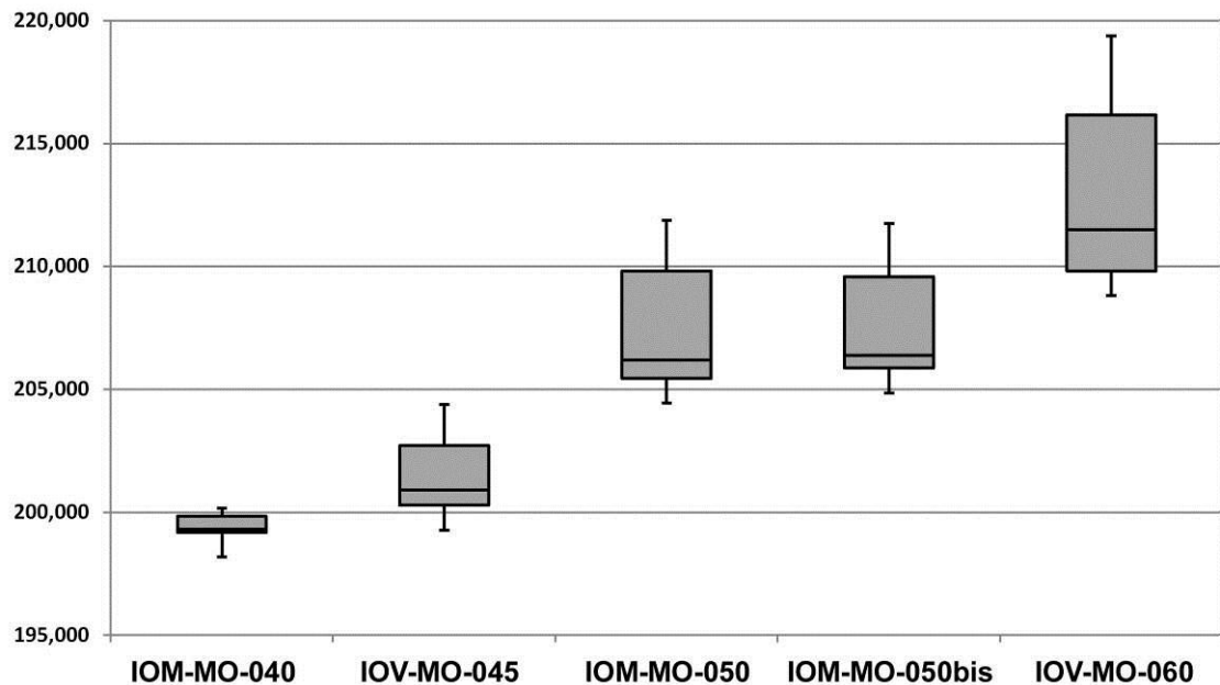
Figura 21. Box-plot delle oscillazioni piezometriche di 5 piezometri della rete di Monitoraggio Ambientale selezionati tra quelli con fenestratura nell'acquifero dei gessi.
