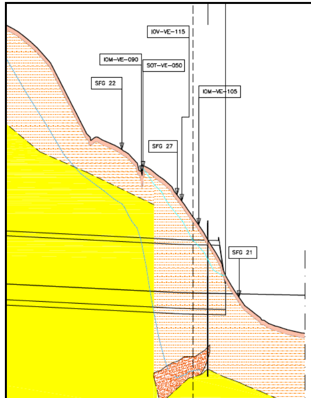
Figura 30. Profilo longitudinale lungo la canna di monte nel settore dell'imboccato lato Alba; sono riportati i livelli della falda profonda e di quella superficiale.
