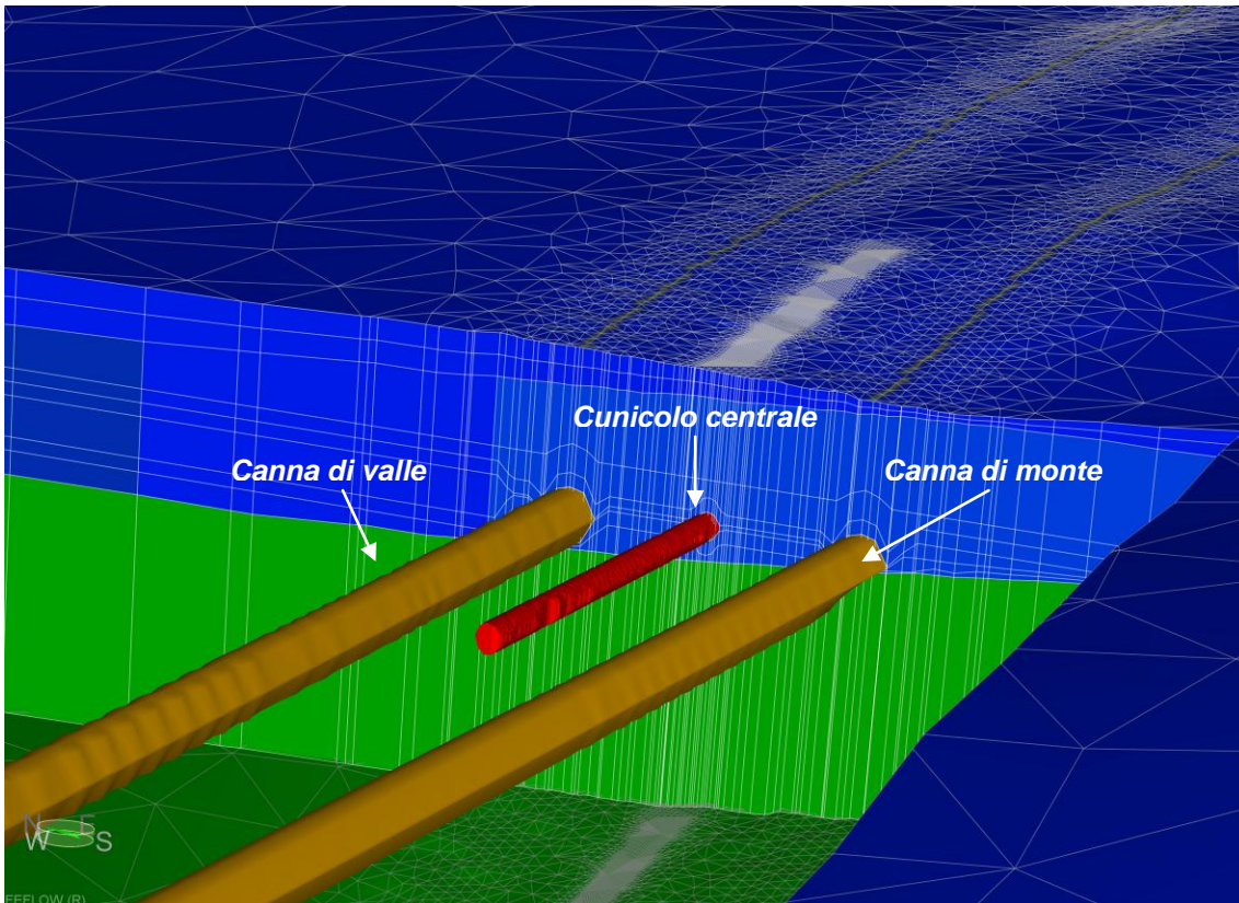
Figura 41. Dettaglio delle due canne del tunnel utilizzate per la simulazione del drenaggio della falda, con spaccato utile per comprendere le geometrie interne dei layer con cui è stato costruito il modello numerico; diversa visione prospettica rispetto alla figura precedente.
