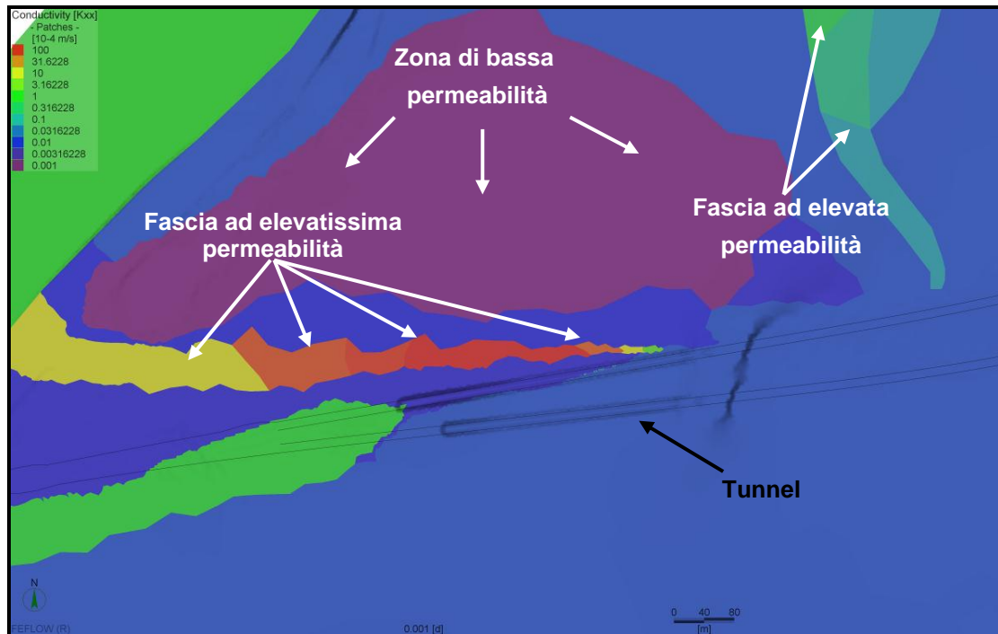
Figura 43. Dettaglio relativo alle conducibilità idrauliche utilizzate (vista in pianta); il layer del modello visualizzato è quello relativo all'acquifero dei gessi.
