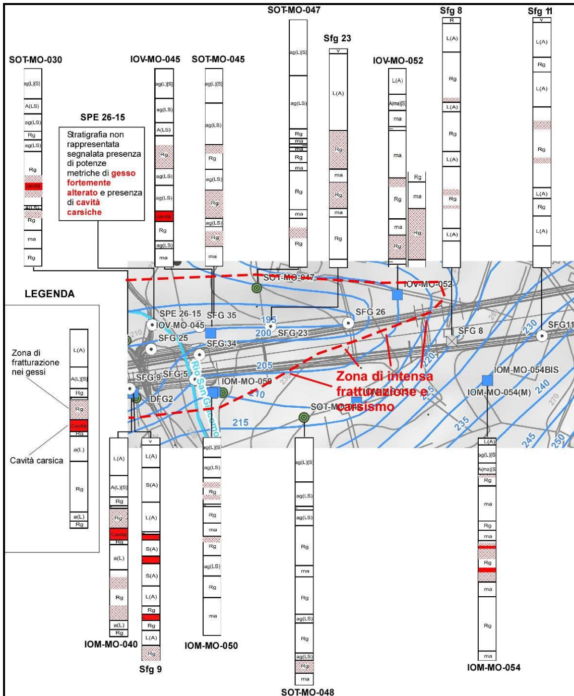
Figura 26. Illustrazione schematica di alcune stratigrafie di sondaggio nel settore dei gessi. La linea rossa tratteggiata demarca una zona in cui all'interno i gessi sono intensamente fratturati e soggetti a fenomeni di dissoluzione carsica.
