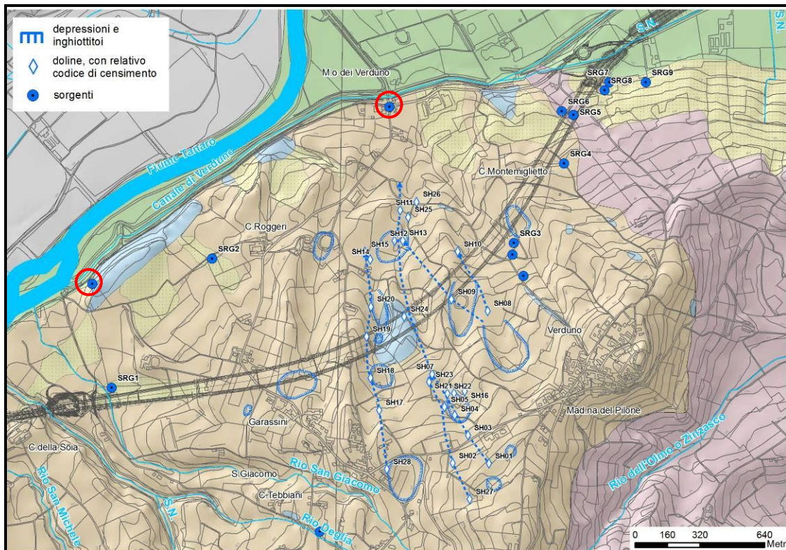
Figura 16. Possibili linee di drenaggio sotterranee ricavate dalla correlazione spaziale tra le doline/inghiottitoi (dal censimento eseguito dal Comune di Verduno, 2011) e ubicazione delle sorgenti (in rosso le sorgenti con acclarata alimentazione da parte dell'acquifero dei gessi); per la legenda dei Complessi idrogeologici fare riferimento alla Carta idrogeologica allegata.
