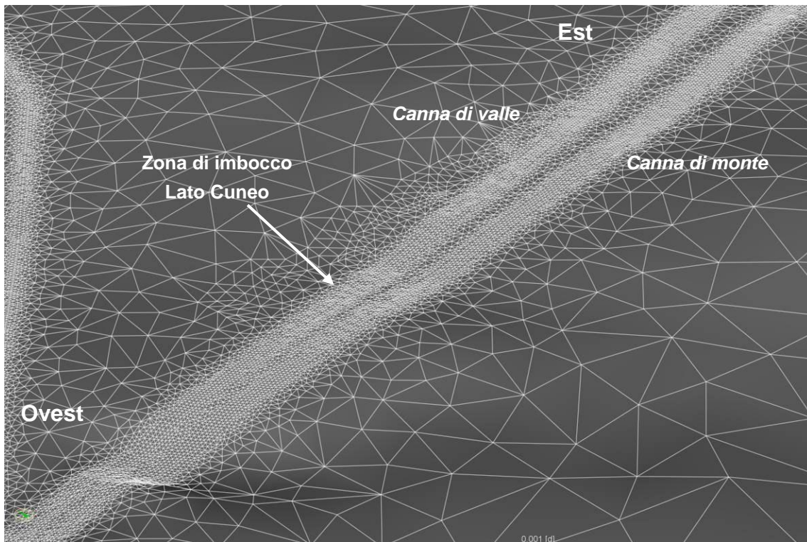
Figura 38. Dettaglio della della zona di imbocco con evidenza dell'elevato raffinamento degli elementi finiti.
