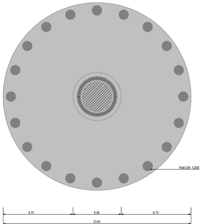
Fig. 4.1.1 pianta e sezione fondazione tipo
