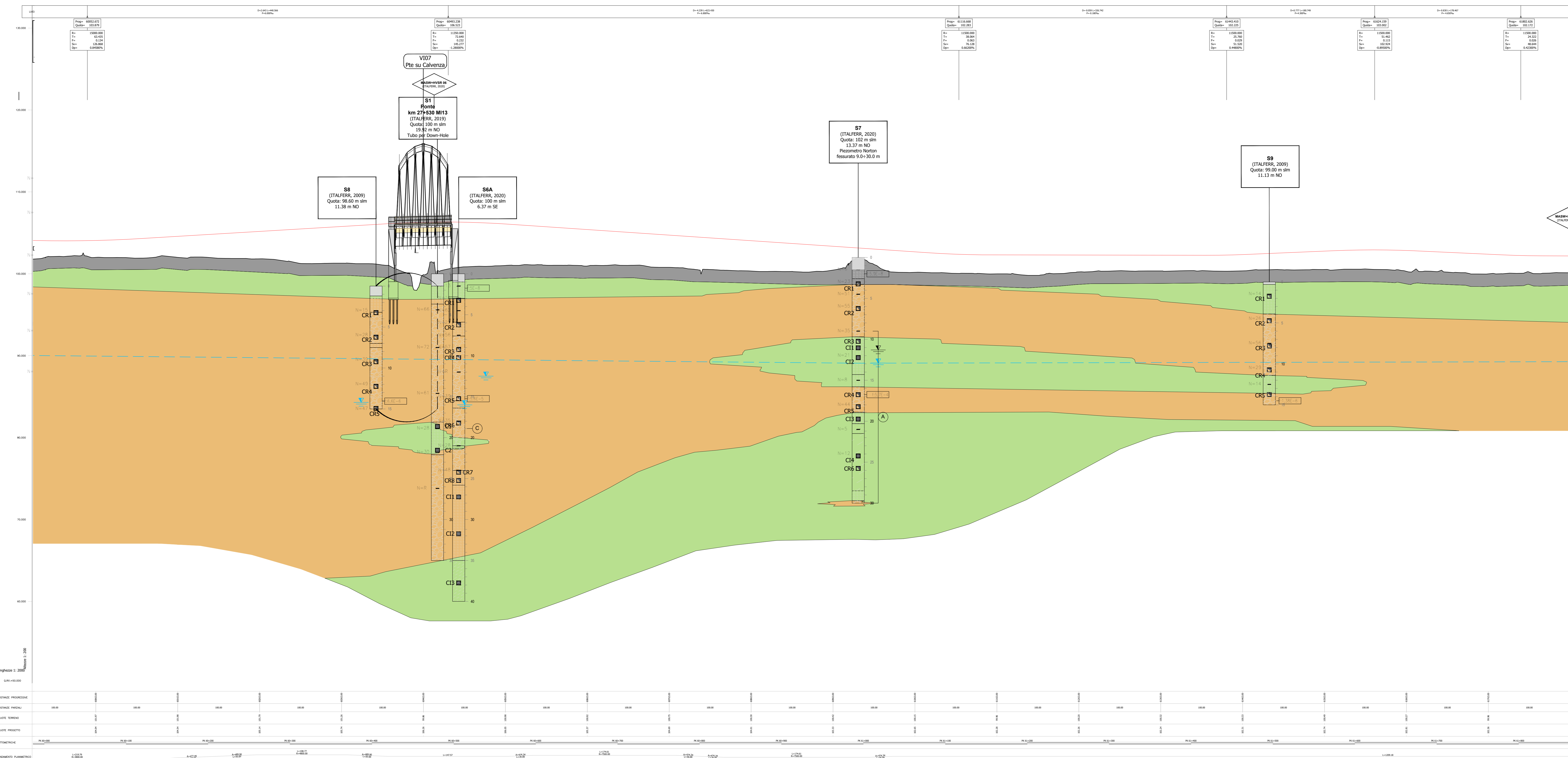
Profilo geotecnico Scala 1:2000/200
