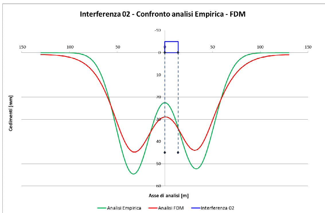
Figura 17 – Confronto bacini di subsidenza
