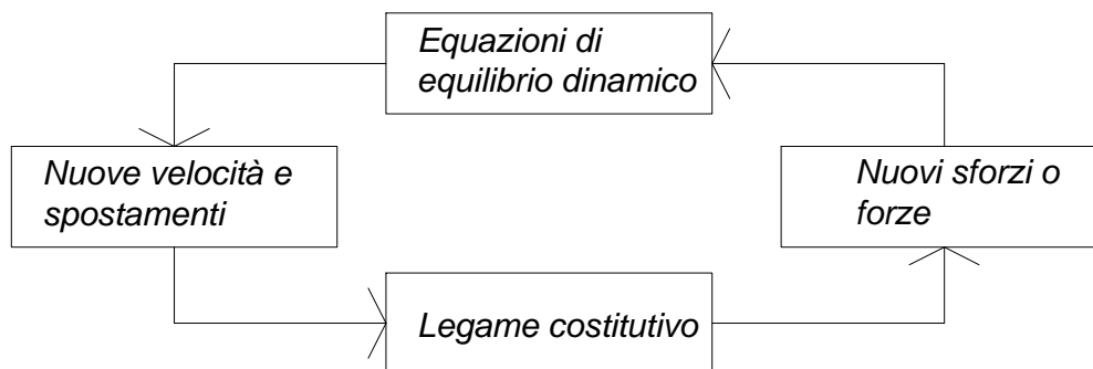
Figura 13 – Fasi di computazione del codice di calcolo FLAC
