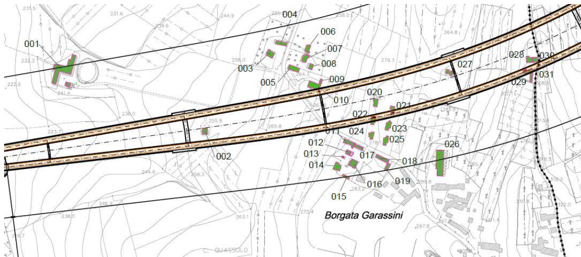
Figura 10 – Planimetria edifici interferenti (Borgata Garassini)
