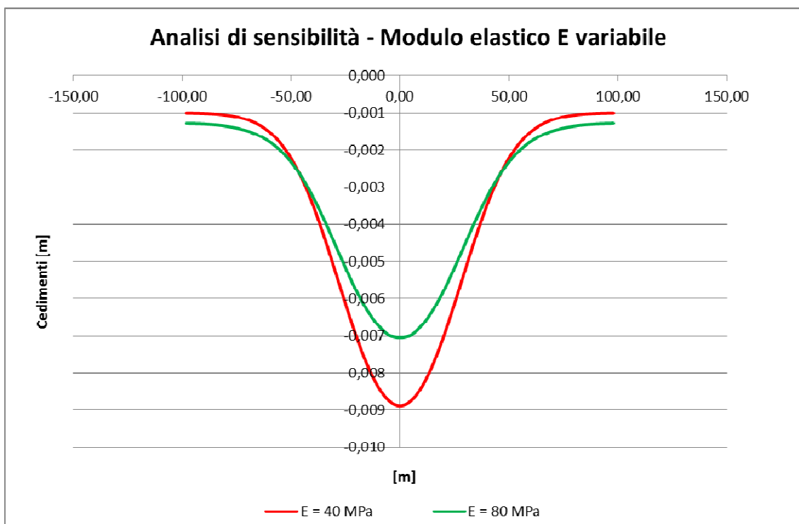
Figura 21 – Cedimenti al variare di E
