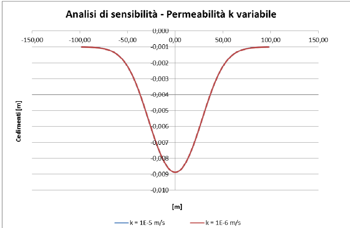
Figura 20 – Cedimenti al variare di k
