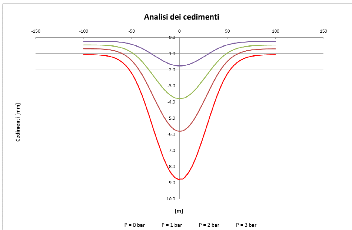
Figura 23 – Cedimenti a piano campagna
