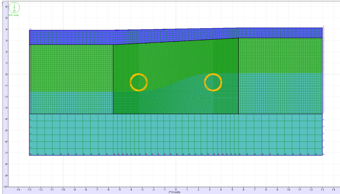
Figura 15 – Mesh di calcolo
