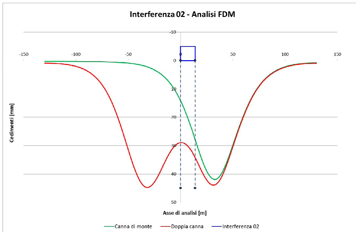
Figura 16 – Bacino di subsidenza
