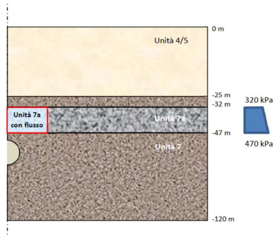
Figura 19 – Modello di calcolo
