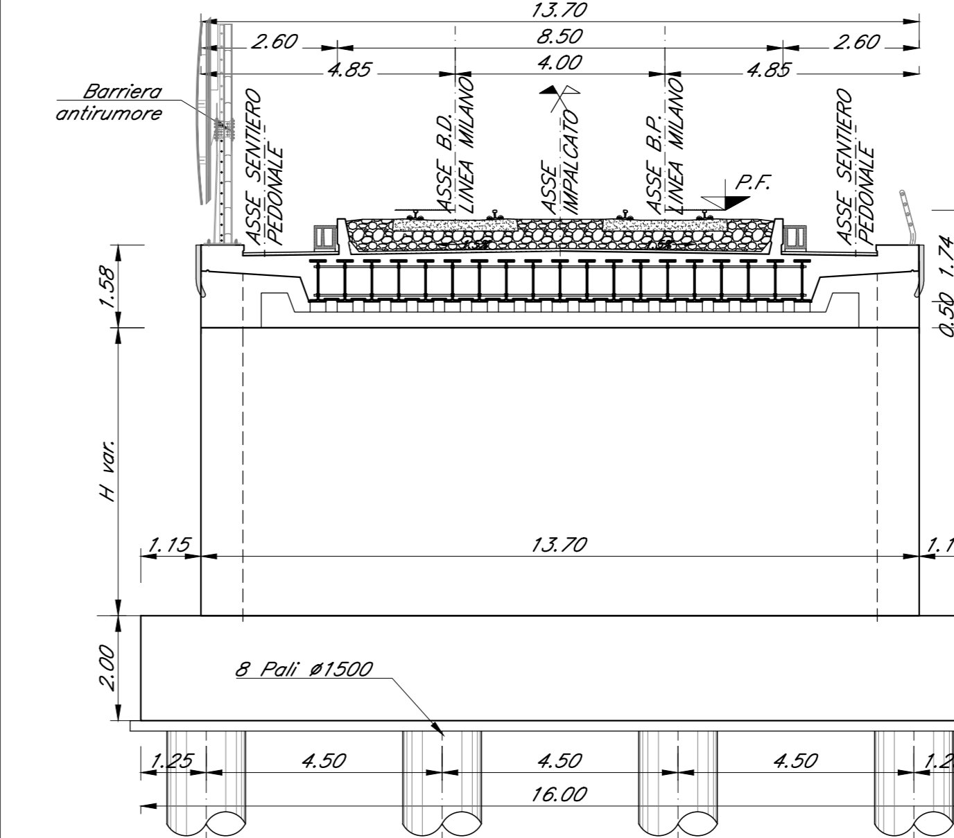
SEZIONE TRASVERSALE TIPO Scala 1:100
