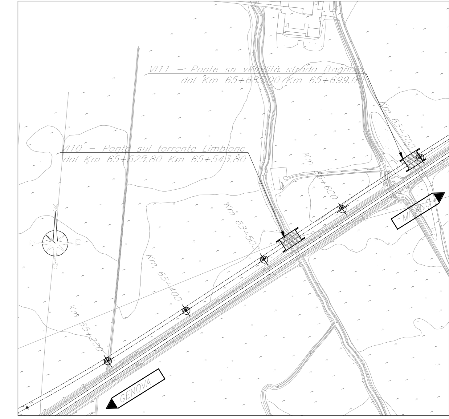
PIANTA CHIAVE
