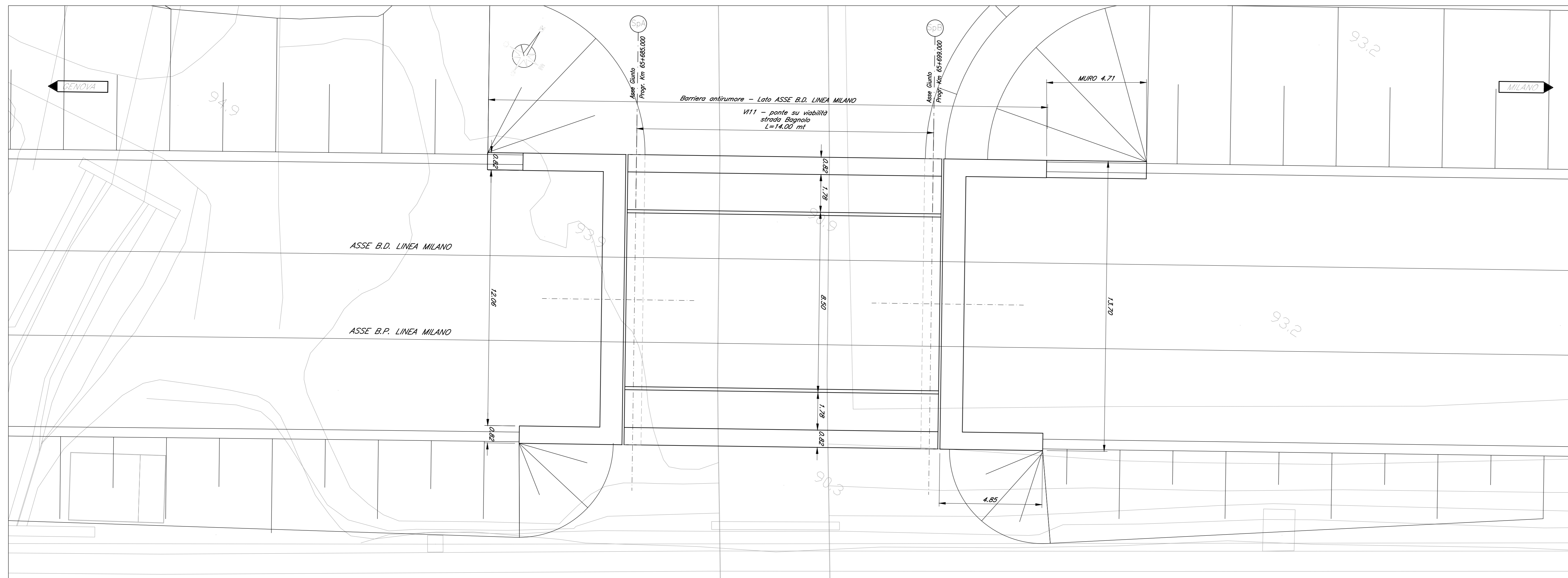
PIANTA FONDAZIONI Scala 1:100
