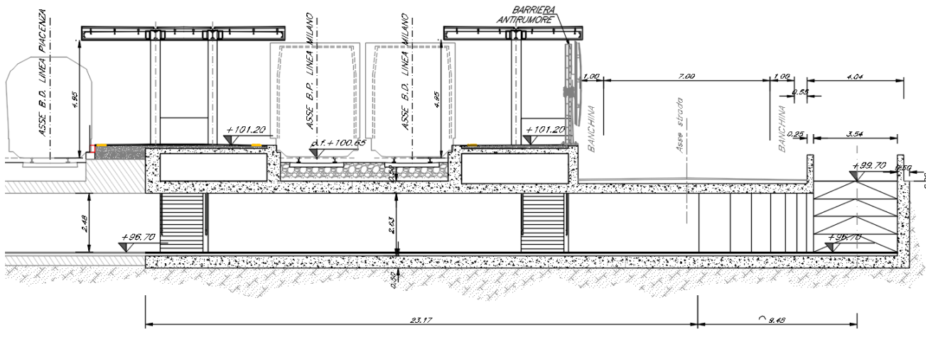
Figura 2: Stralcio sezione longitudinale finita
