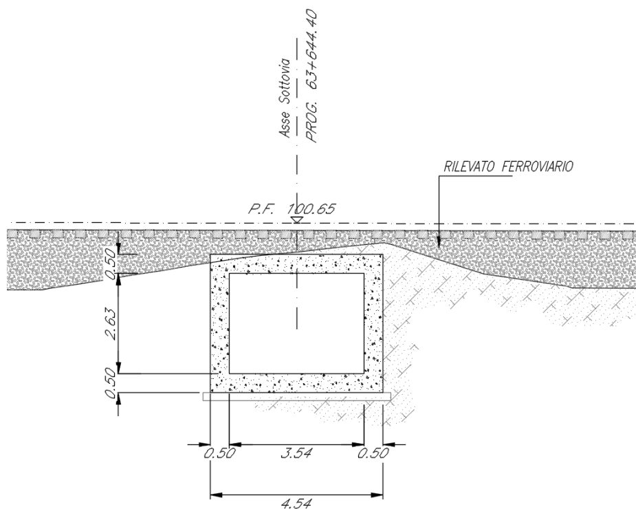
Figura 1: Sezione trasversale del sottovia
