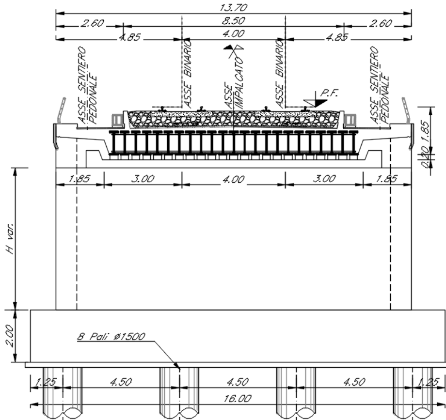
Figura 2: Sezione tipo su Spalla A
