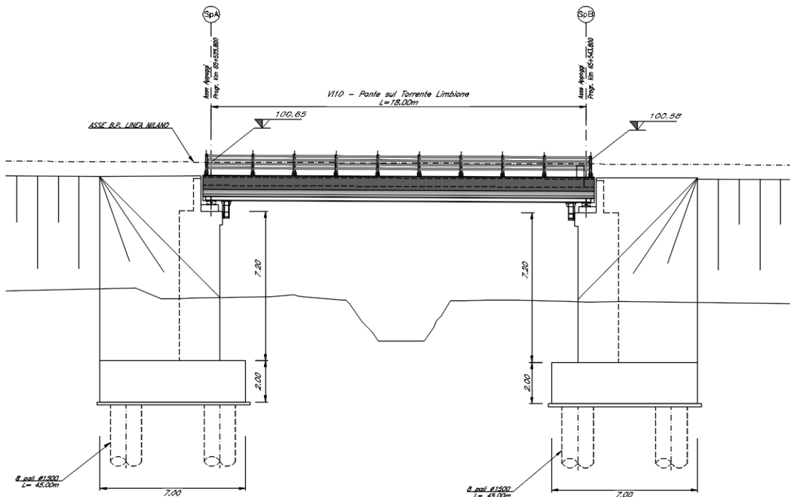
Figura 1: Stralcio prospettico del viadotto
