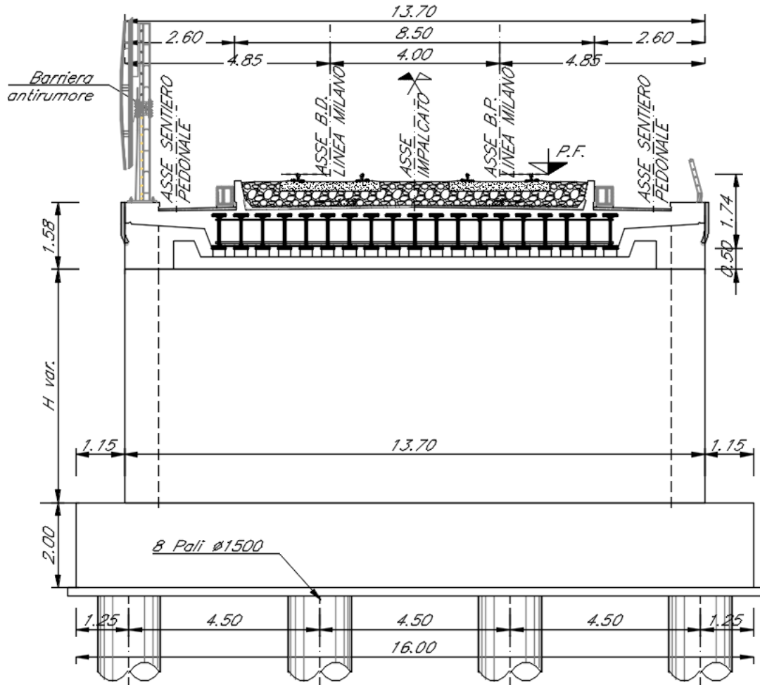
Figura 2: Sezione tipo su Spalla A
