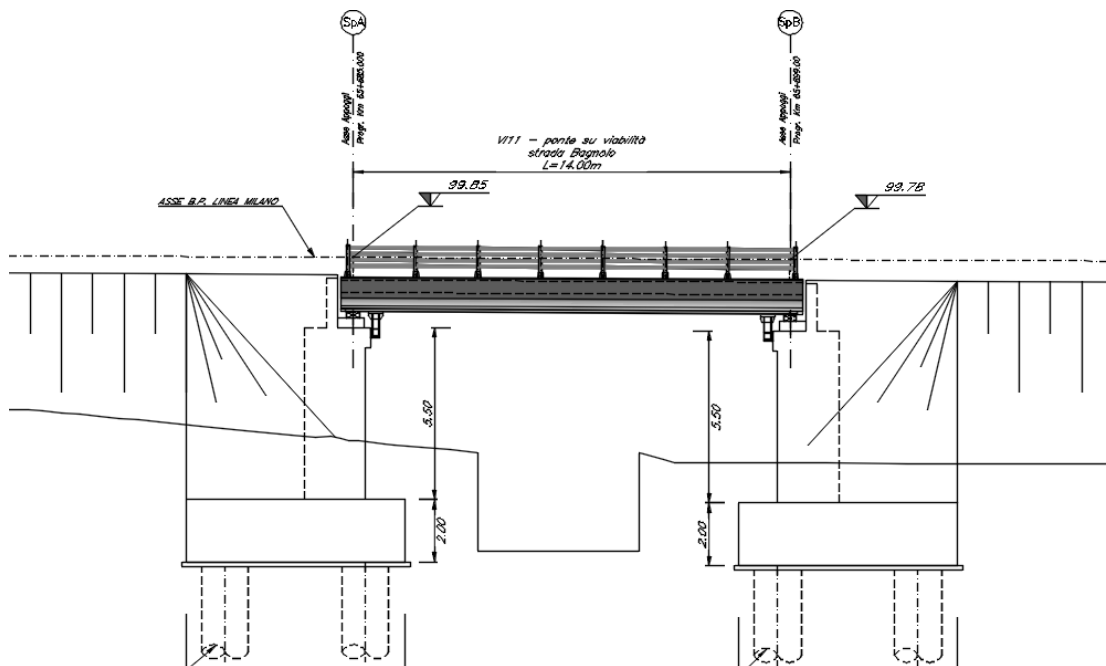
Figura 1: Stralcio prospettico del viadotto
