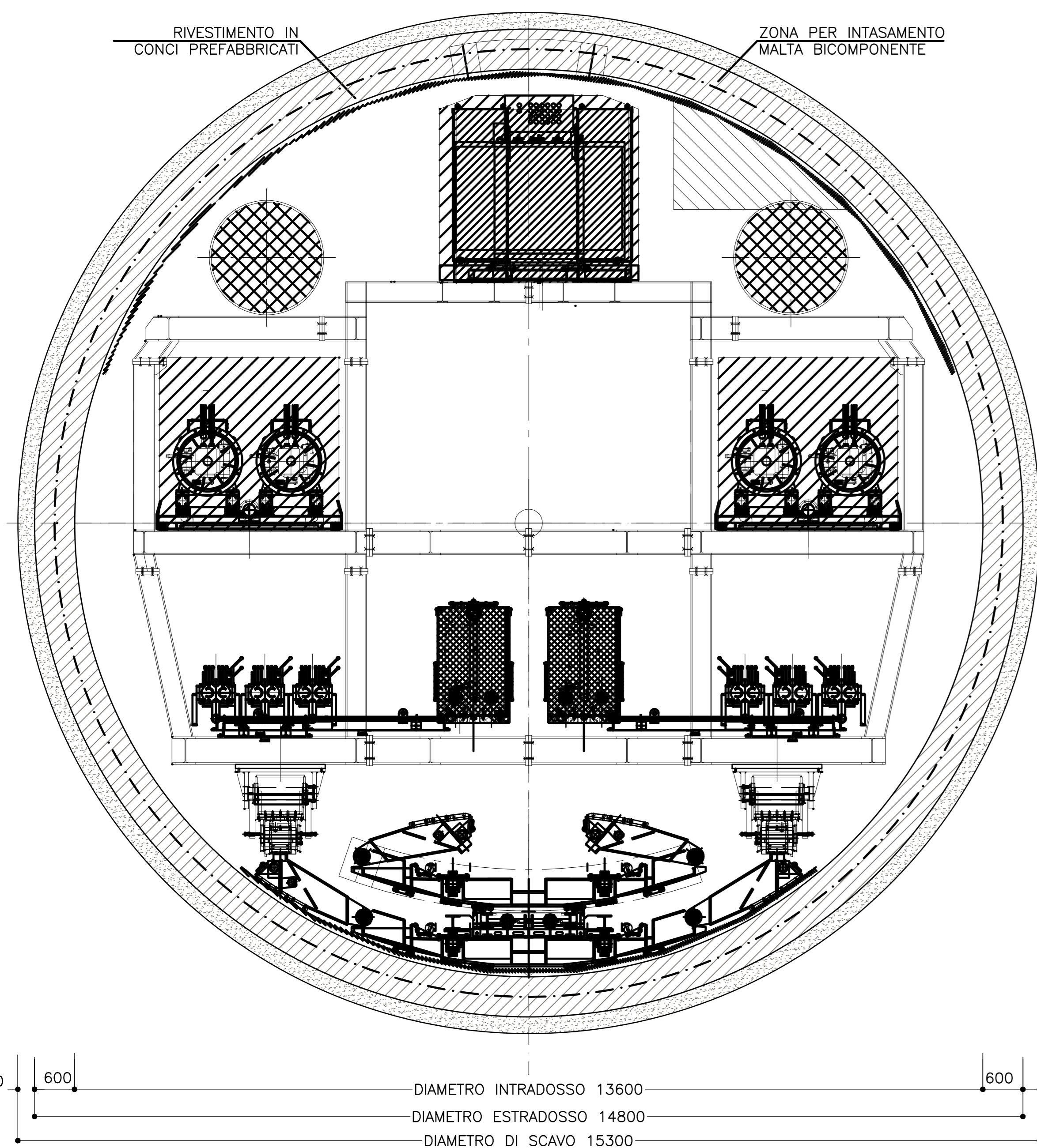
SEZIONE TRASVERSALE TBM
