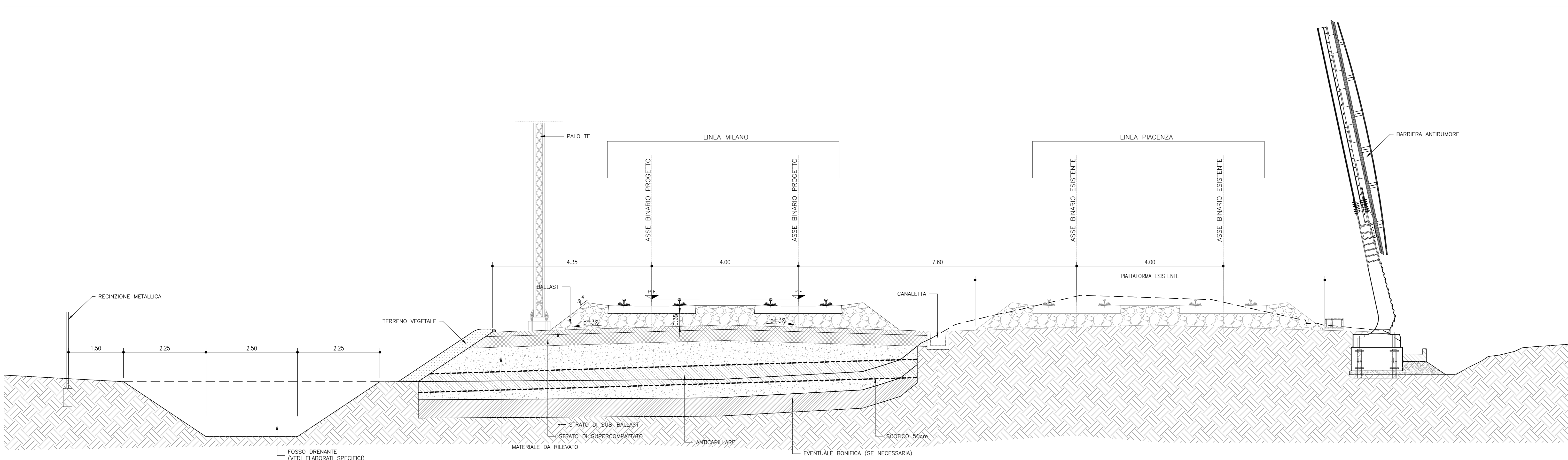
SEZIONE TIPO IN RILEVATO - INTERASSE ESISTENTE/PROGETTO = 7.60m SCALA 1:50
