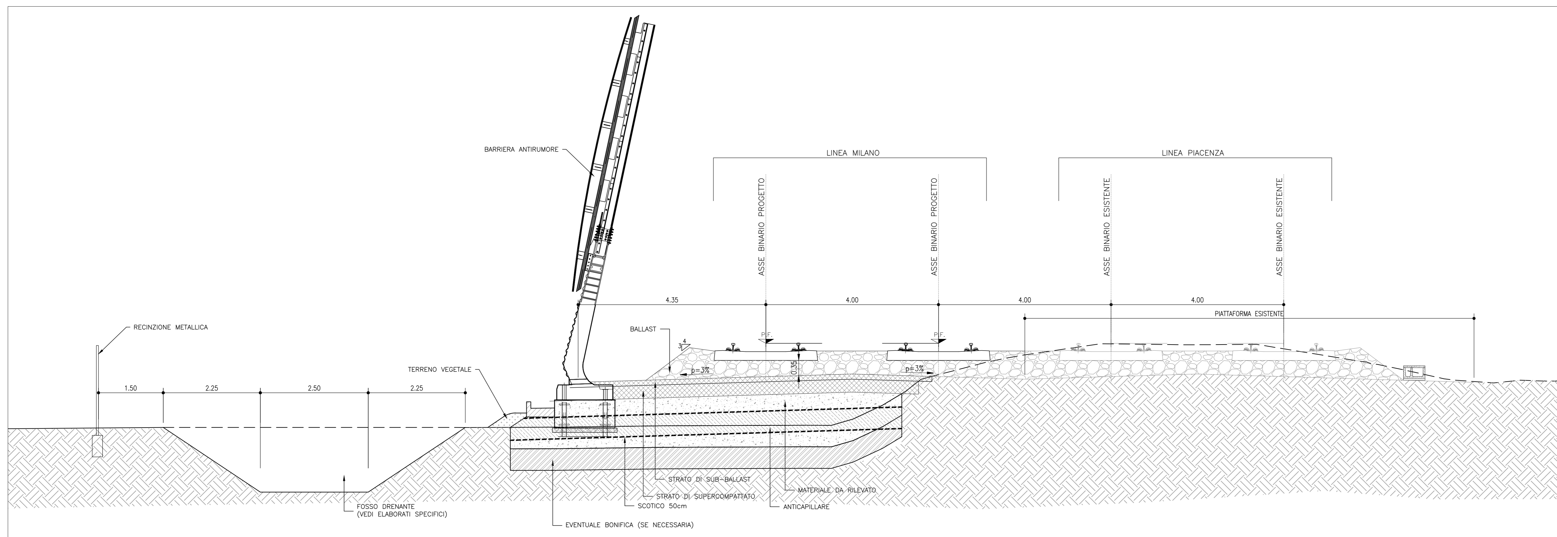
SEZIONE TIPO IN RILEVATO - INTERASSE ESISTENTE/PROGETTO = 8.60m SCALA 1:50
