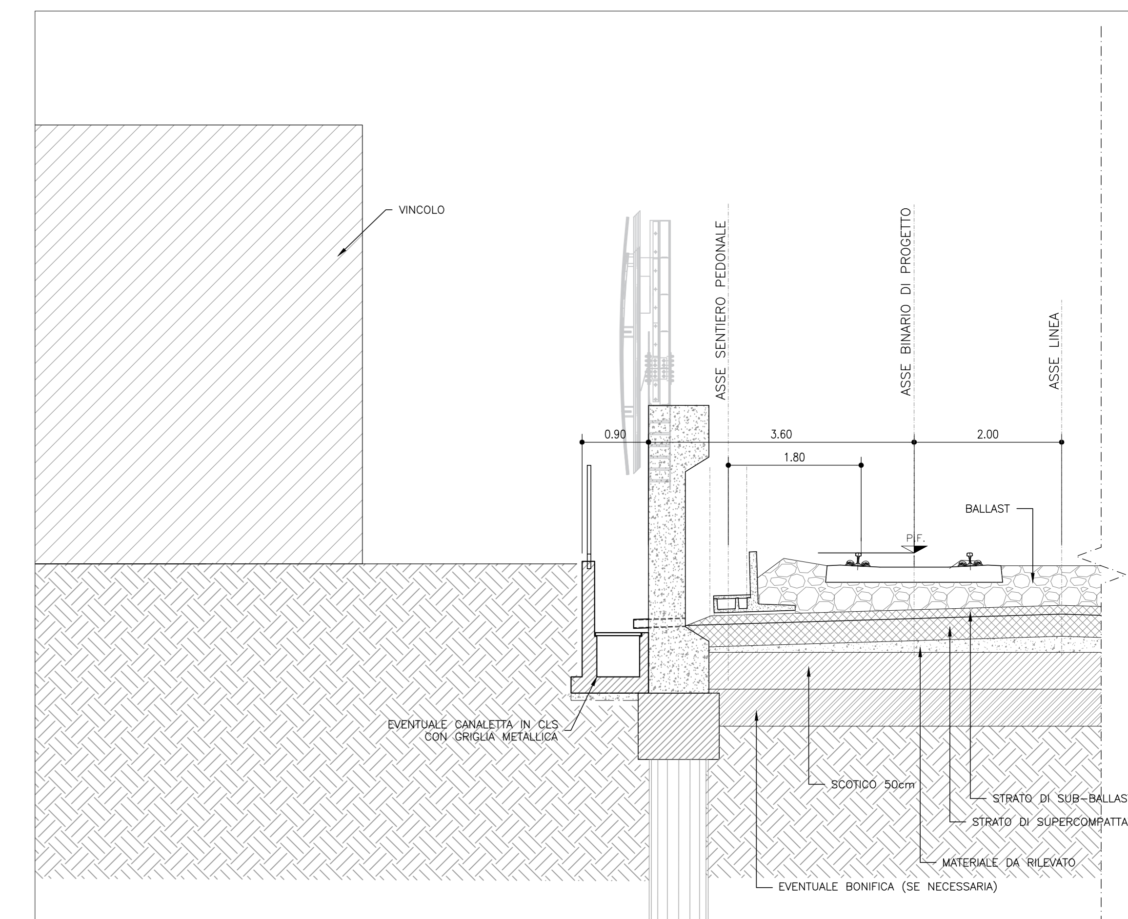
SEZIONE TIPO RIDOTTA - INTERASSE PROGETTO/MURO RECINZIONE = 3.60m SCALA 1:50
