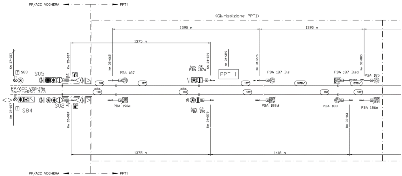
FIGURA 4 – PPT1 STATO INERZIALE
