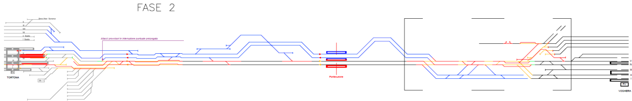
FIGURA 14 - FASE 2 INTERVENTO DI QUADRUPPLICAMENTO TORTONA-VOGHERA
