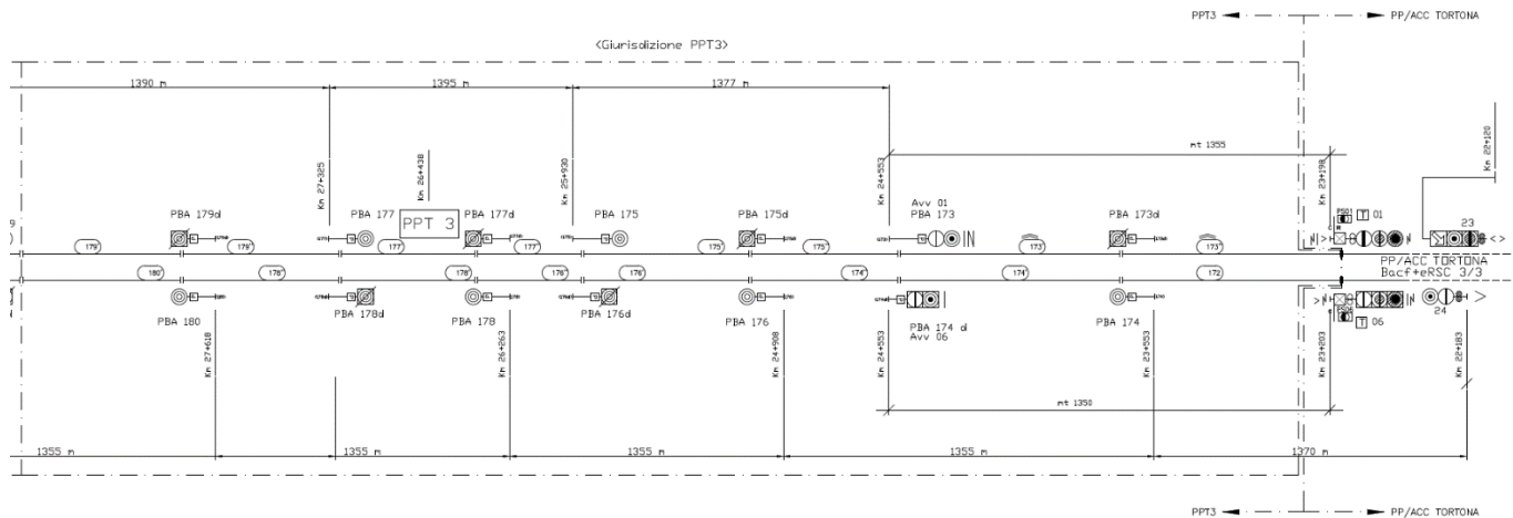
FIGURA 6 – PPT3 STATO INERZIALE
