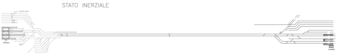
FIGURA 3 - STATO INERZIALE TORTONA-VOGHERA
