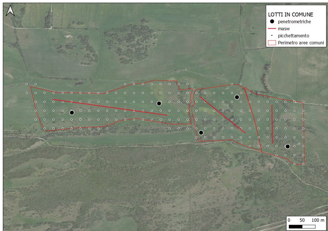
Figura 12: Planimetria delle indagini eseguite nei lotti comuni
