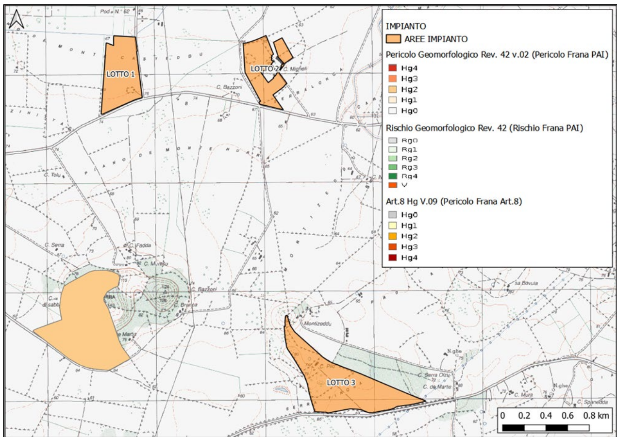
Fig. 1: Stralcio del P.A.I. (Piano di Assetto Idrogeologico) RISCHIO e PERICOLOSITÀ GEOMORFOLOGICA secondo l'art. 42 e 8 redatto dalla Regione Autonoma della Sardegna
