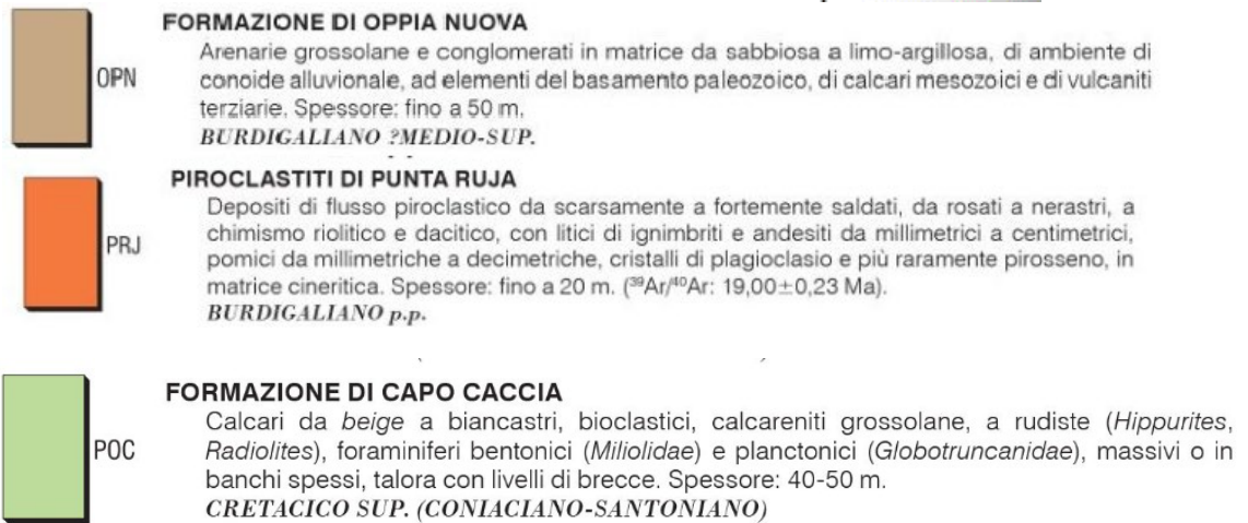
Figura 10: stralcio del F.459” Sassari” della Carta Geologica d'Italia in scala 1:50.000.
