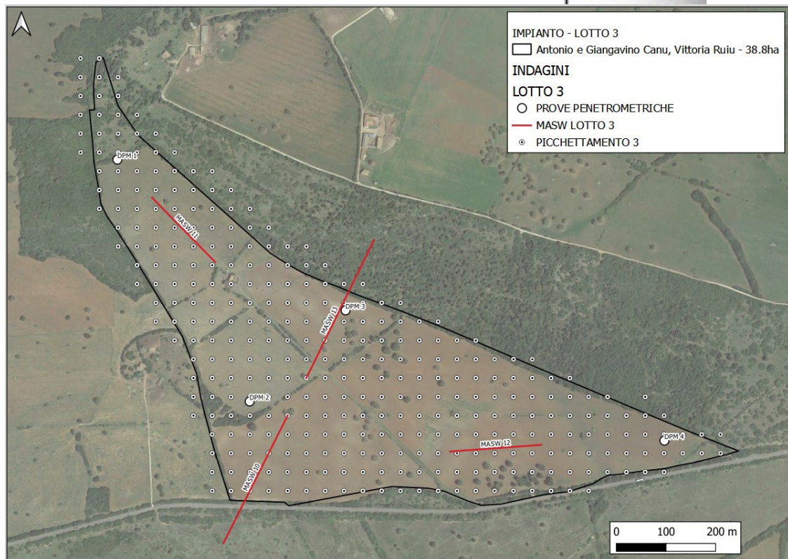
Figura 11: Ubicazione delle indagini geotecniche e geofisiche in sito - Aree impianto
