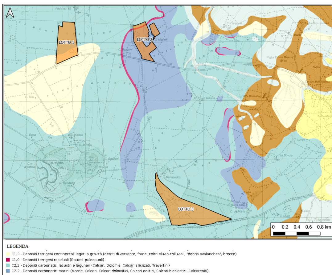
Figura 4: Carta Litologica di dettaglio redatta dalla Regione Autonoma della Sardegna. – Area impianto
