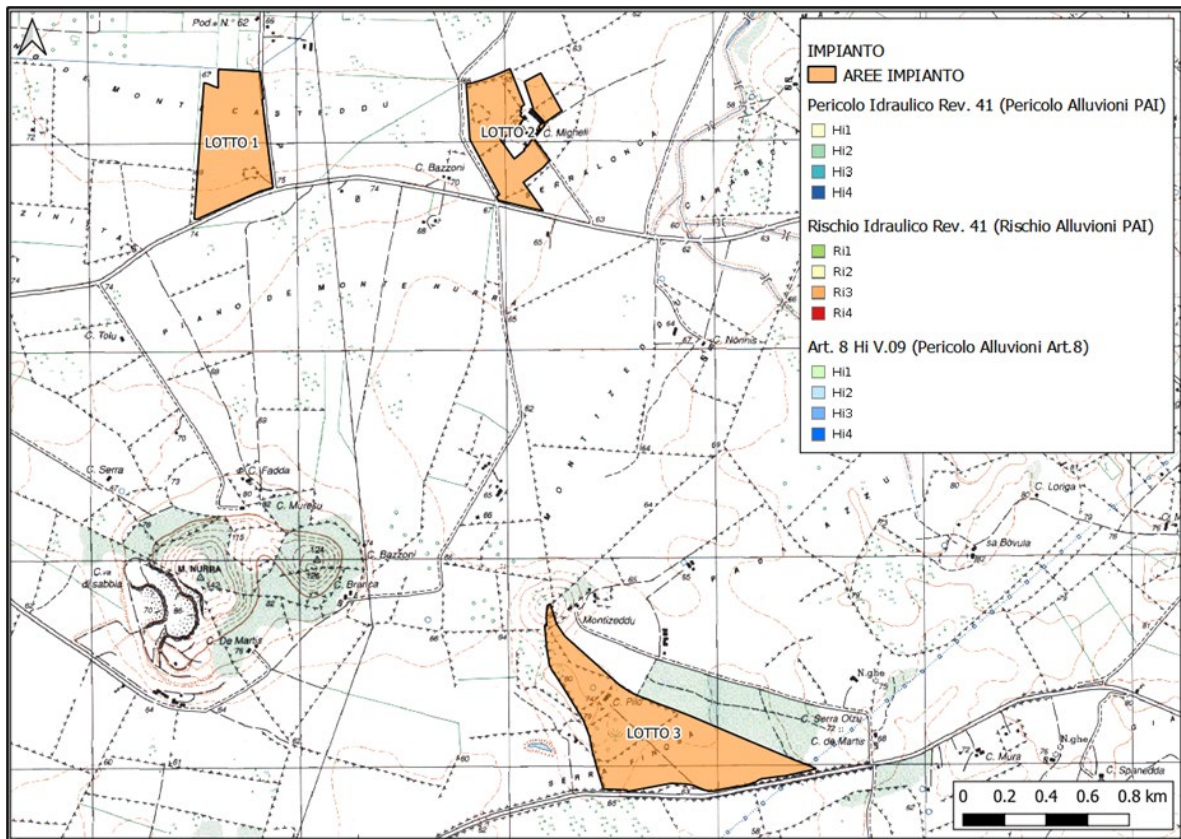
Fig. 4: Stralcio del P.A.I (Piano di Assetto Idrogeologico) RISCHIO e PERICOLOSITÀ DA ALLUVIONE secondo l'art. 41 redatto dalla Regione Autonoma della Sardegna
