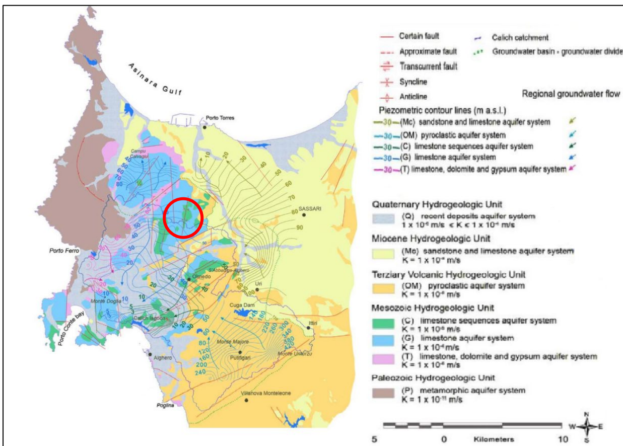
Figura 7: Mappa Idrogeologica e di Conducibilità Idraulica (K) (Ghiglieri et al., 2009) – In Verde (C), Azzurro (G) e Rosa (T) i Sistemi Acquiferi dell'Unità Idrogeologica Mesozoica
