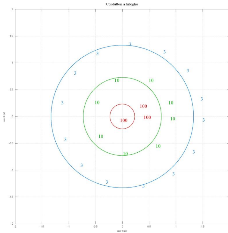
Isolinee – linea MT Altopiano-Su Campu (vista in sezione)
