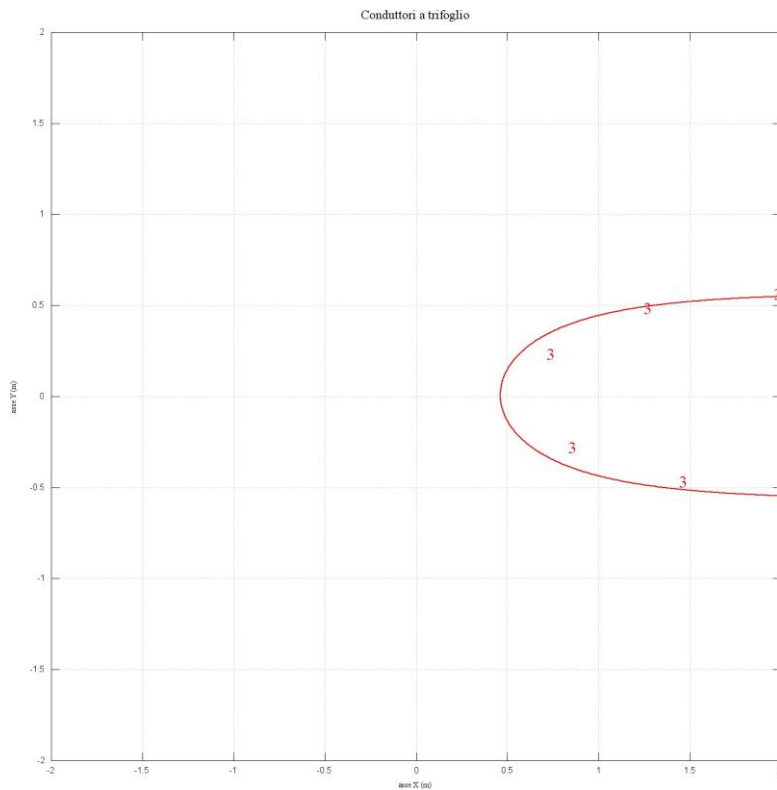
Isolinee – linea MT Altopiano-Su Campu (vista in pianta)
