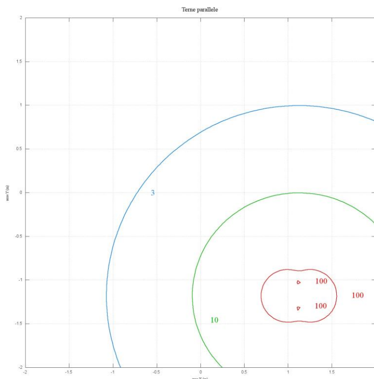
Isolinee – linea MT Su Campu – Stazione Elettrica Terna (vista in sezione)
