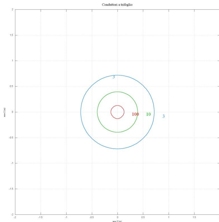
Isolinee - singola linea MT
