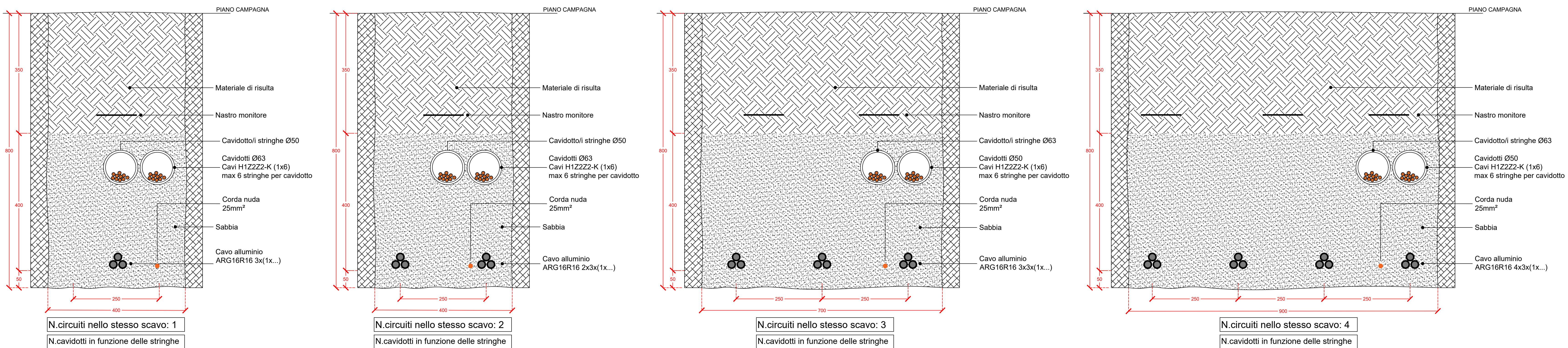
Collegamento BT inverter-trafo + stringa-inverter (sovrapposizione tracciato): sezione di scavo tipo
