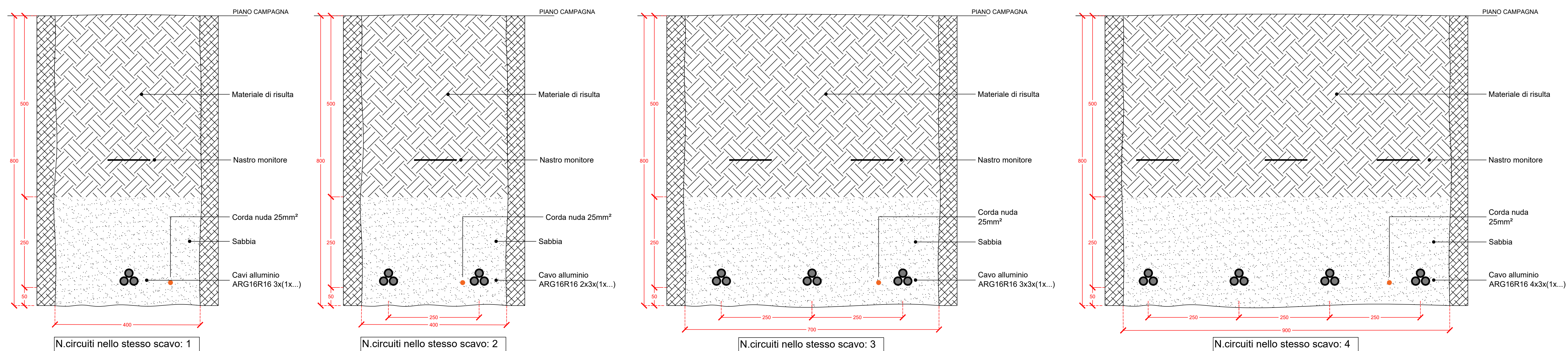
Collegamento BT stringa-inverter: sezione di scavo tipo
