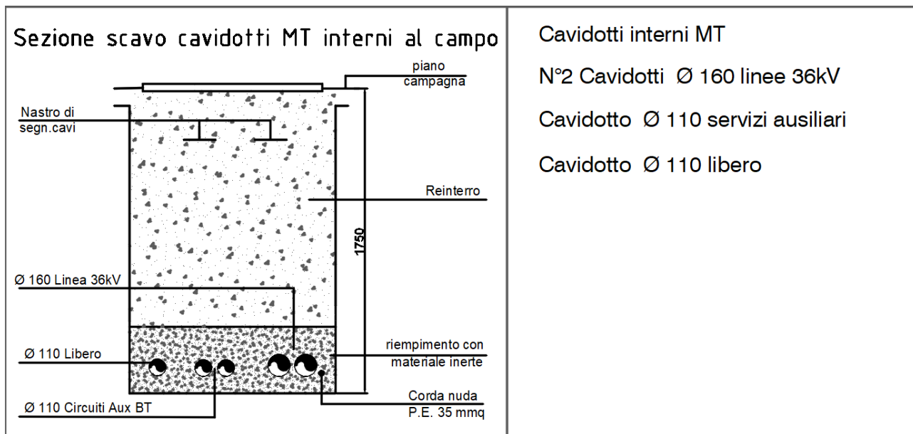
Tipologici scavi cavidotti di campo
