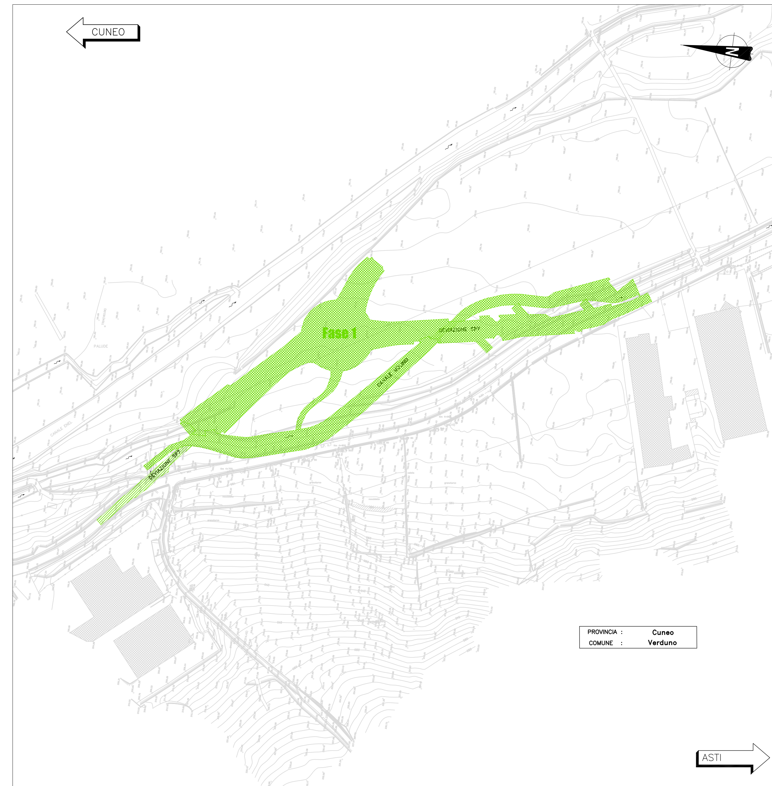
PLANIMETRIA CANTIERE IMBOCCO LATO ASTI – FASI DI REALIZZAZIONE FASE 1 scala 1:2000
