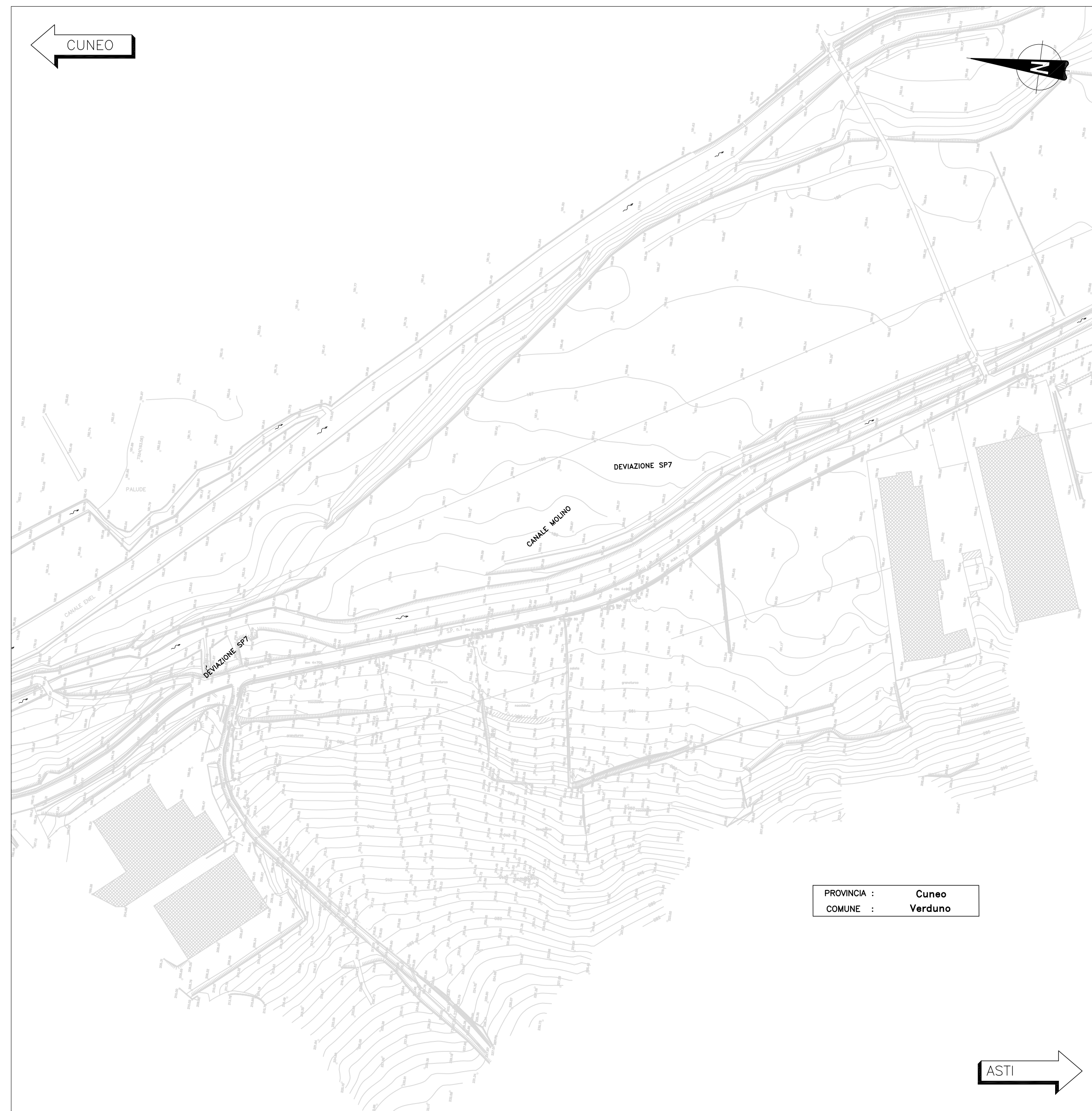
PLANIMETRIA CANTIERE IMBOCCO LATO ASTI – FASI DI REALIZZAZIONE STATO DI FATTO scala 1:2000
