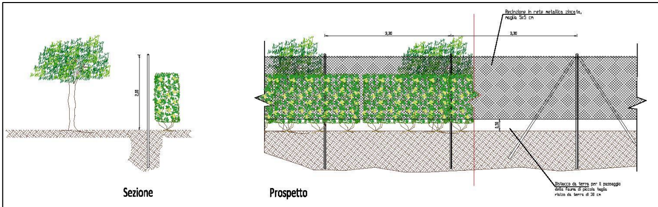
Figura 3 Particolare recinzione impianto agrovoltaico
