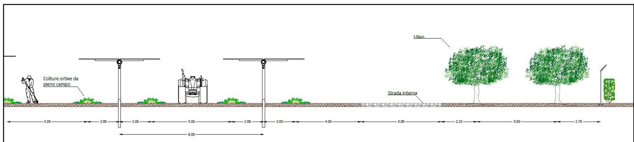
Figura 2|Sezione tipo tracker monoassiali e fascia di mitigazione
