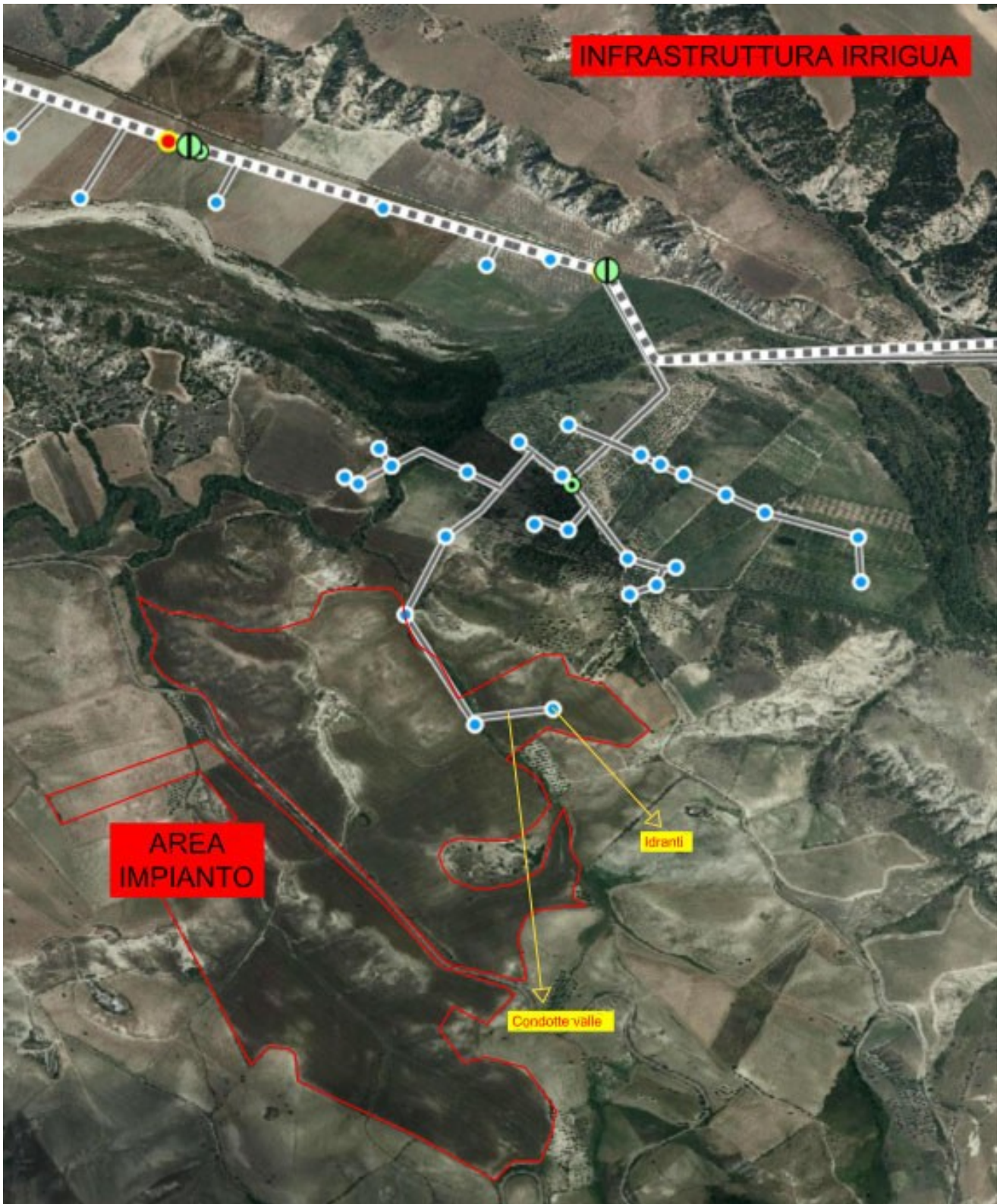
Figura n. 1 - Schema attuale rete irrigua consortile pubblica
