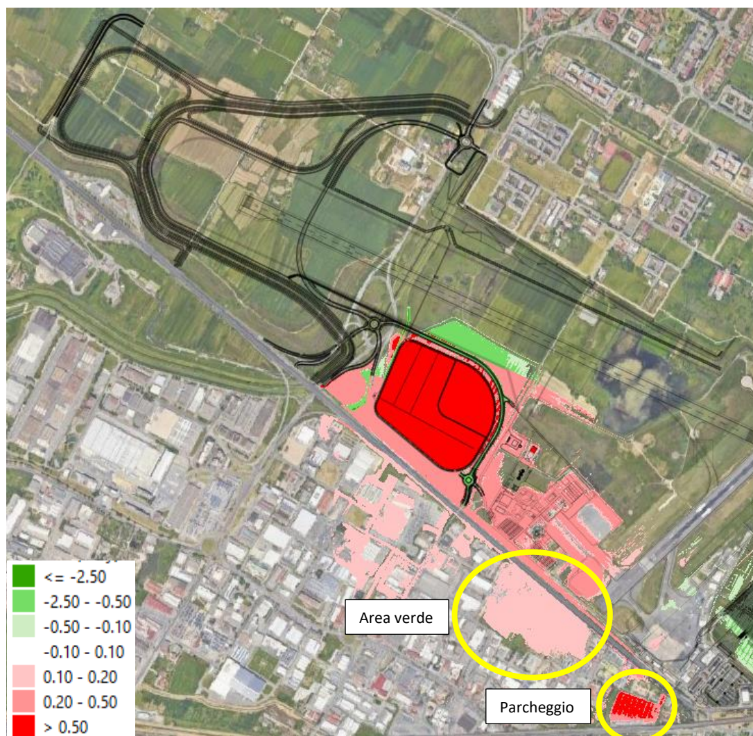
Figura 5-1: Differenza di battenti massimi per evento TR200 anni
