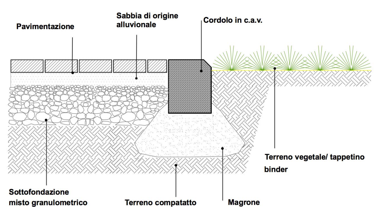
Particolare costruttivo - Sezione Area Parcheggio
