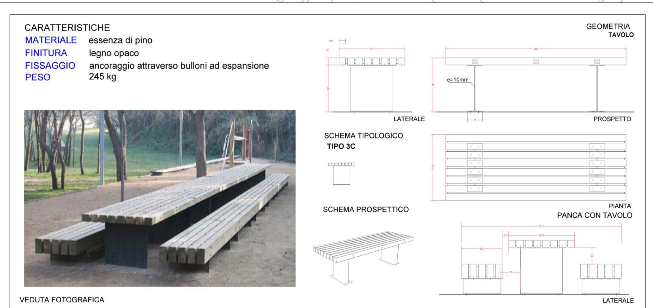
Particolare costruttivo - Tipologico sedute
