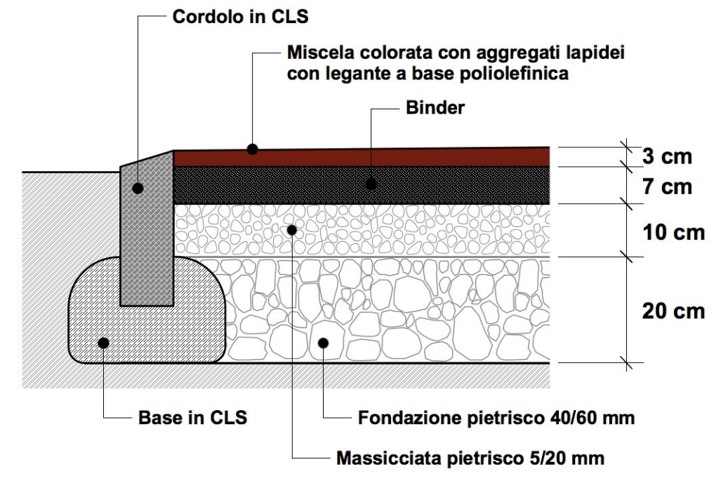
Particolare costruttivo - Sezione Pista ciclo-pedonale
