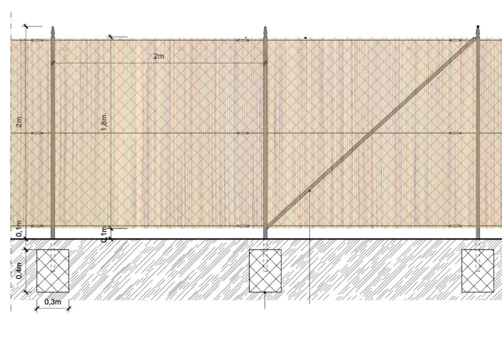
Particolare costruttivo - recinzione con schermatura
