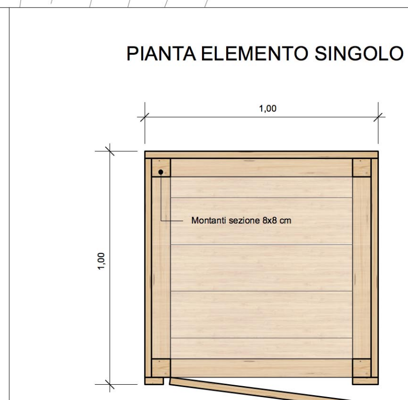
Particolare costruttivo - Contenitore multifunzione in legno
