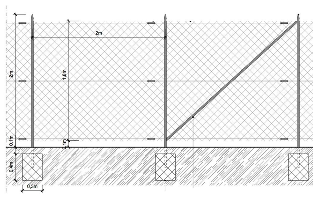
Particolare costruttivo - recinzione a maglia sciolta
