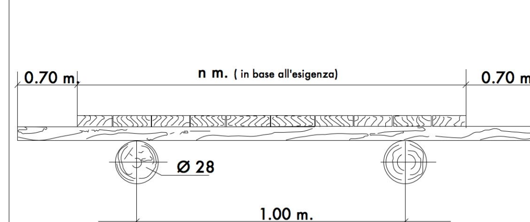
Particolare costruttivo - Sezione Ponte su fosso TIPO 2
