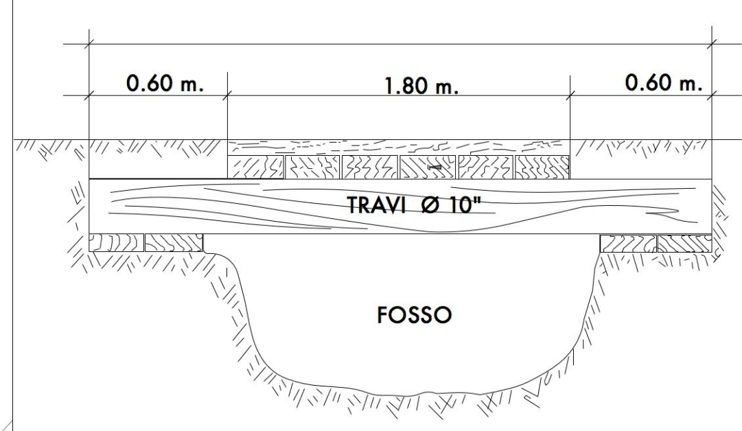
Particolare costruttivo - Sezione Ponte su fosso TIPO 1
