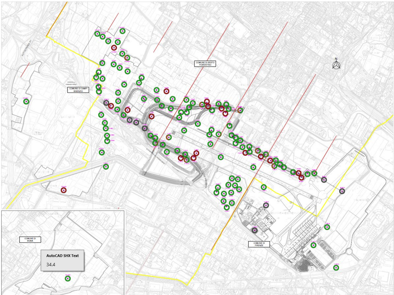
Figura 3-3 - Stralcio dell'elaborato grafico di progetto "Esiti dei saggi archeologici eseguiti", (rif. elab. FLR-MPL-PSA-ARG1-003-AL-PL_Esiti Saggi Arceo)
