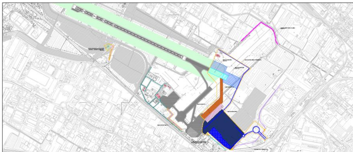
Figura 11 Fase di cantierizzazione C2
