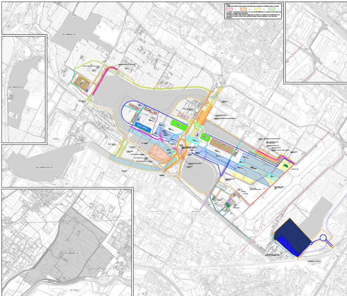
Figura 9. Fase di cantierizzazione B3
