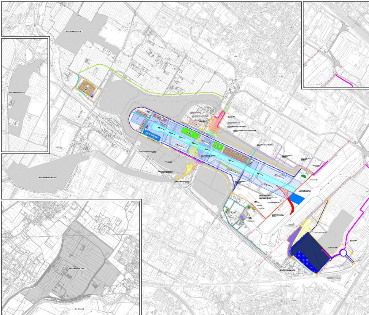
Figura 10 Fase di cantierizzazione C1
