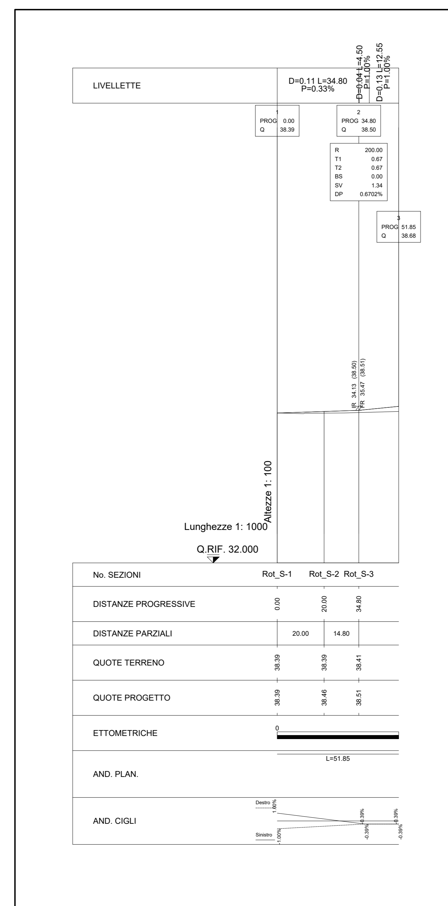
PROFILO LONGITUDINALE "SUD" 1:1000/100
