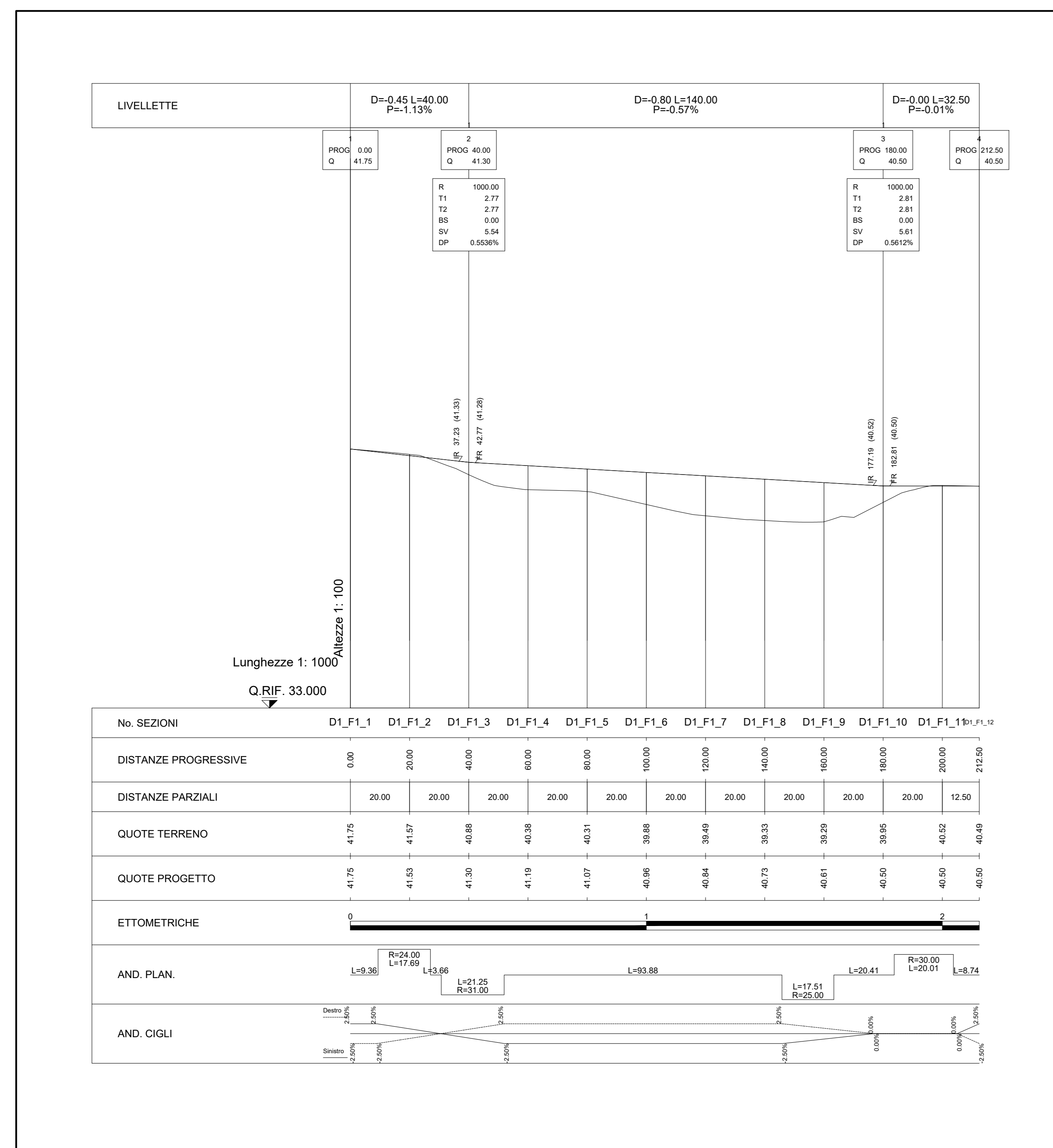
PROFILO LONGITUDINALE "D1_F1" 1:1000/100
