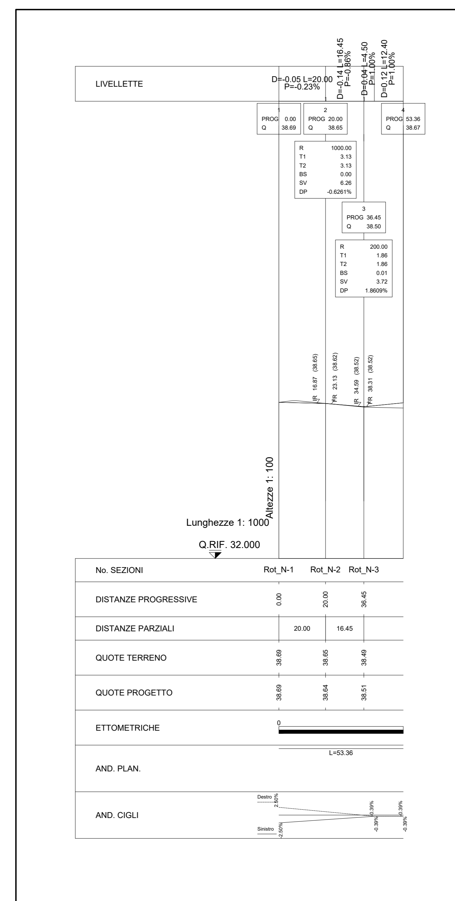
PROFILO LONGITUDINALE "NORD" 1:1000/100
