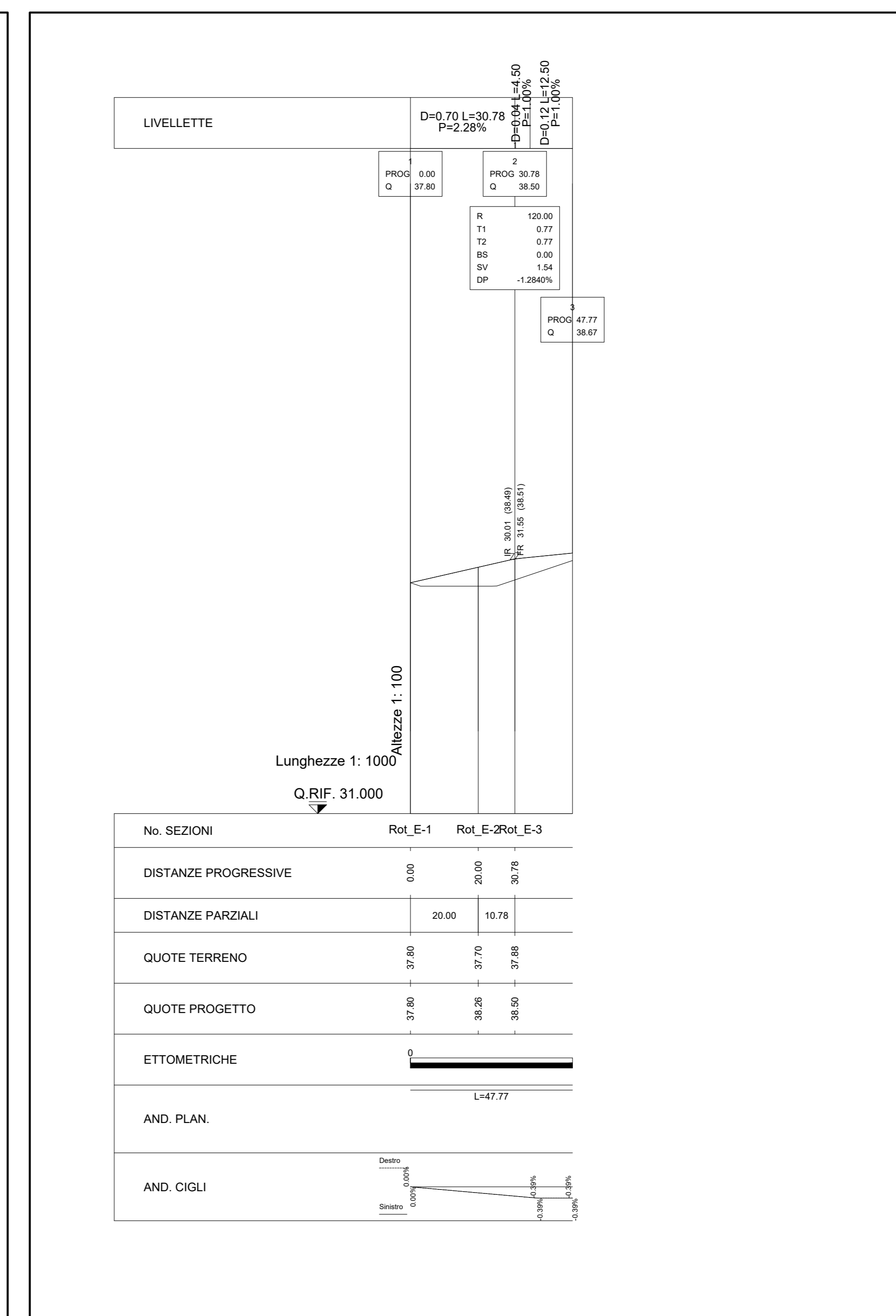
PROFILO LONGITUDINALE "EST" 1:1000/100
