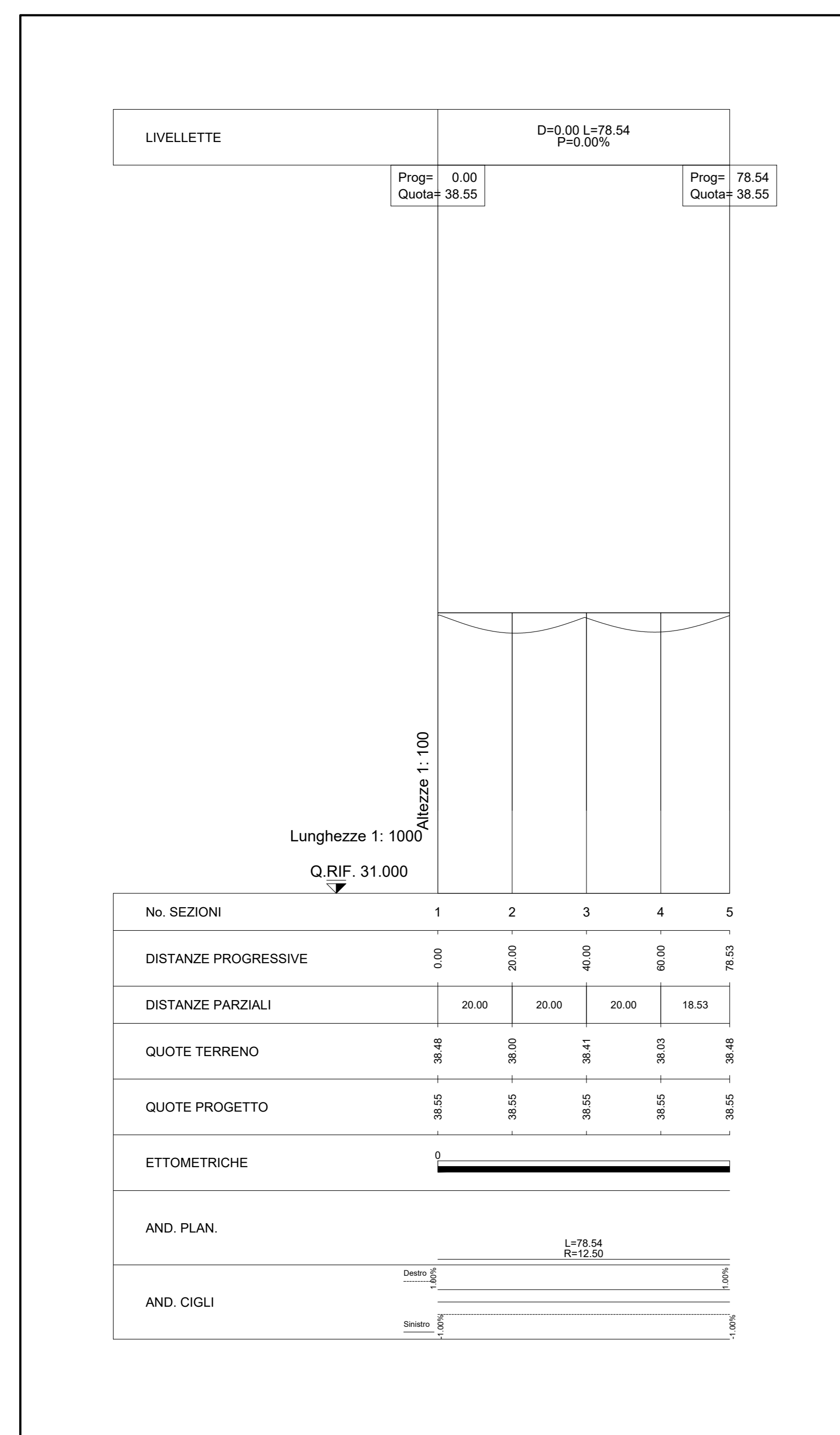
PROFILO LONGITUDINALE "ANELLO" 1:1000/100
