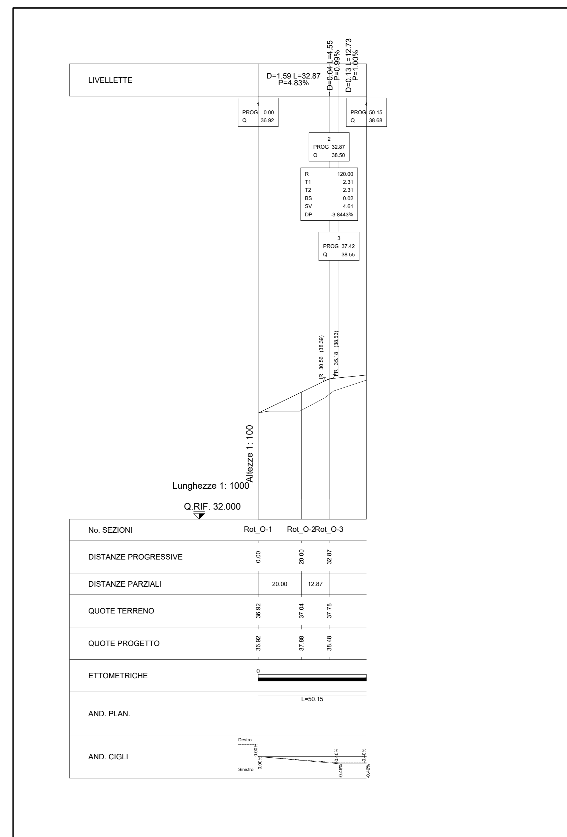
PROFILO LONGITUDINALE "OVEST" 1:1000/100
