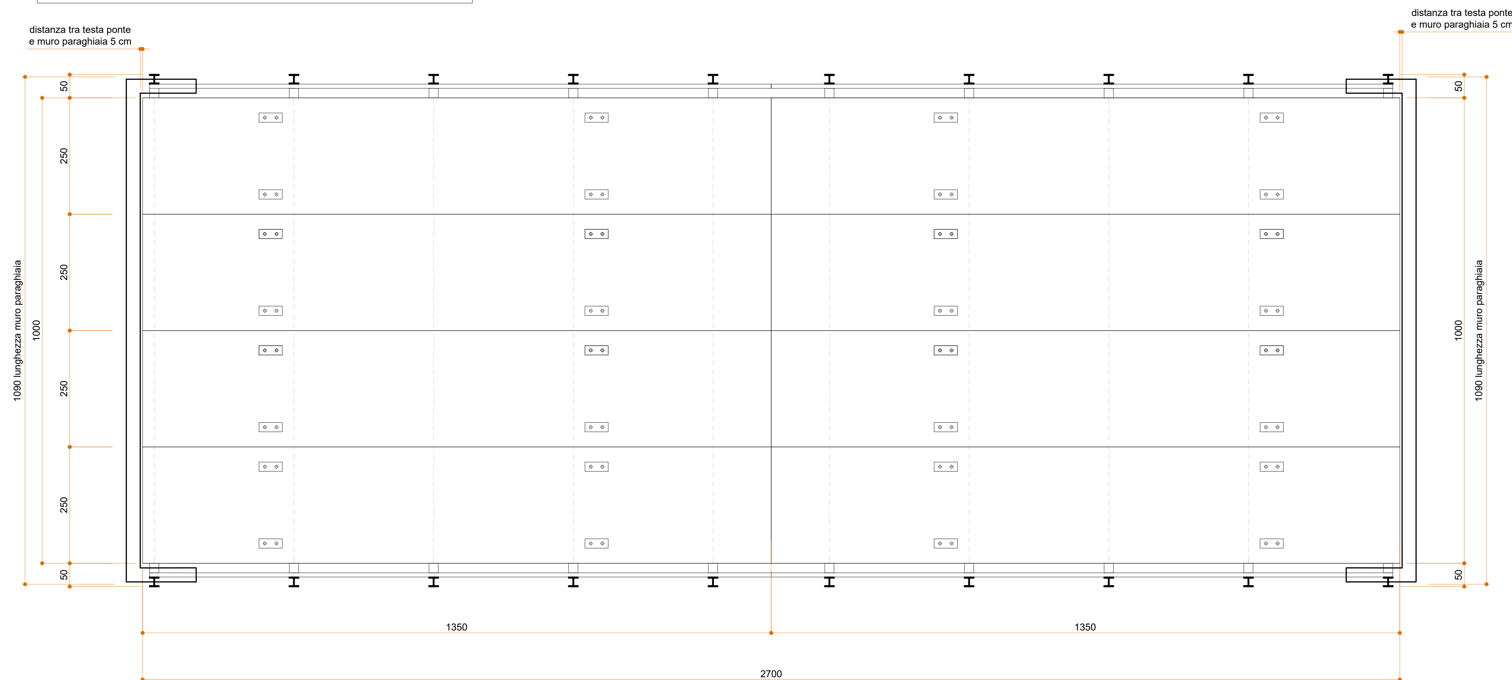
PIANTA STRUTTURE IMPALCATO - scala 1:50
