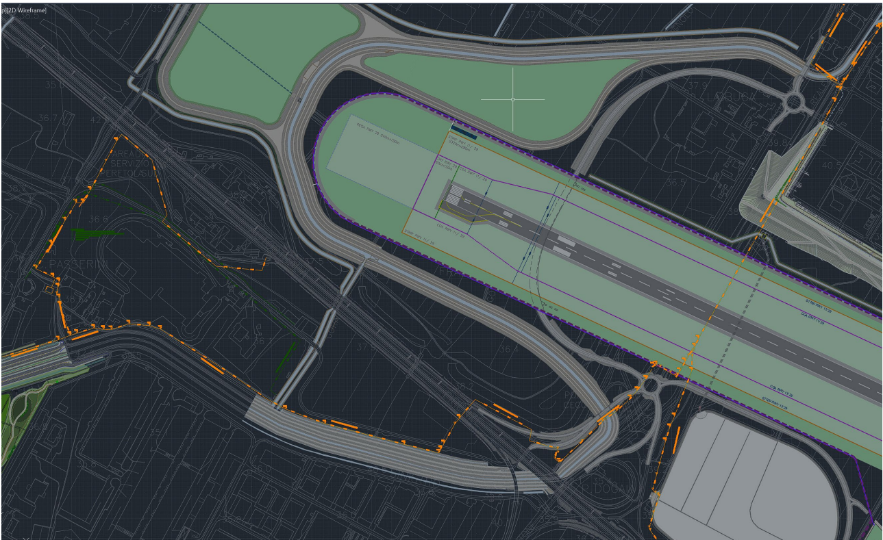
Figura 5 Sovrapposto masterplan – rete Snam
