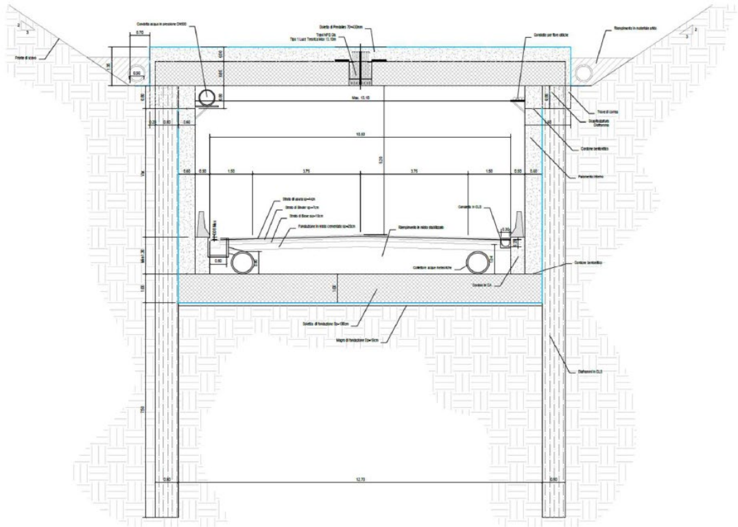
Figura 2 Sezione del sottoattraversamento e riprotezione sottoservizi
