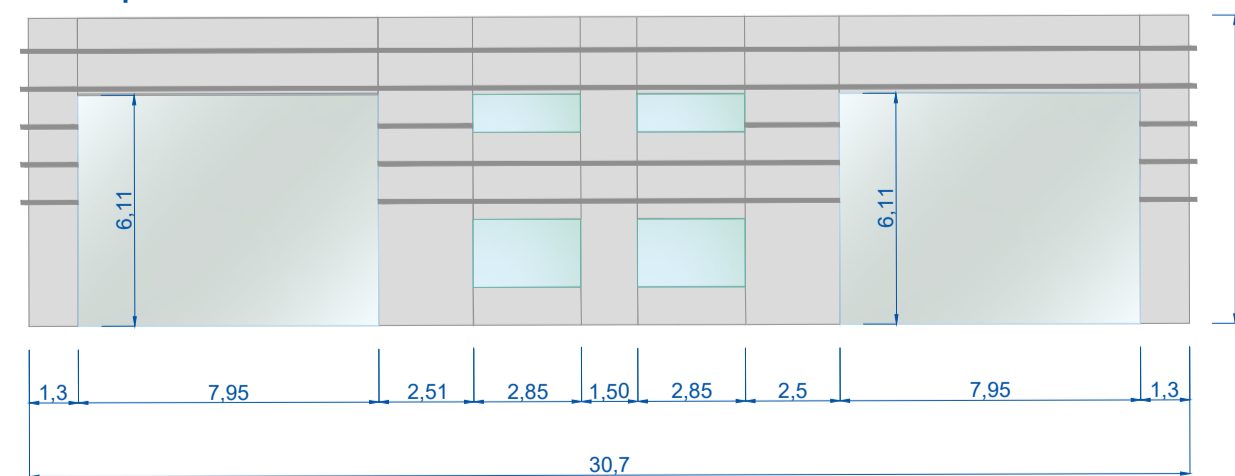
Prospetto Sud-Ovest - C - C08
