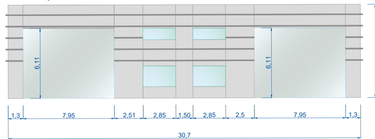
Prospetto Nord Est - A - C08
