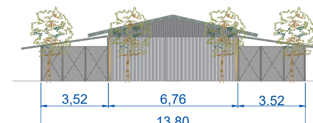
Prospetto Ovest - D - C13 Canile
