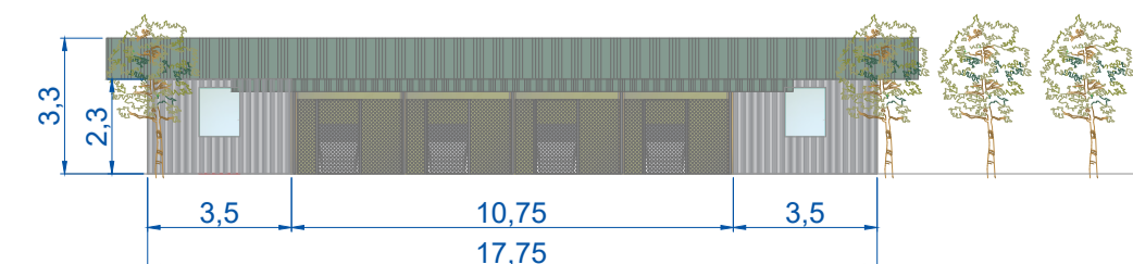
Prospetto Sud - C - C13 Canile
